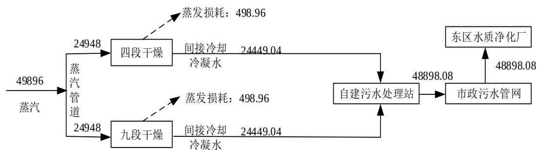
图 2-5 本项目蒸汽平衡图 (单位: t/a)
