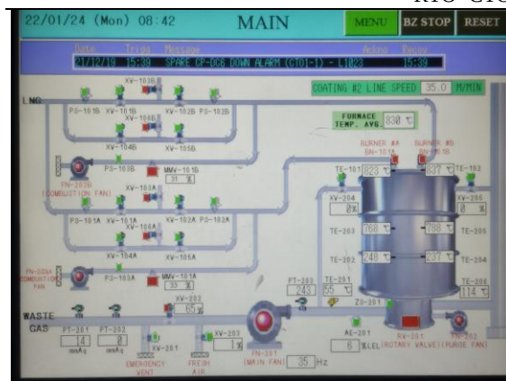
RTO+CTO实时运行图
