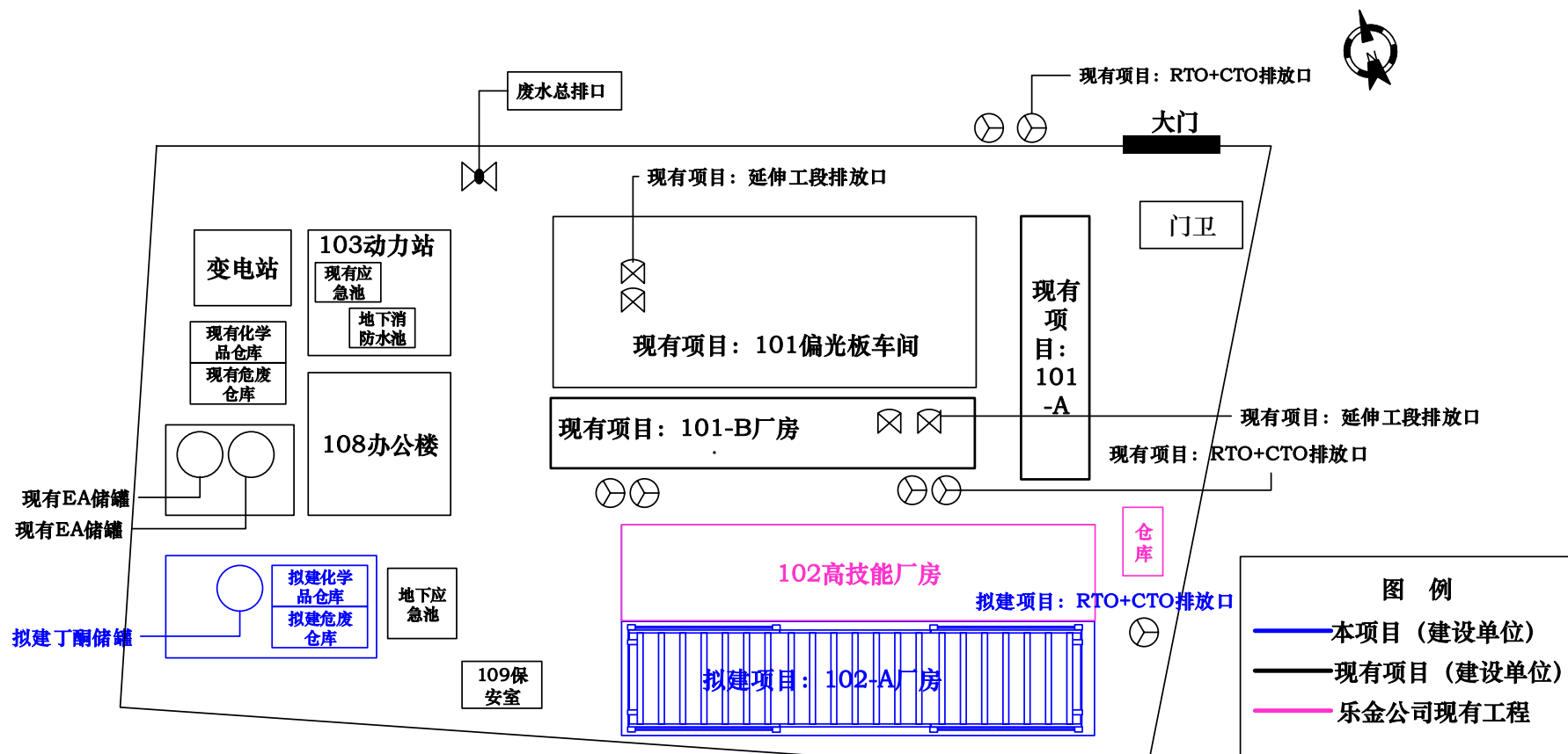
附图 3-① 项目总平面布置图
