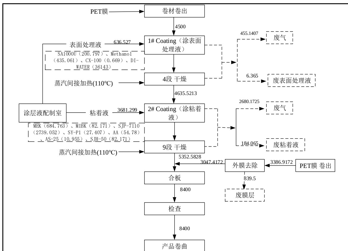
图 2-4 本项目物料平衡图 (单位: t/a)
