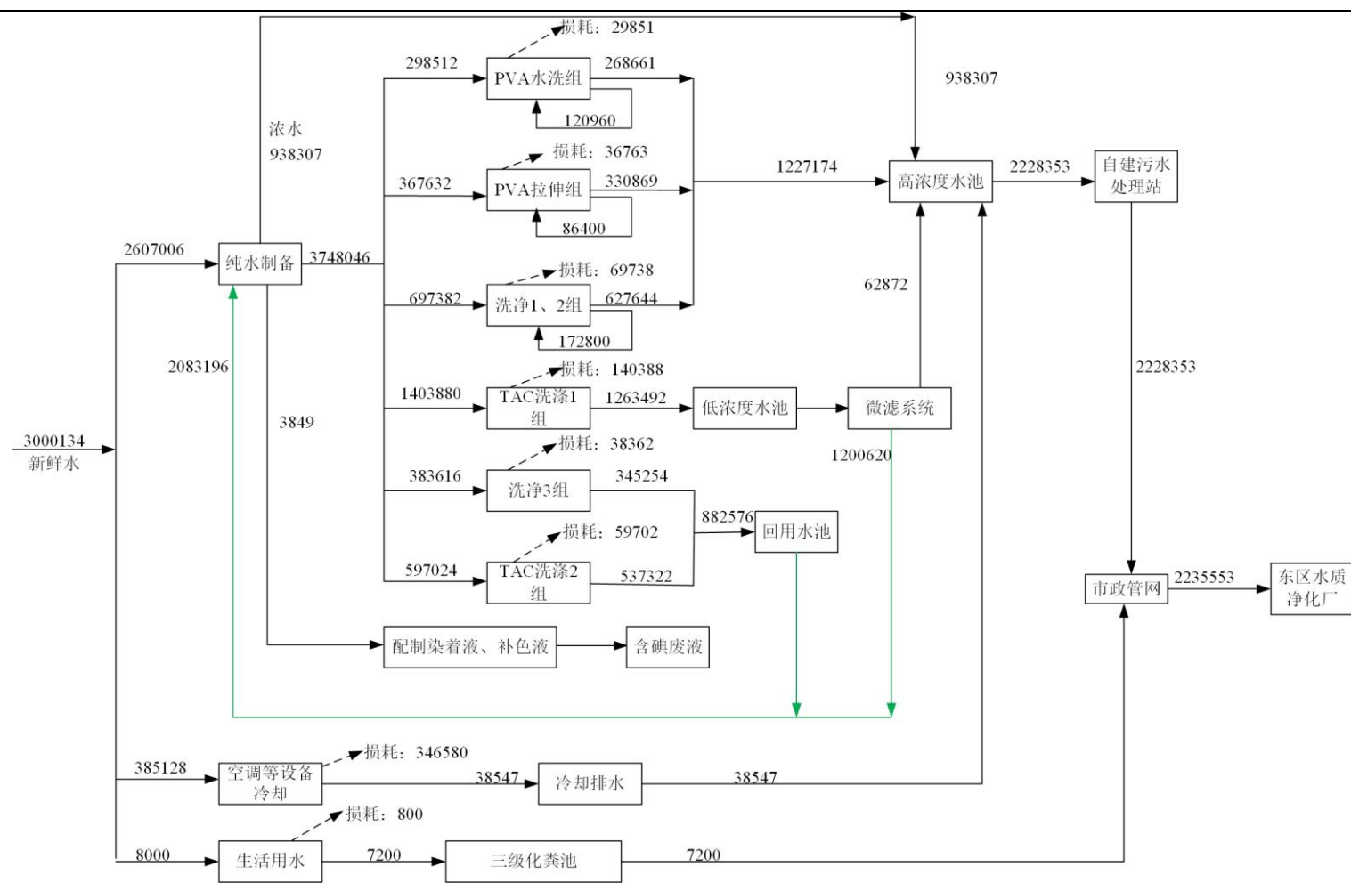
图 2-2 现有项目水平衡图（单位：t/a）
