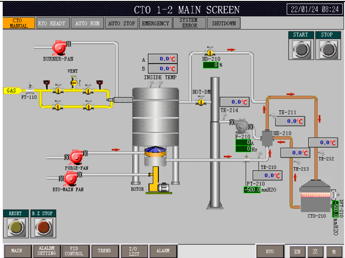
RTO+CTO实时运行图
