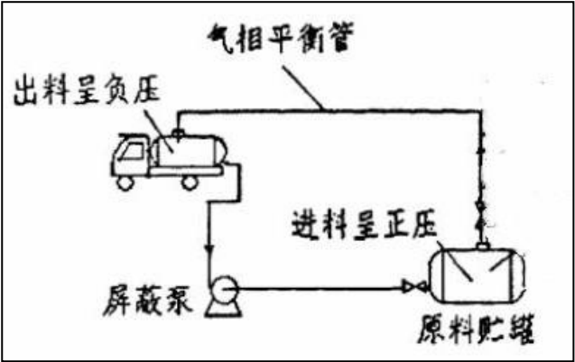
图 4-1 气相平衡管原理图
