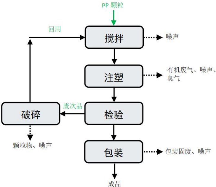
图2-3 塑料衣架生产工艺流程图
