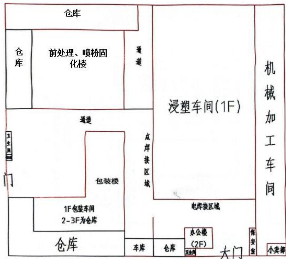
附图 17 原项目车间布局图
