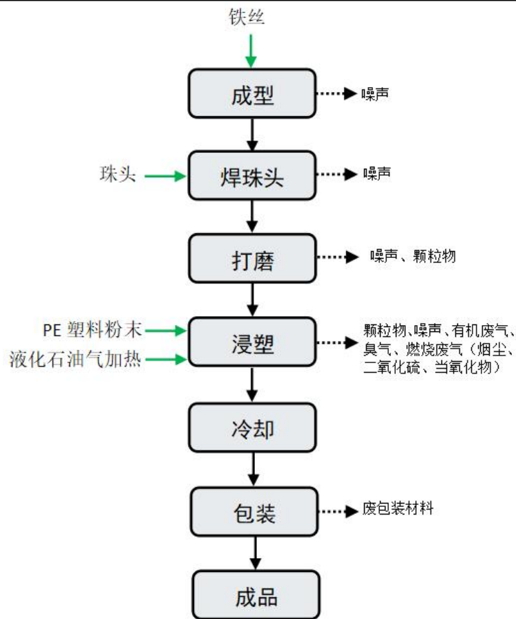
图2-2 金属衣架生产工艺流程图
