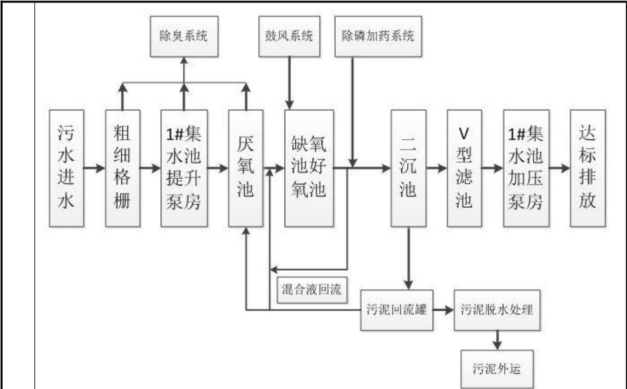
图 4-2 永和污水处理厂一、二期污水处理工艺流程图
