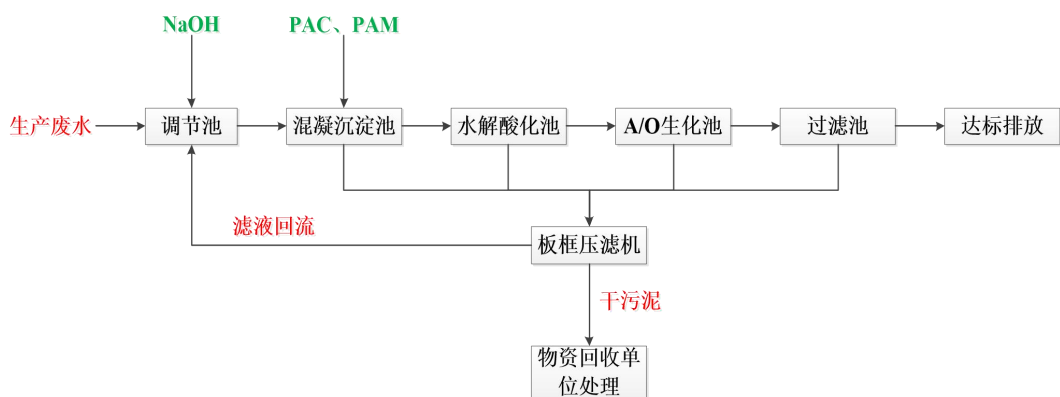
图 4-1 本项目自建污水处理设施工艺流程图例
