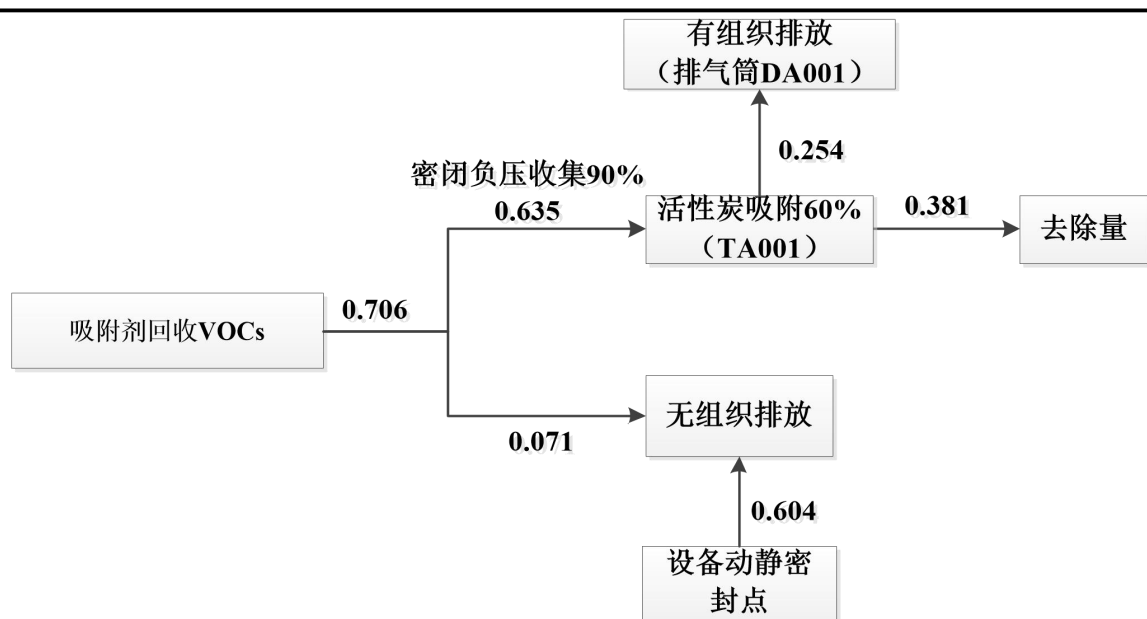
图2-2 本项目有机废气平衡图（单位t/a）
