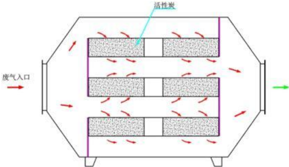
图 4-4 本项目活性炭箱设计图
