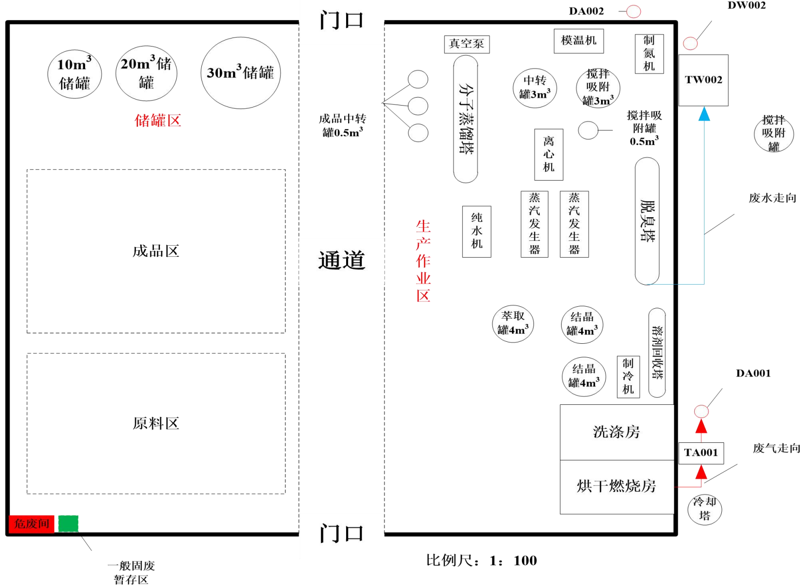
附图 4 建设目总平面布图
