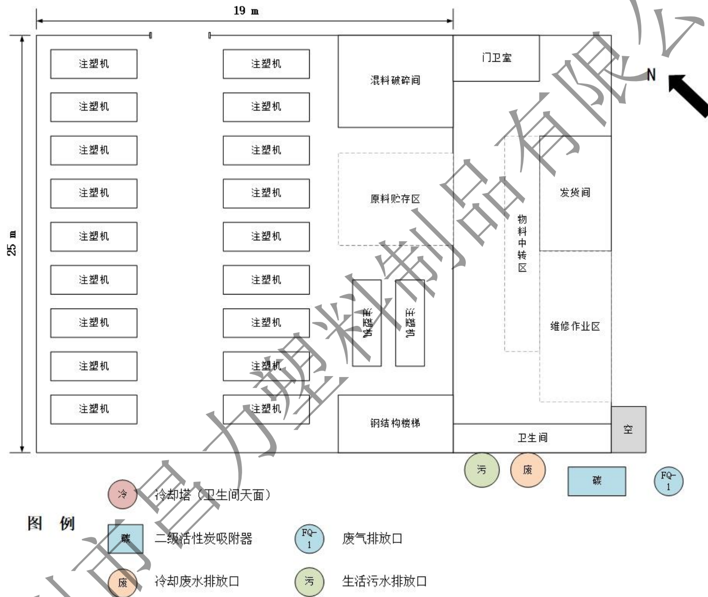
附图 3-1 平面布置图—地面层及外部
