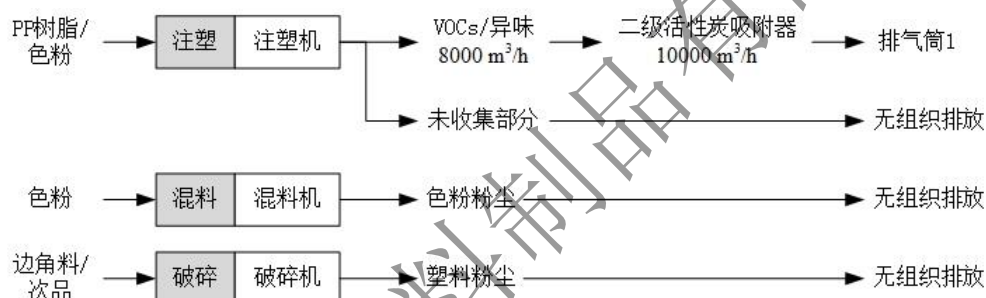
图 4-2 废气收集、治理和排放汇总示意图
