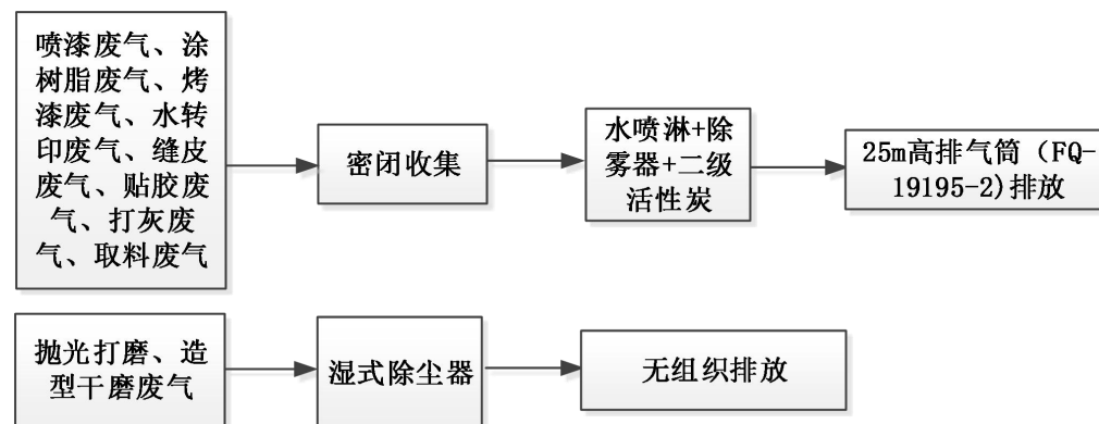
图 4-1 废气治理工艺流程图
