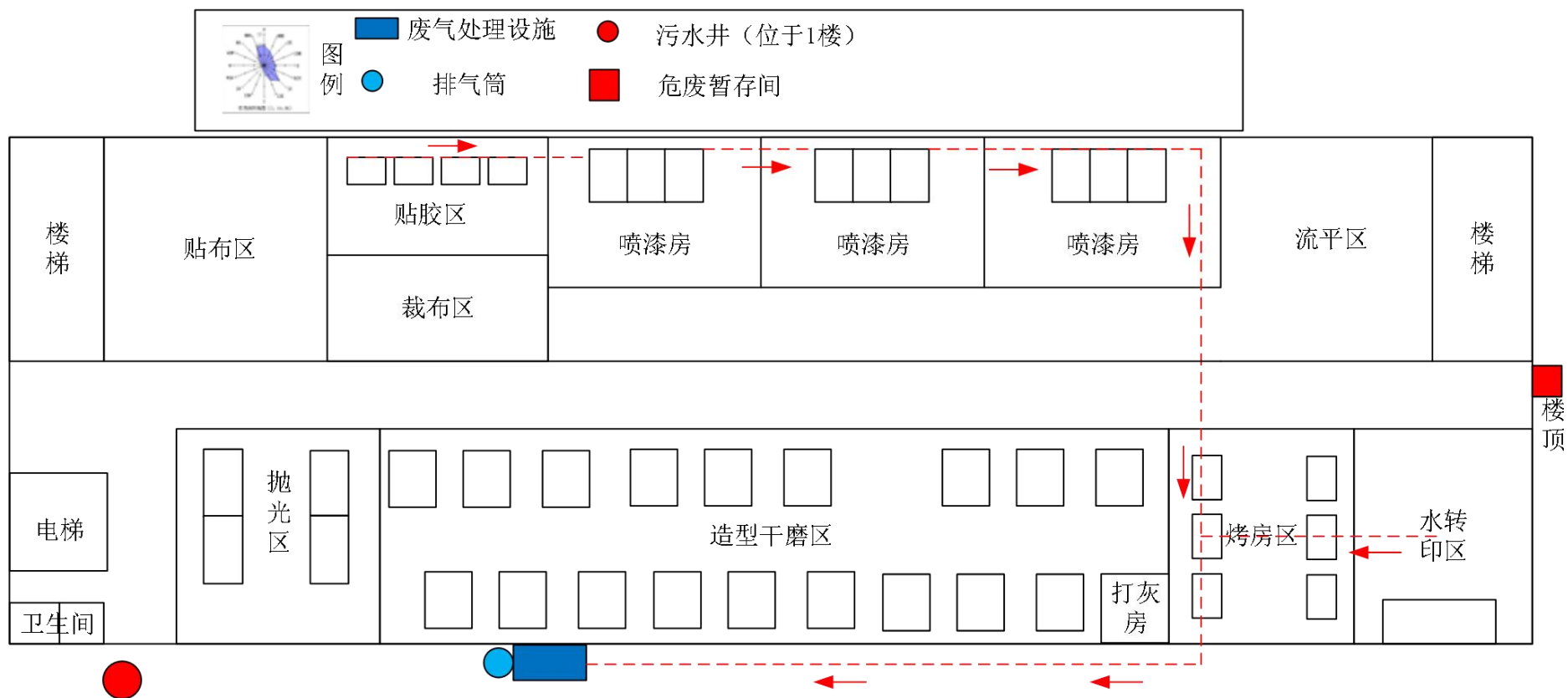
附图4-3 项目平面布局图四楼（扩建后全厂）
