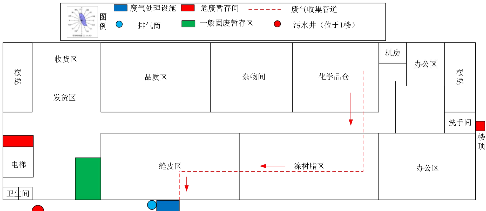
附图4-2 扩建项目平面布局图三楼（扩建后全厂）
