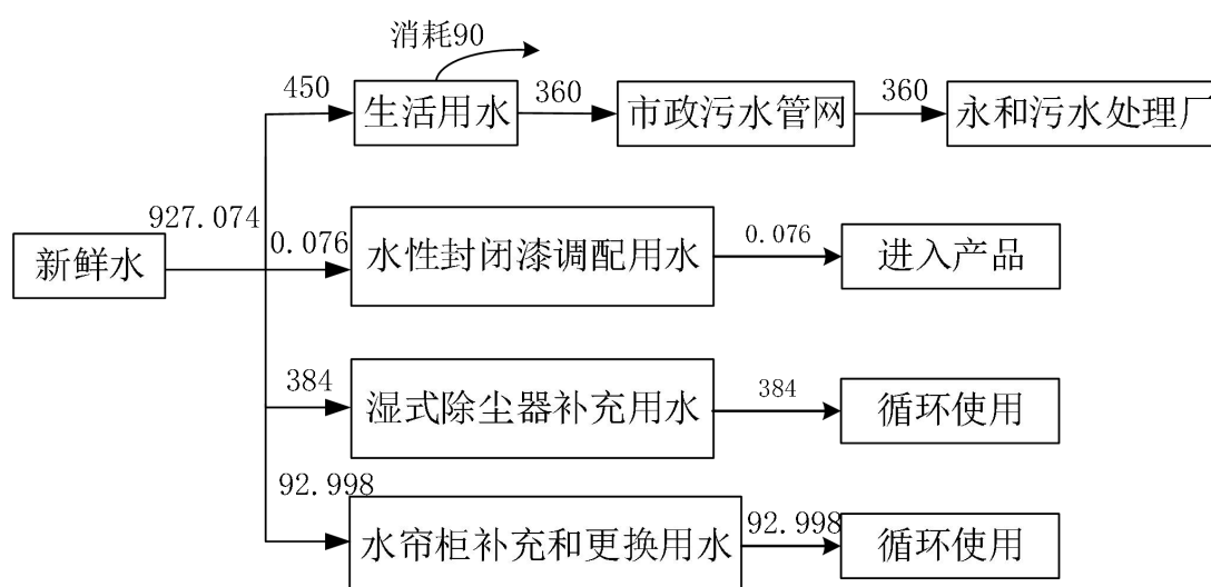
图2-1 本扩建项目水平衡图（单位：t/a）
