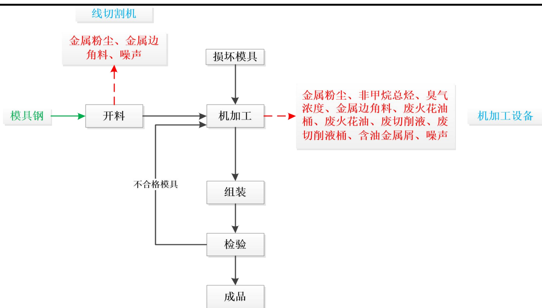
图 2-4 本项目模具制造、维修工艺流程及产污环节图
