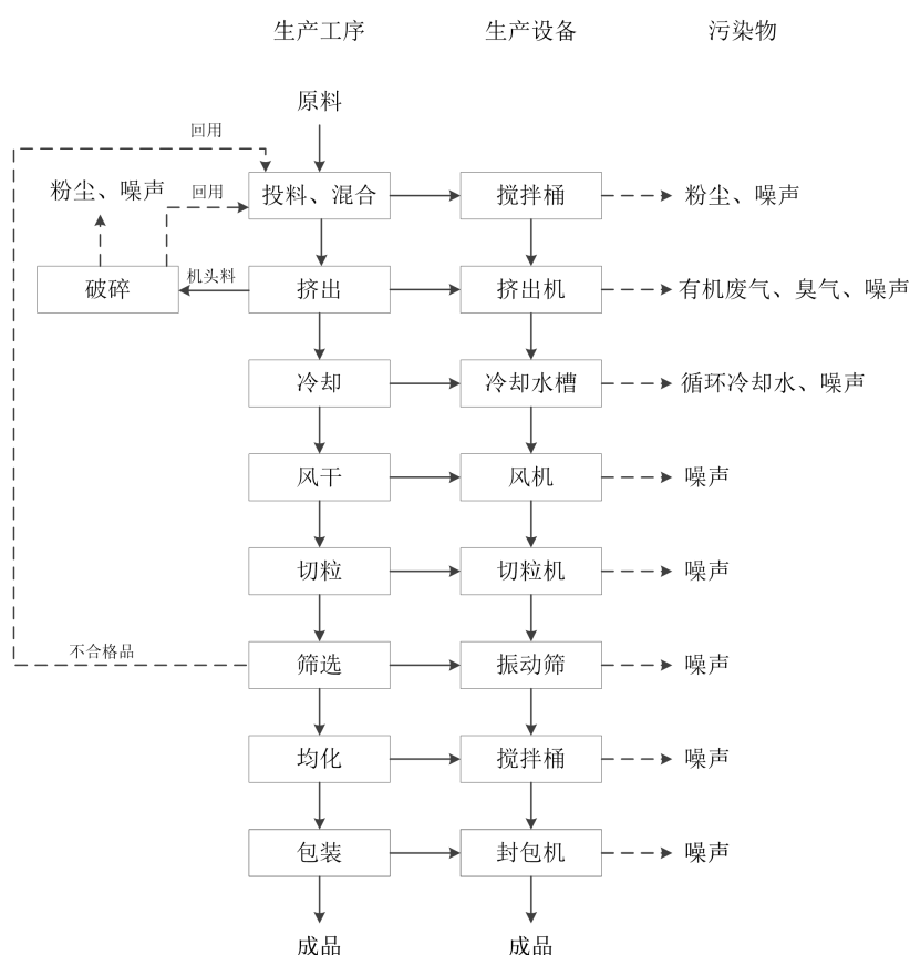
图 2-2 改性塑料生产工艺流程及产污环节图
