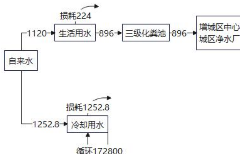
图 2-1 水平衡图 单位：m³/a
