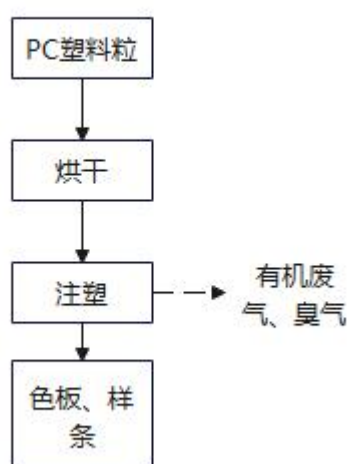
图 2-3 色板和样条注塑工艺流程及产污环节图
