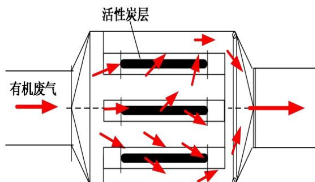
图 4-2 本项目活性炭箱设计图
