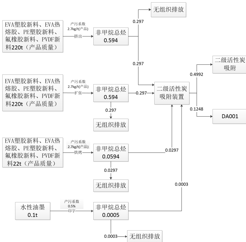
图 2-2 本项目有机废气平衡图 (单位 t/a)
