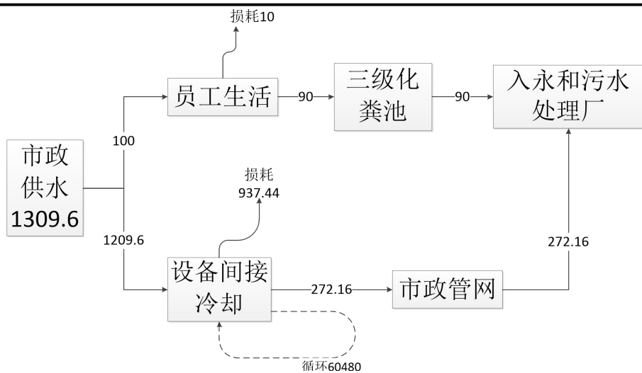
图 2-1 本项目水平衡图 (单位 m³/a)
