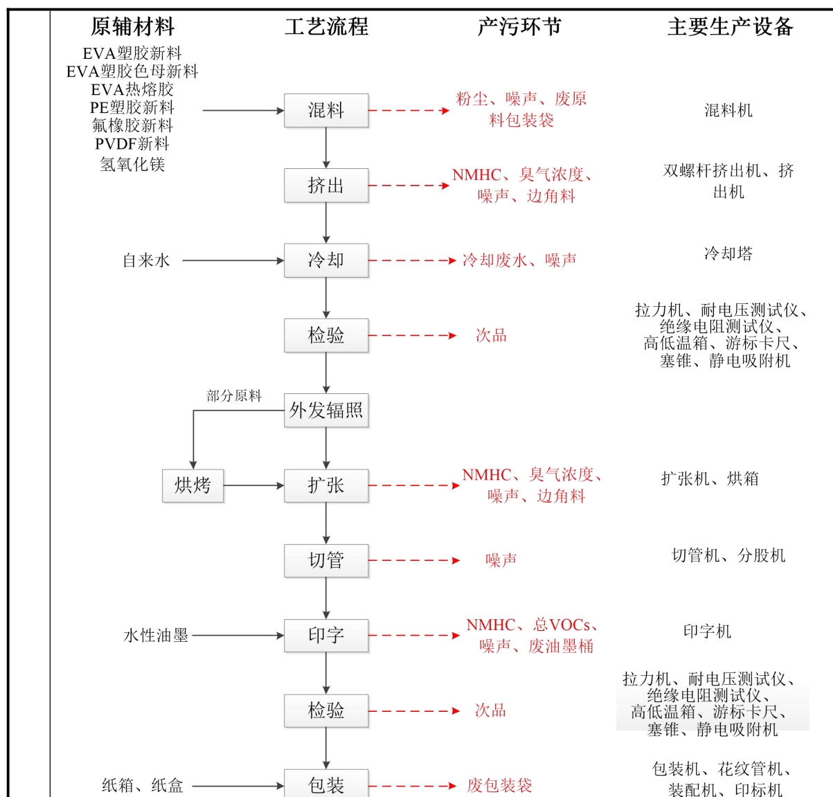
图 2-3 本项目生产工艺流程及产污环节图
