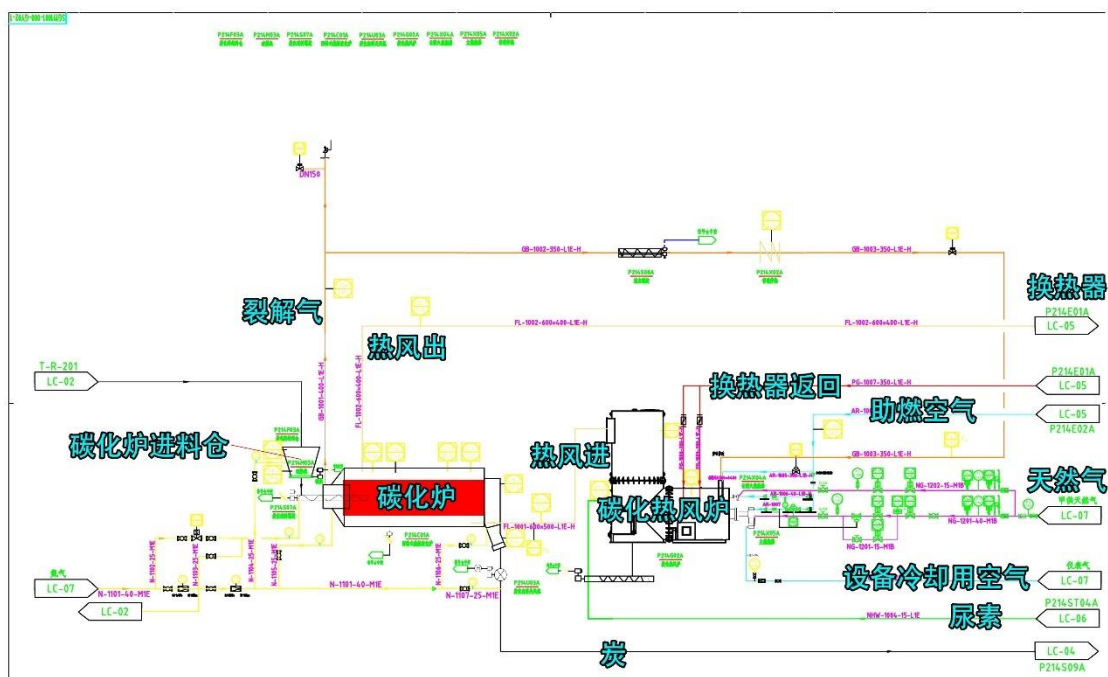
图 2-3 碳化单元设备连接图
