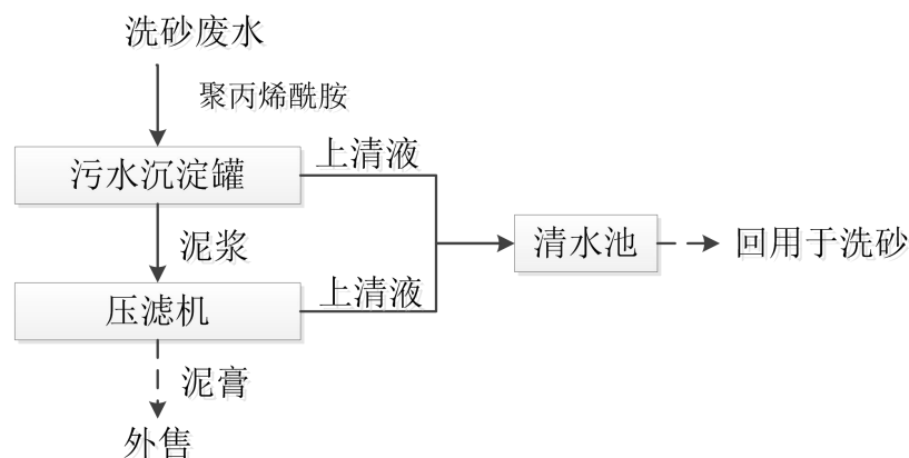
图 4-1 本项目泥浆水处理工艺流程图
