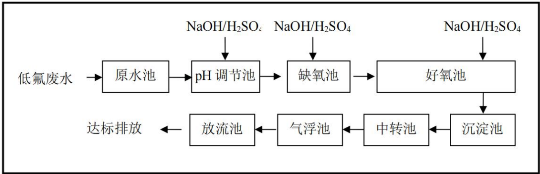
图 4-1 华星光电 t9 项目低氟有机废水处理系统废水处理工艺
