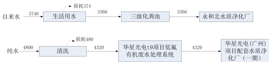
图 2-1 本项目水平衡图 (m³/a)
