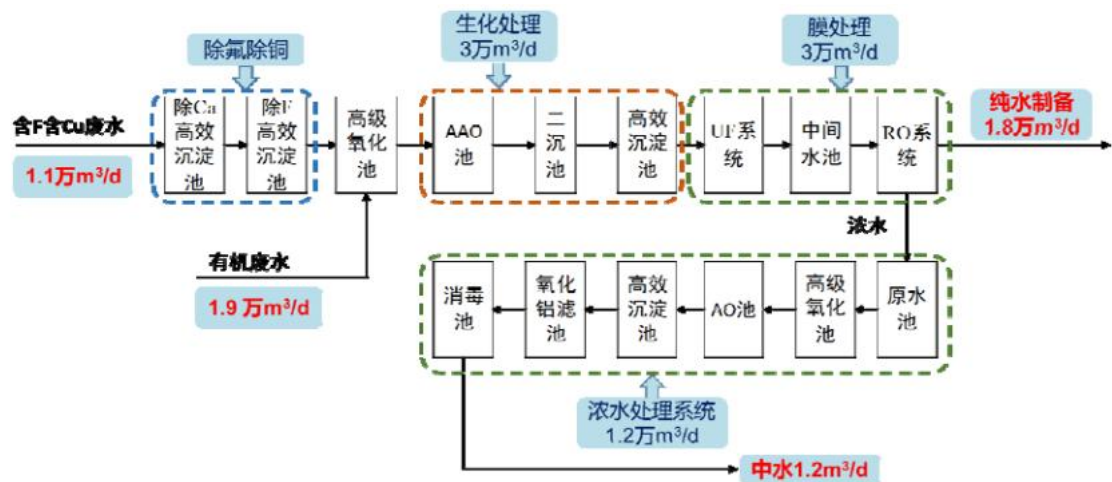
图 4-2 华星光电（广州）项目配套水质净化厂工程（一期）工艺流程图
