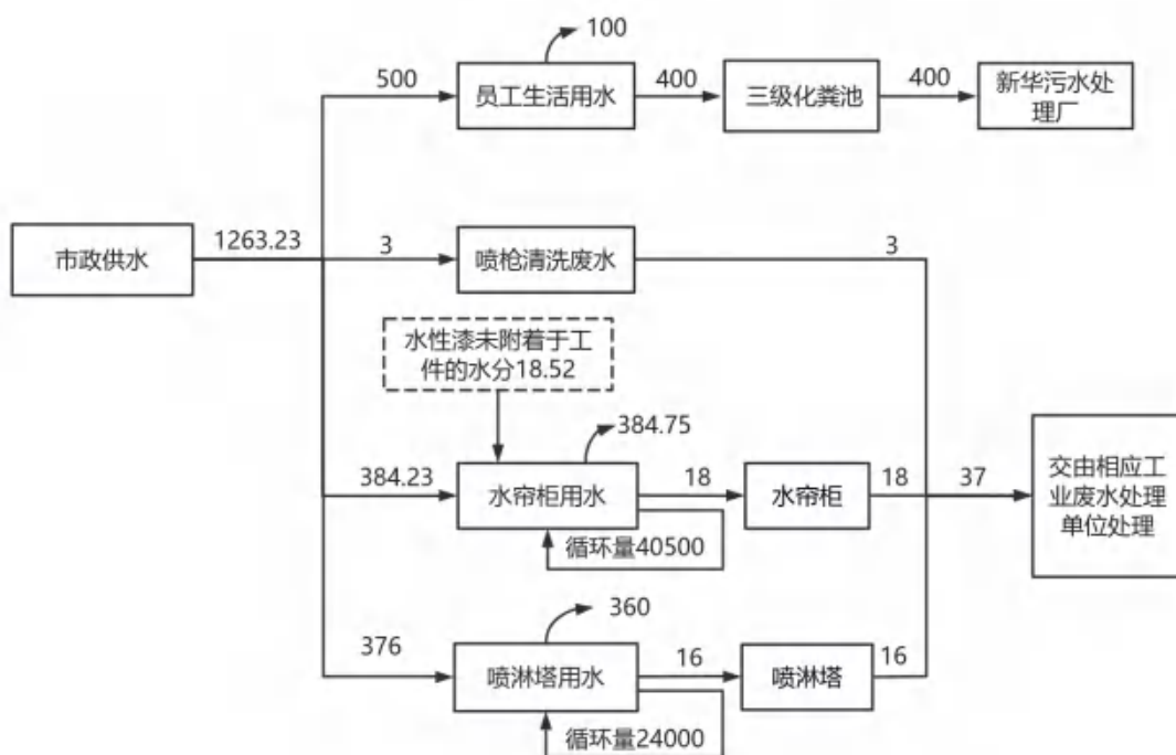
图2-1 本项目水平衡图 (单位 \text{m}^3/\text{a} )
