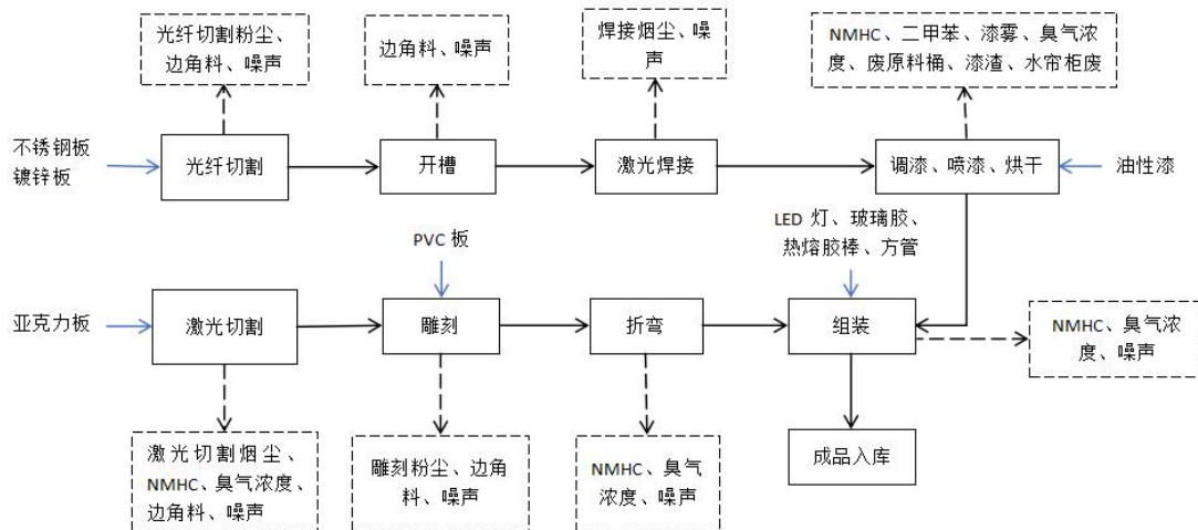
图 2-4 发光字生产工艺流程图
