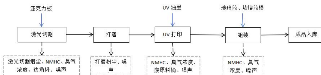
图 2-5 亚克力制品生产工艺流程图
