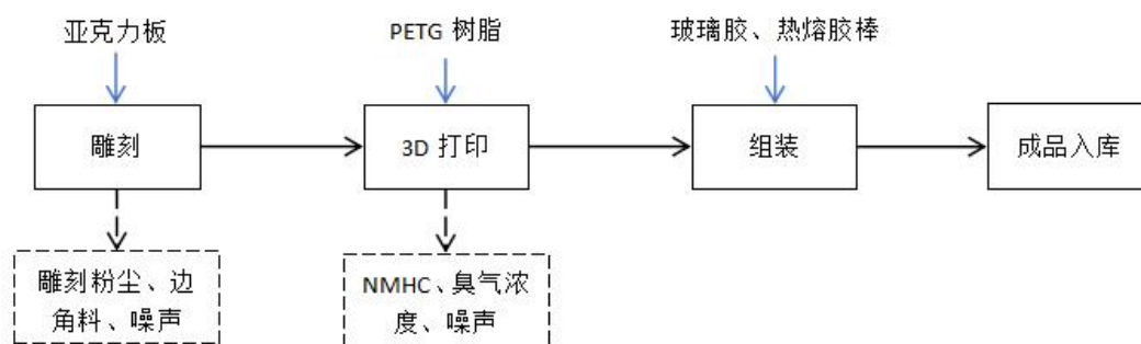
图 2-6 3D 打印字工艺流程图
