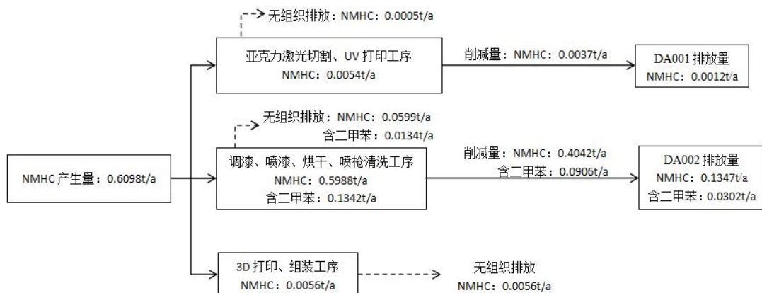
图 2-2 有机废气（NMHC、二甲苯）平衡图
