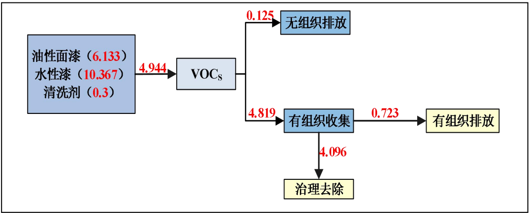
图 2-2 本次改扩建项目涂装 1#线 VOCs 物料平衡图 (单位: t/a)
