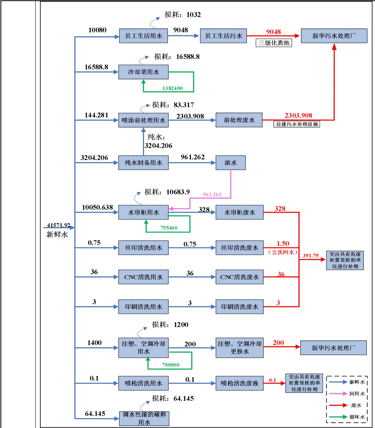
图 2-6 总体项目水平衡图 (t/a)
