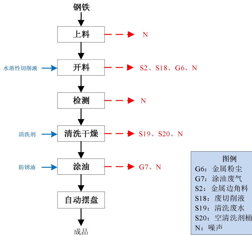
图 2-9 铁环工艺流程图
