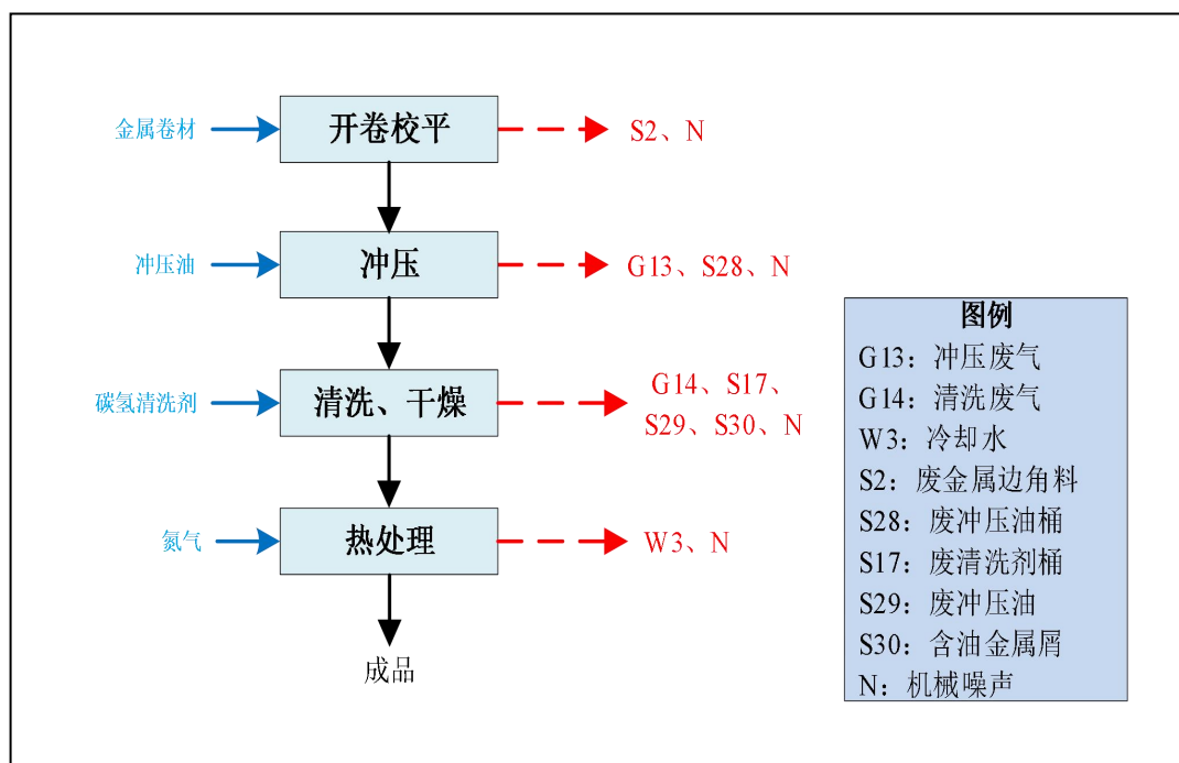
图 2-11 stator（定子）生产工艺流程图
