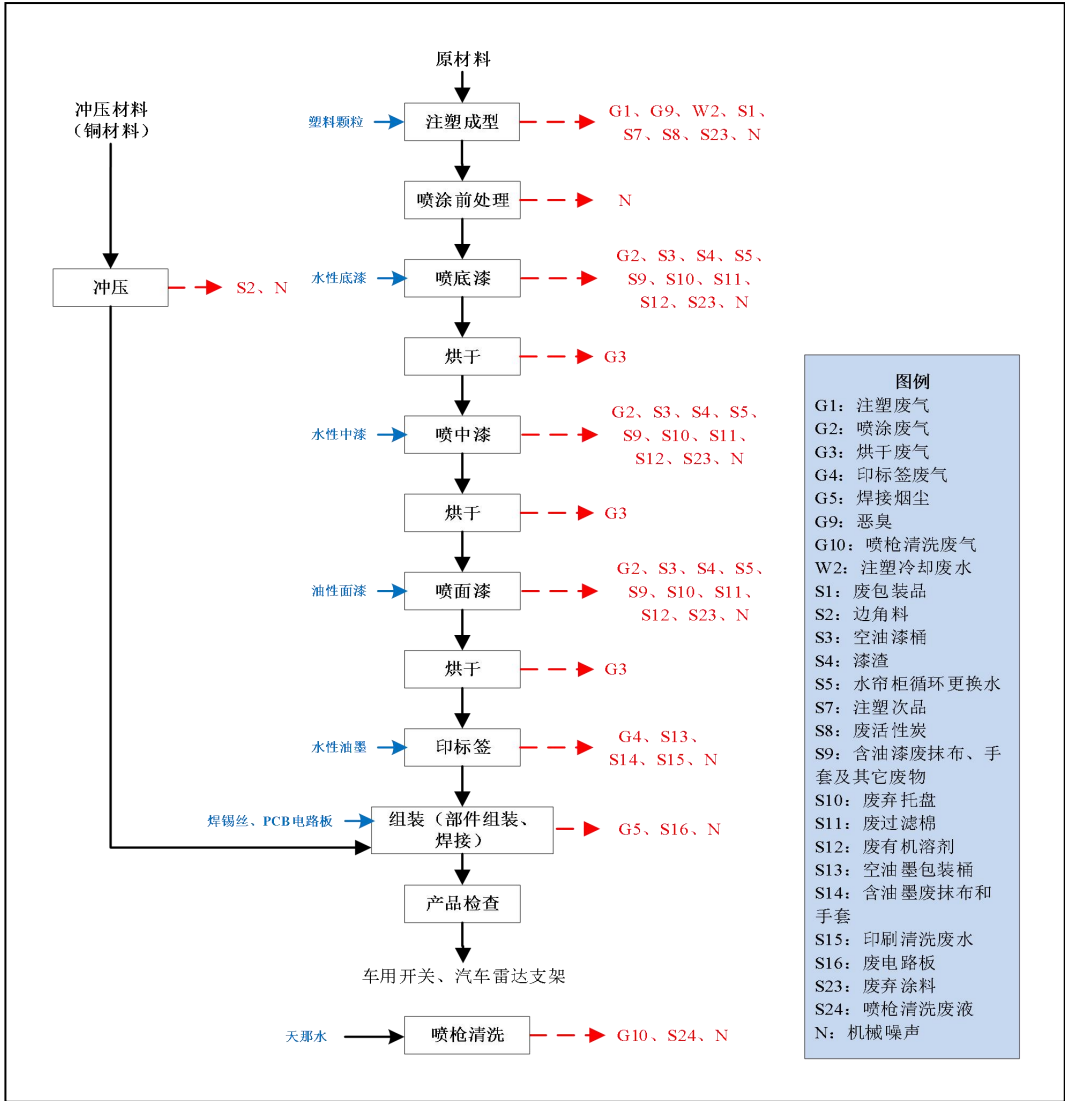
图 2-8 车用开关、汽车雷达支架的生产工艺流程图
