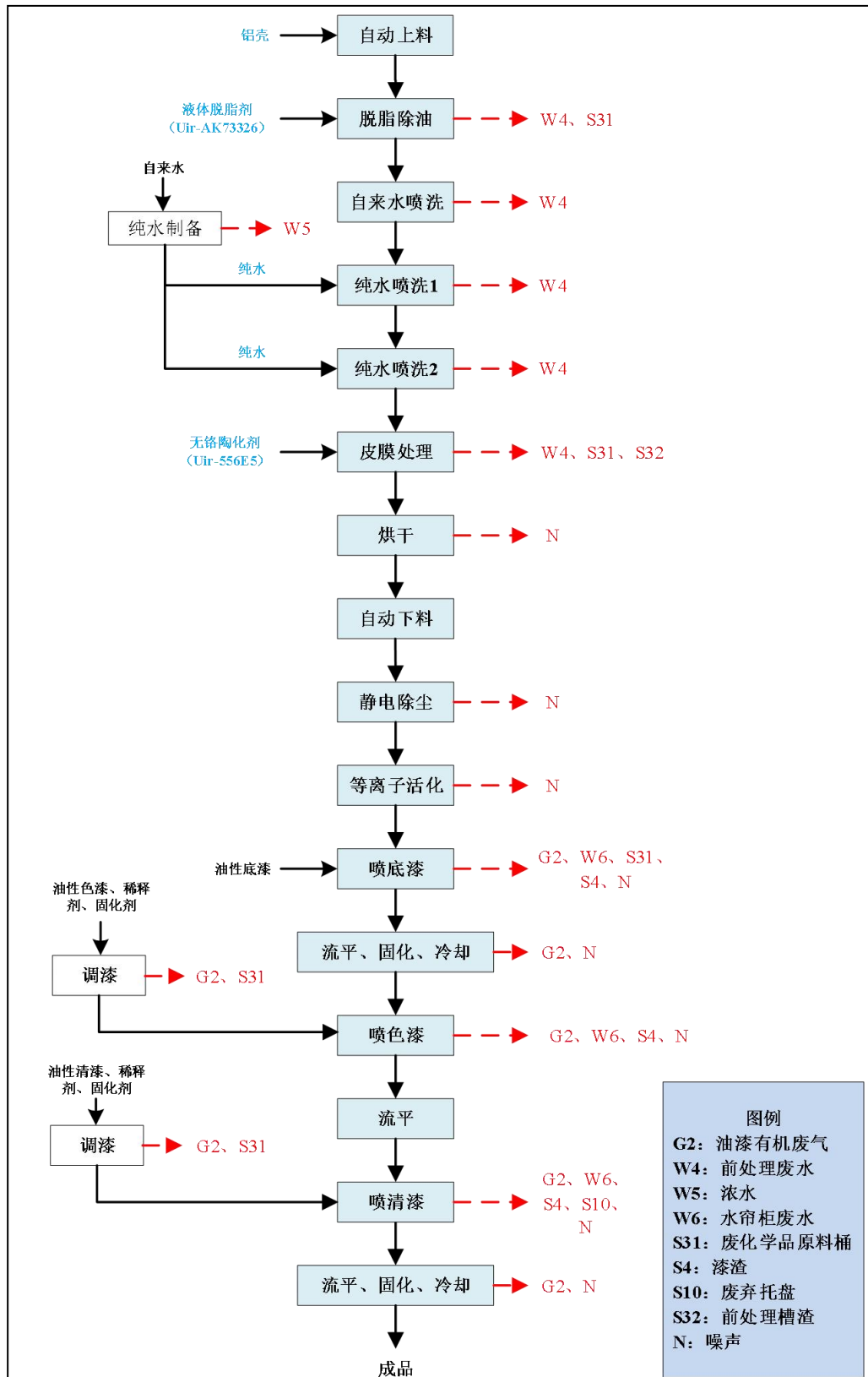
图 2-12 汽车雷达生产工艺流程图
