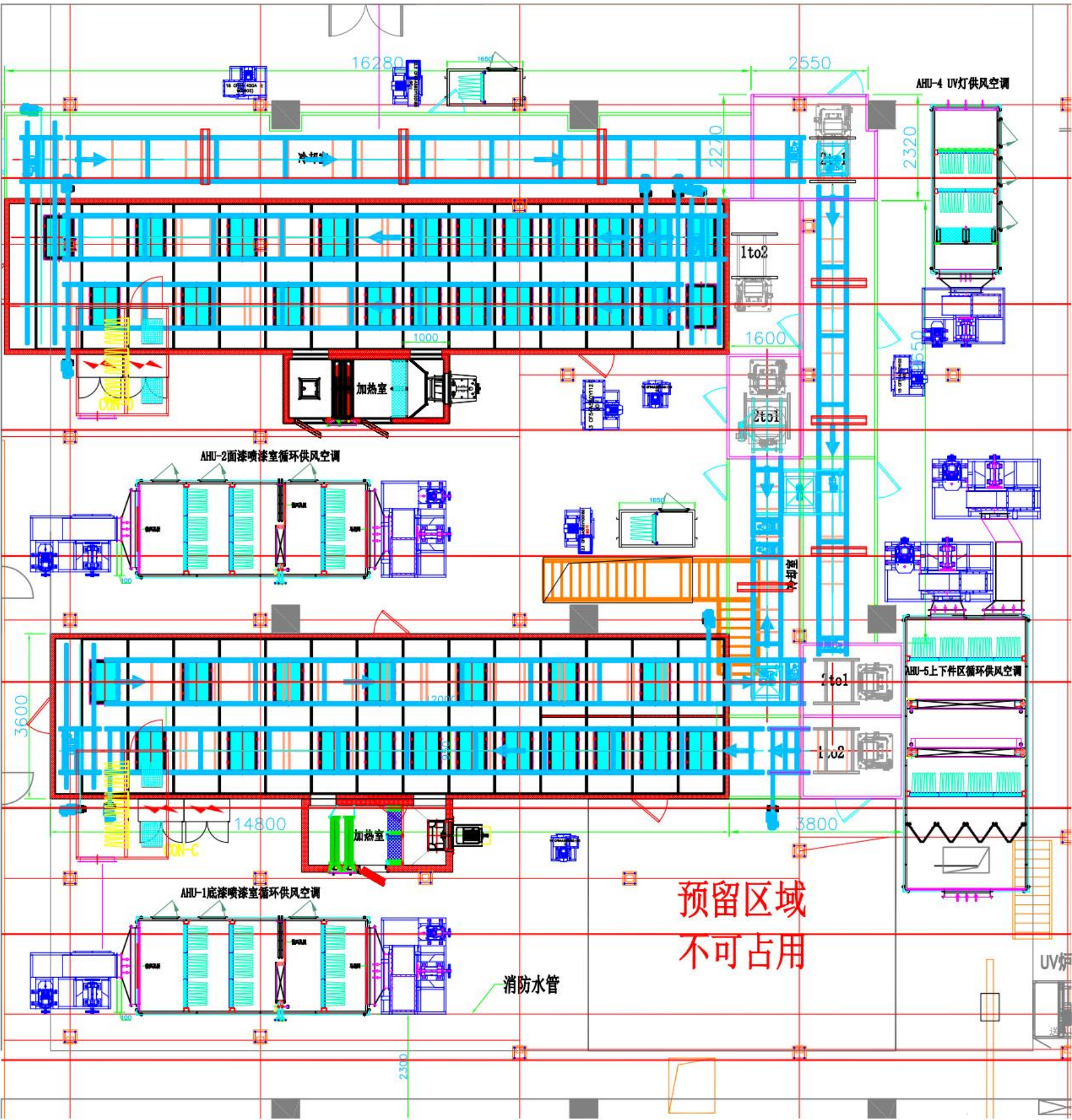
附图 6 改扩建项目喷涂 1#线二层平面布置图
