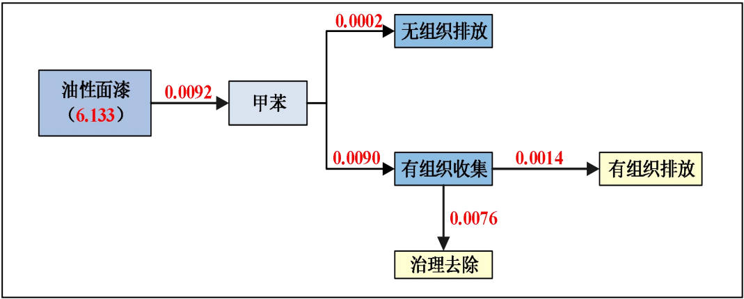
图 2-3 本次改扩建项目涂装 1#线甲苯物料平衡图 (单位: t/a)
