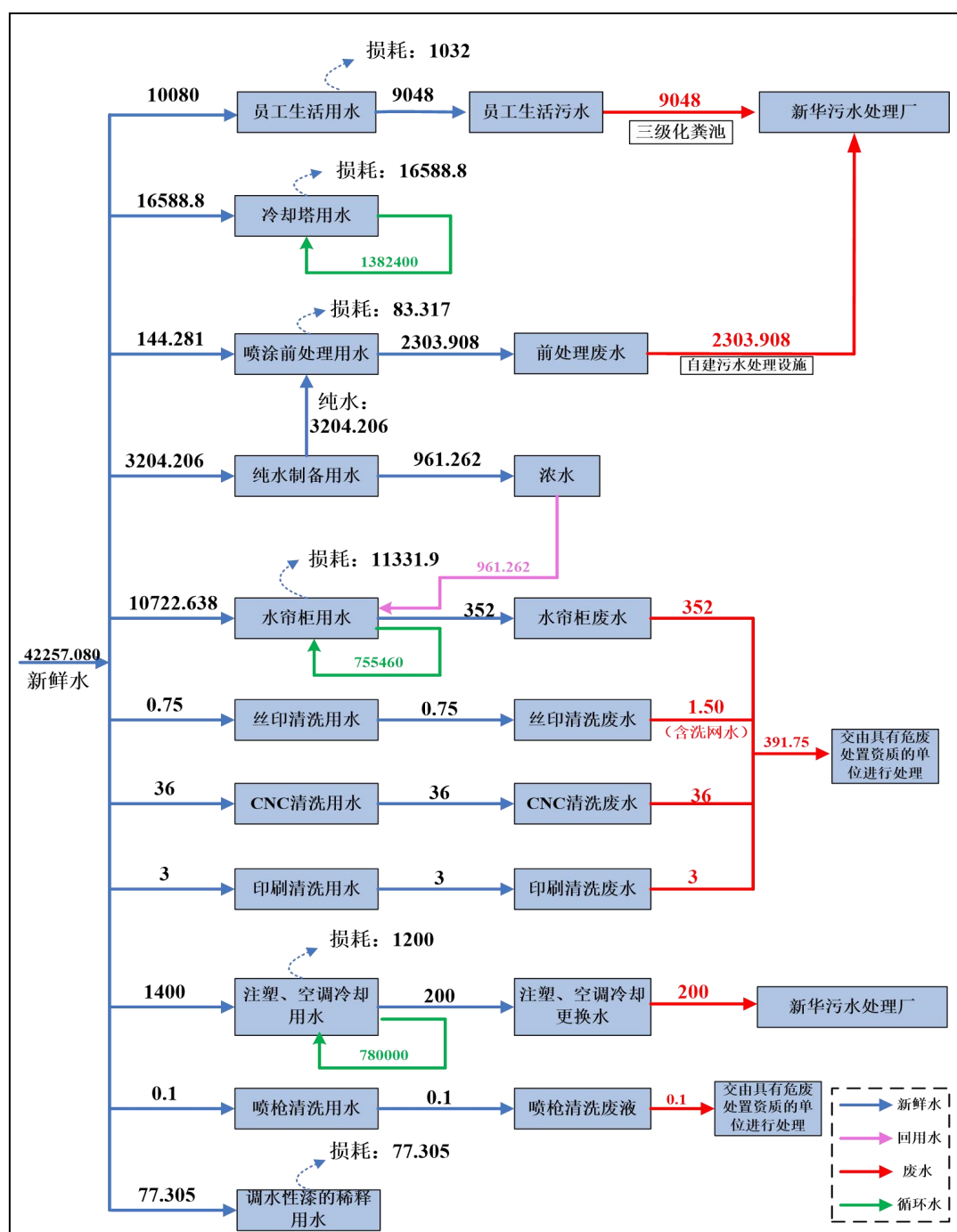
图 2-5 现有项目水平衡图 (t/a)
