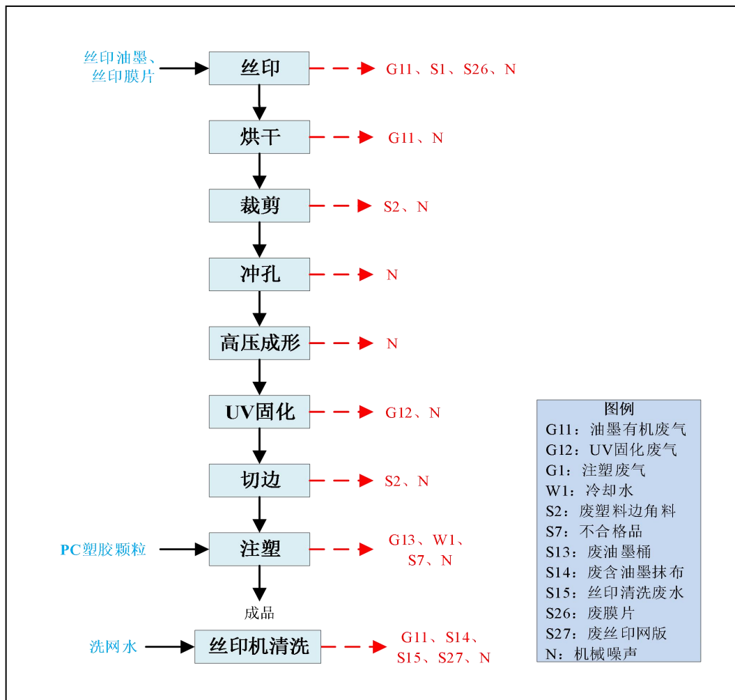
图 2-10 方向盘功能按钮的生产工艺流程图
