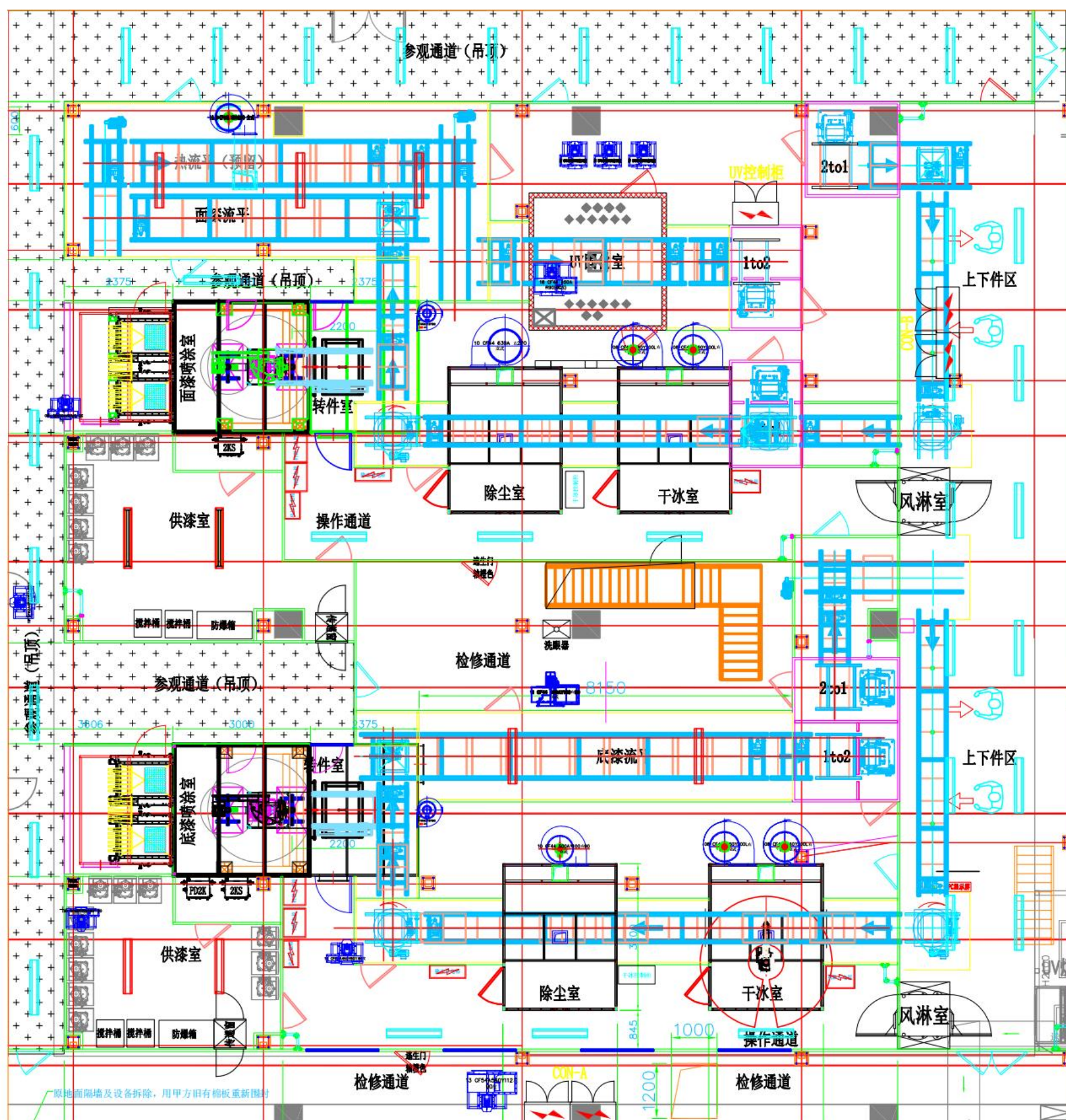
附图5 改扩建项目喷涂1#线一层平面布置图
