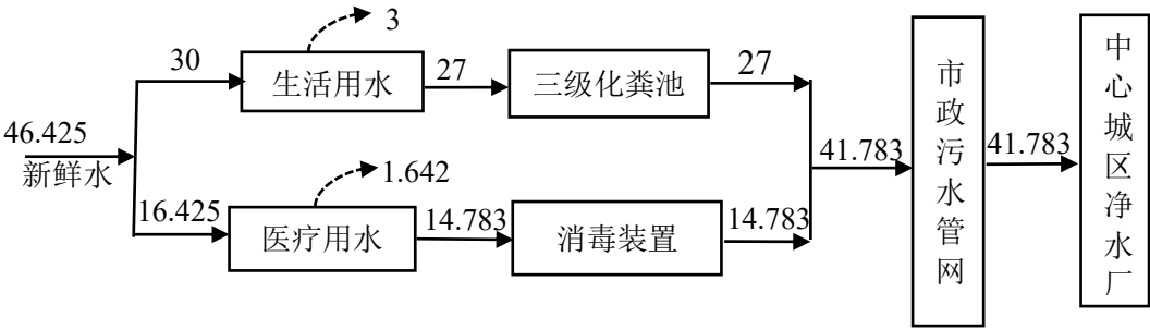
图 2-1 本项目新增用水水平衡图（单位： m 3 /a）
