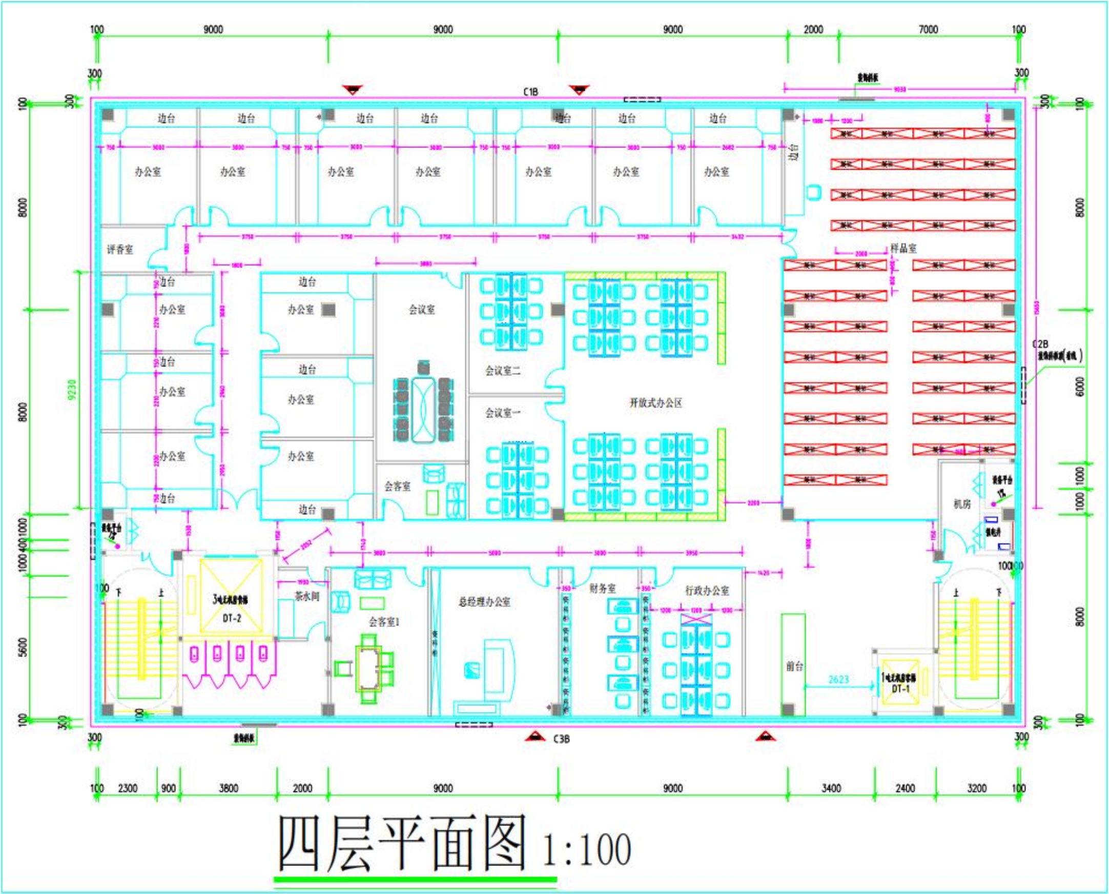
附图 3-4 项目四层平面布置图
