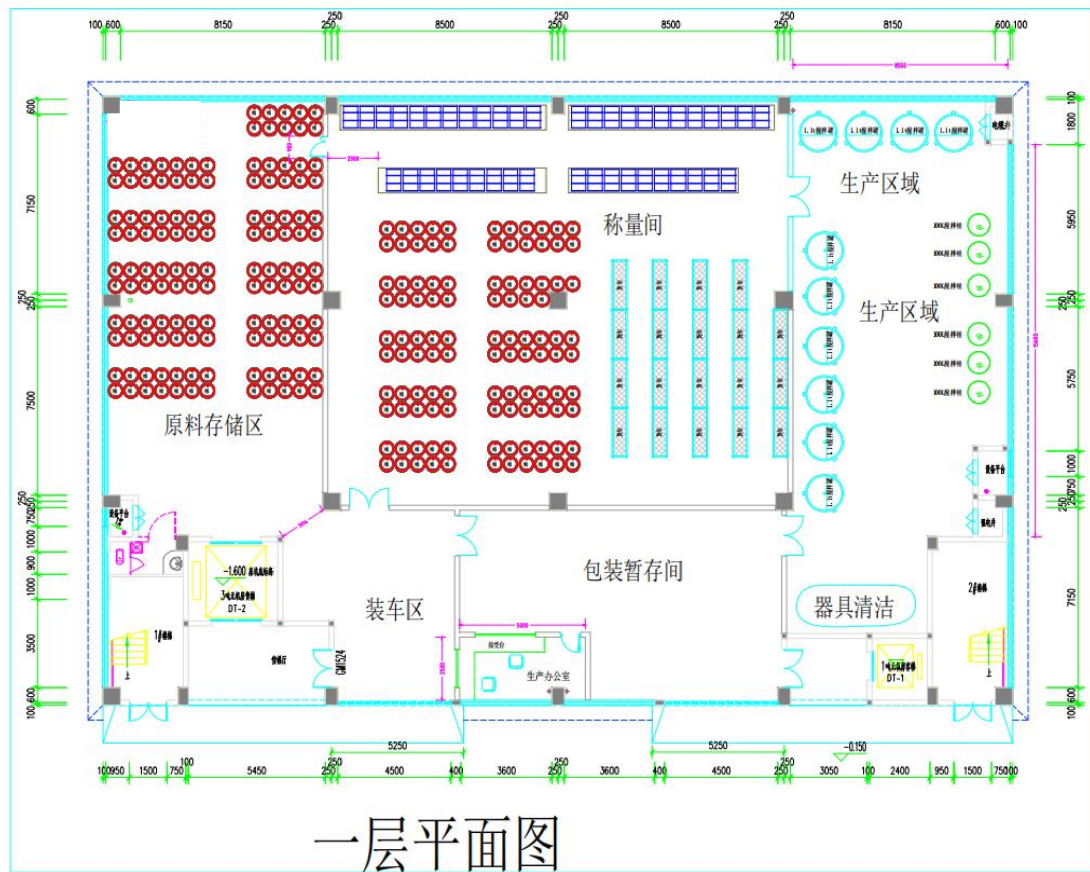
附图 3-1 项目一层平面布置图
