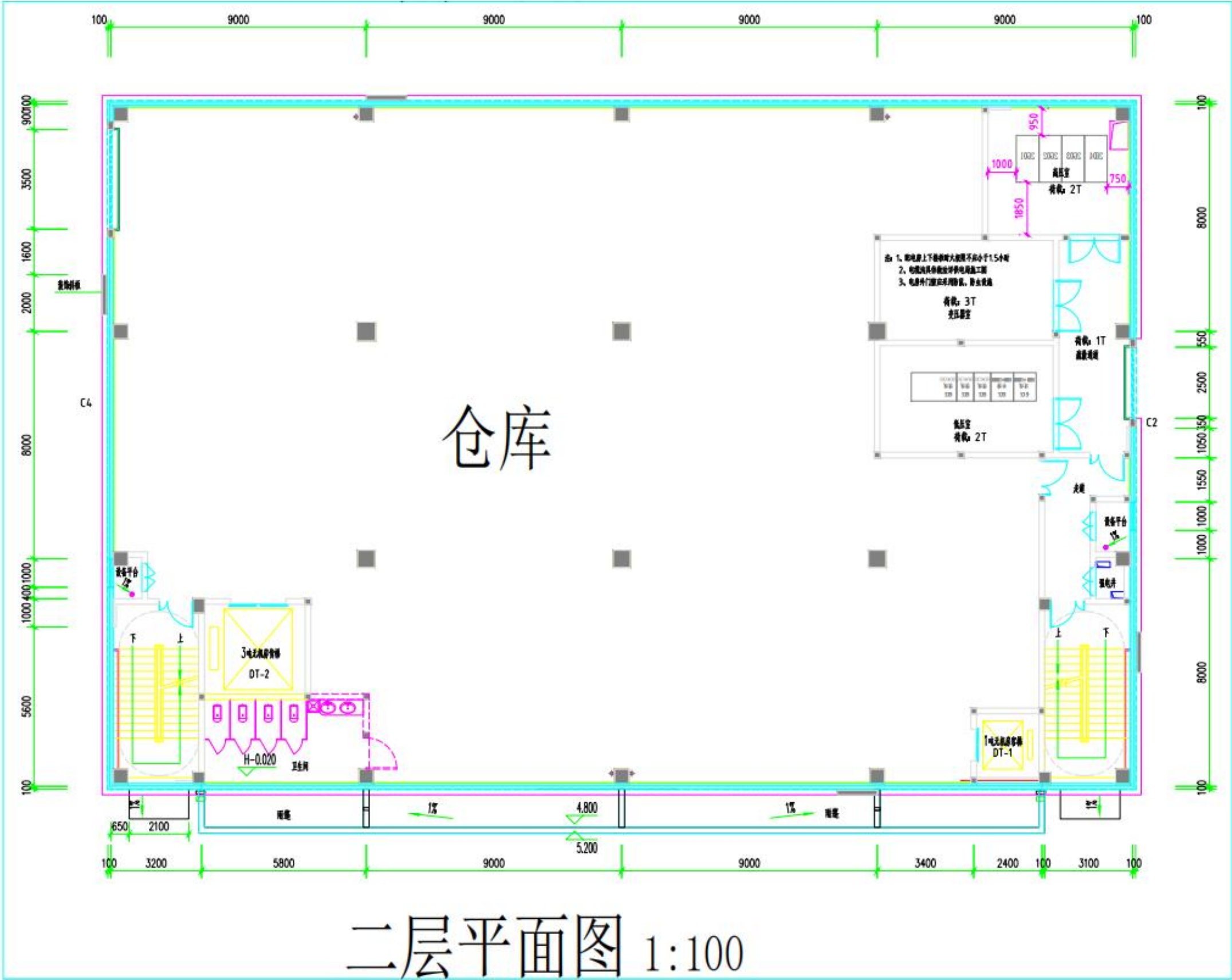
附图 3-2 项目二层平面布置图
