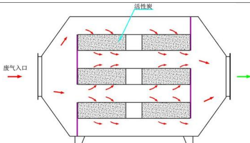
图 4-1 活性炭吸附工作原理图
