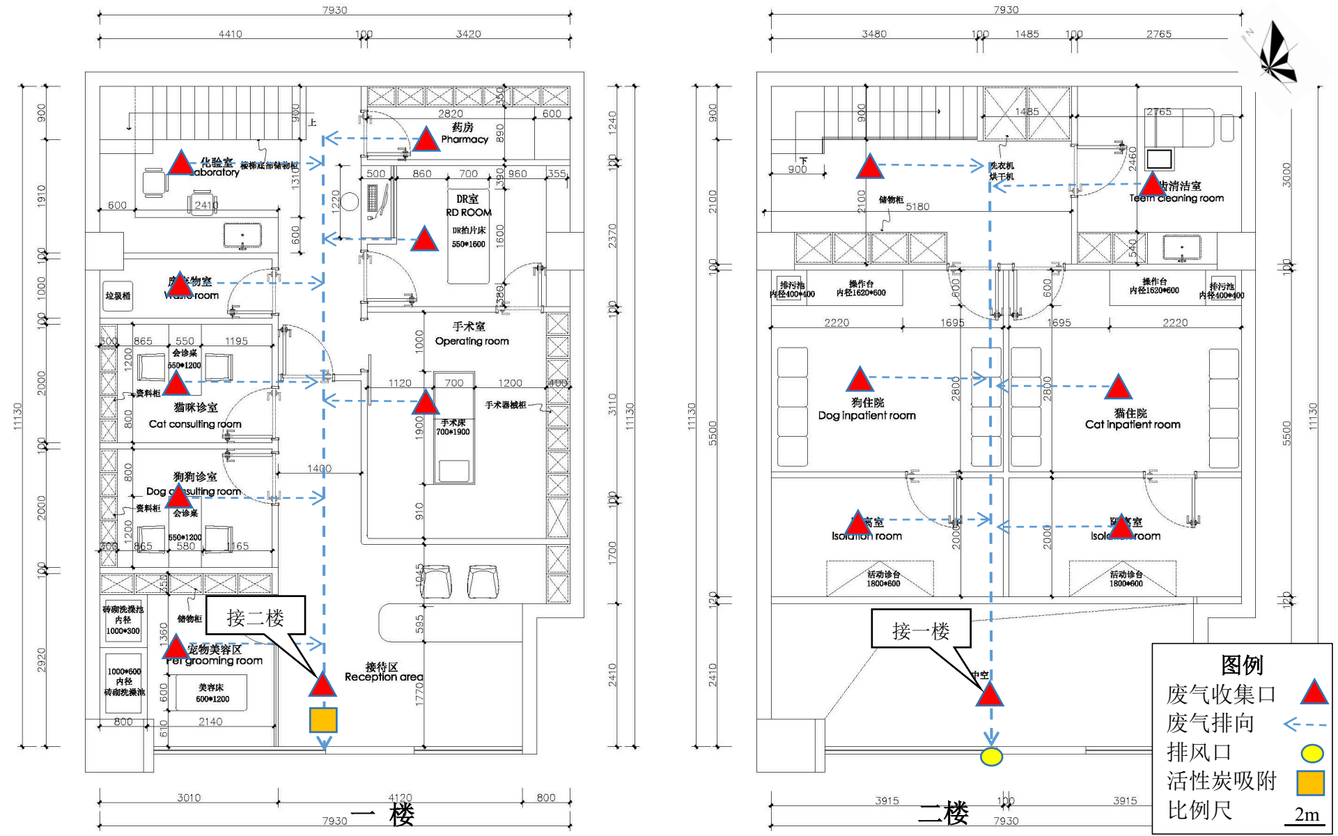
附图 4-1 项目平面布置及废气流向图
