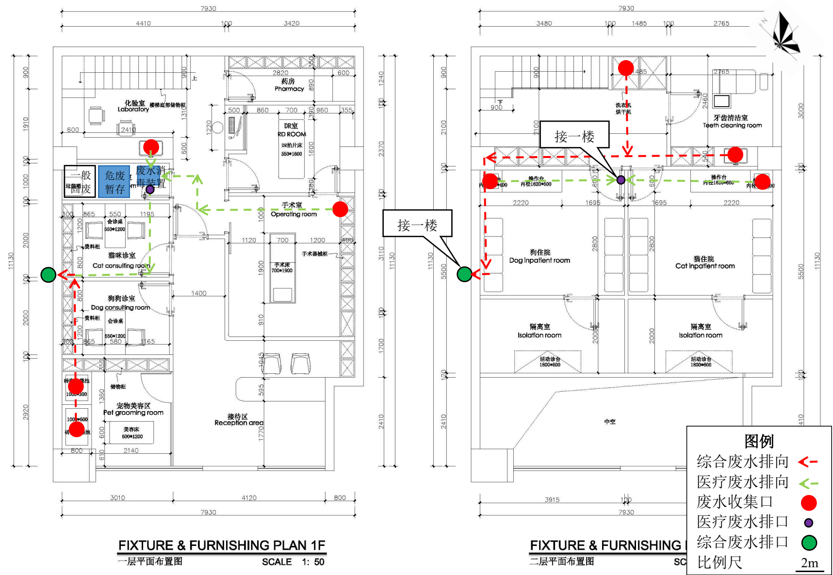
附图 4-2 项目平面布置、废水流向及分区防渗图
