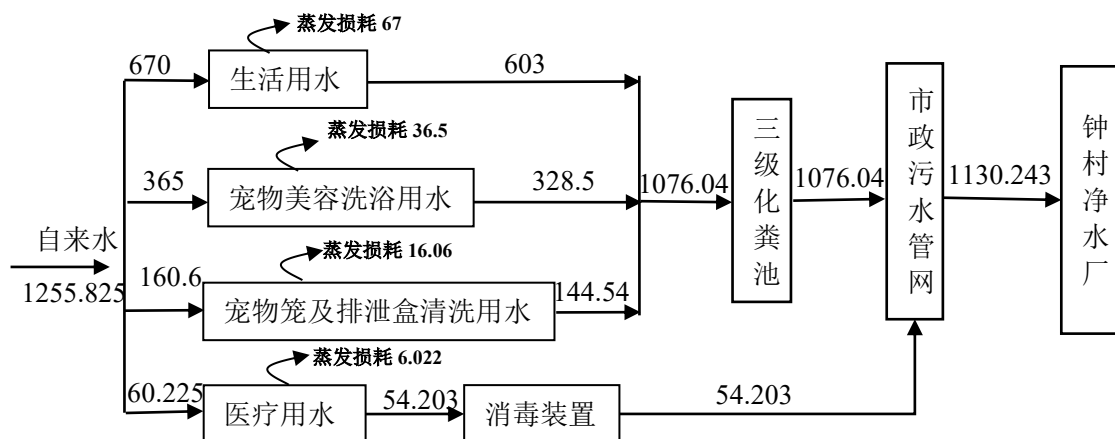
图 2-2 扩建后整体项目水平衡图 (单位: \text{m}^3/\text{a} )
