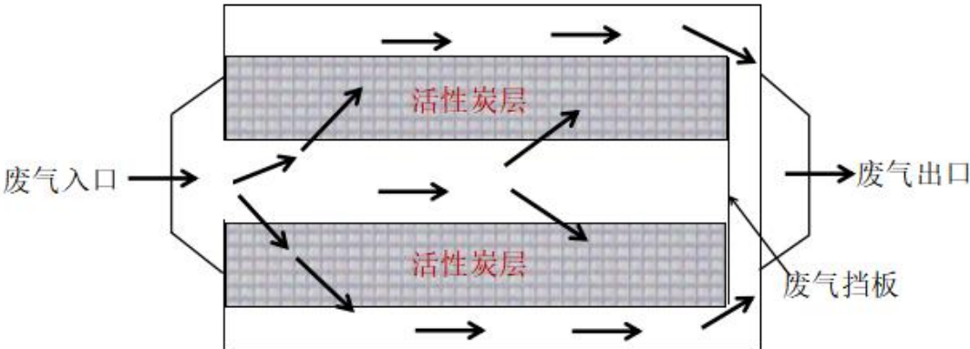
图 4-1 项目活性炭装置示意图
