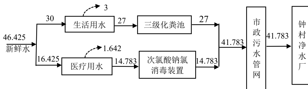
图 2-1 本项目新增用水水平衡图 (单位: \text{m}^3/\text{a} )
