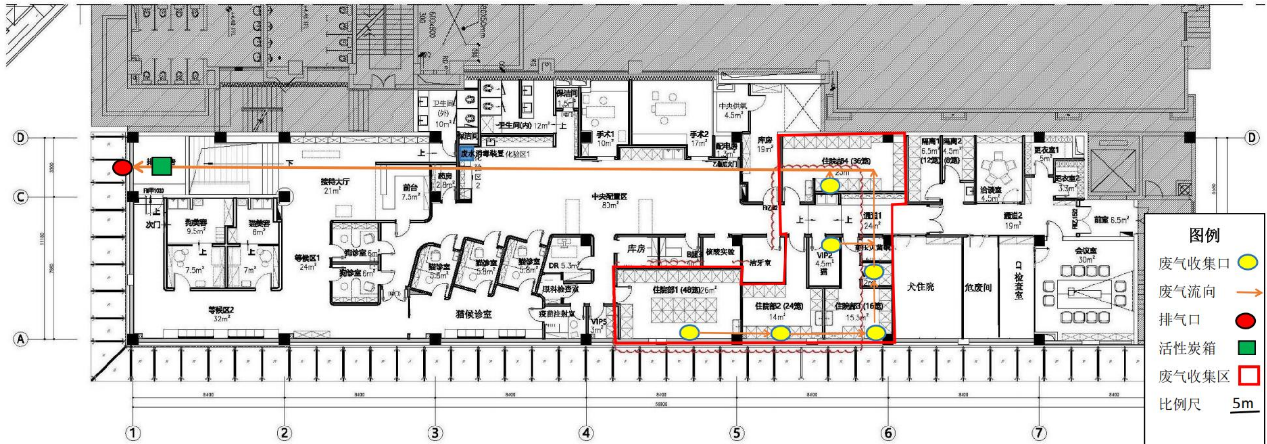
附图 4-2 项目平面布置图-排气图
