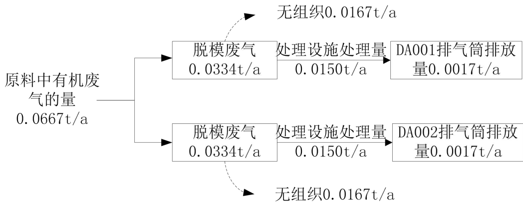
图9 项目有机废气平衡图
