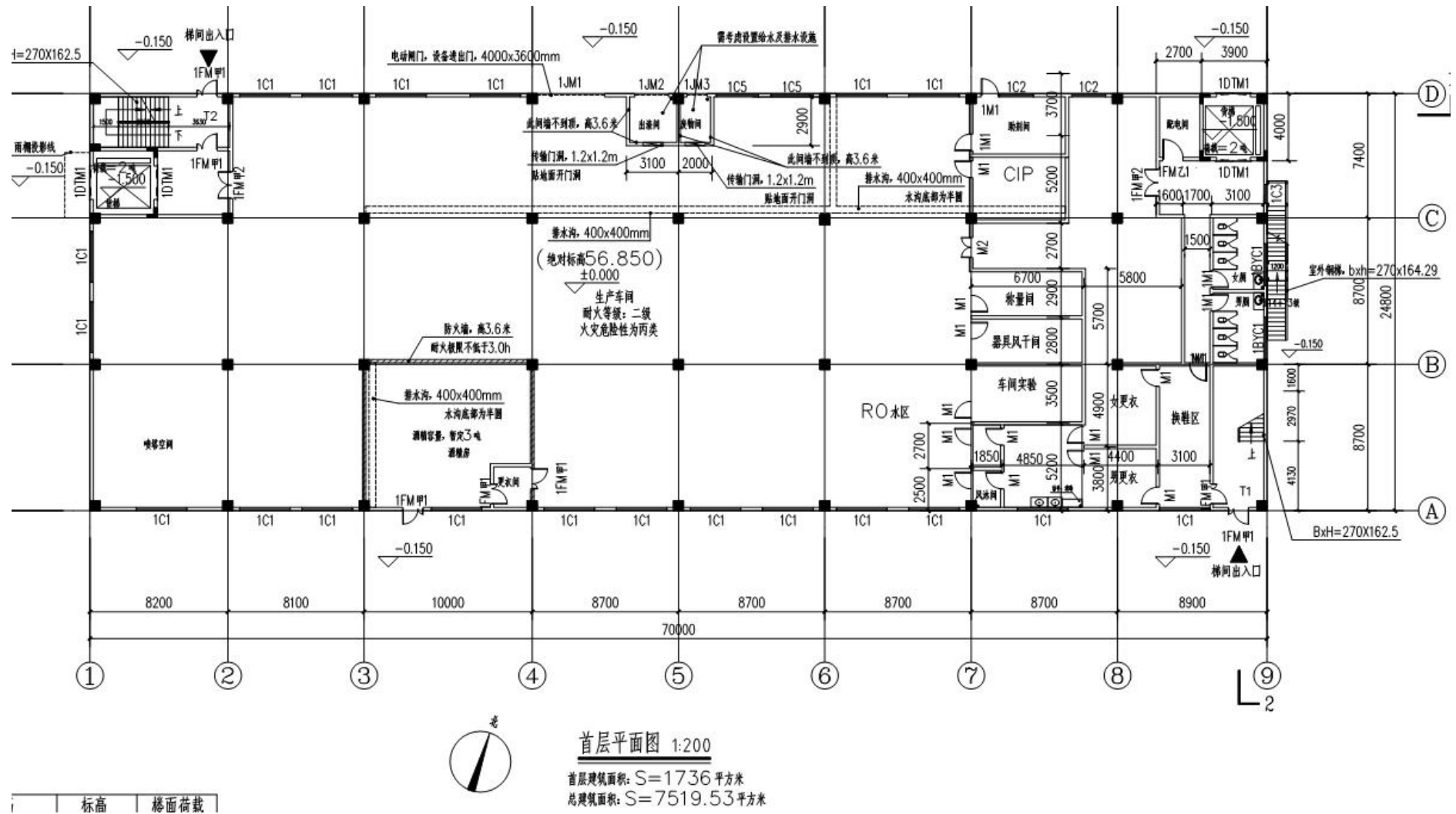
附图3 本项目各层及总平面布置图
