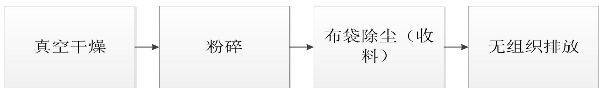
图 4-5 真空干燥粉碎工艺粉尘处理流程图
