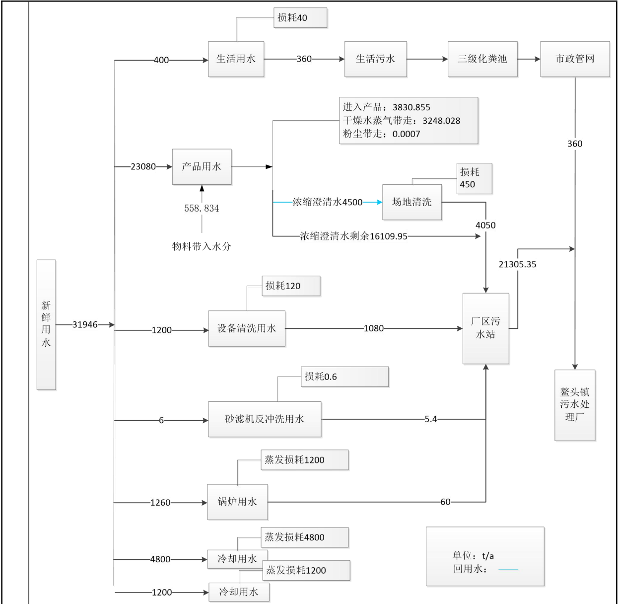
图 2-1 本二期扩建项目新增水平衡图
