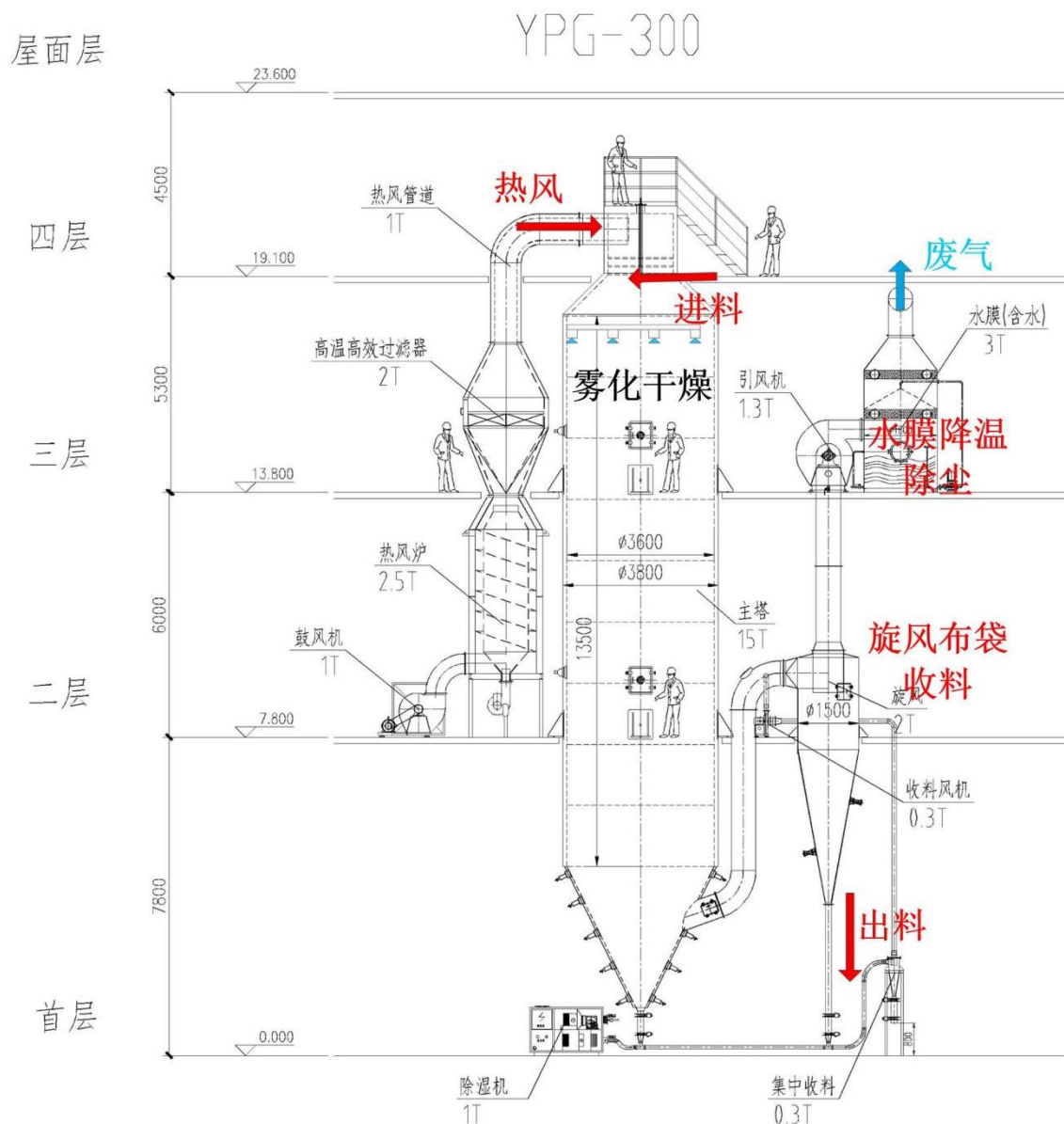
图 4-6 喷塔干燥机结构图
