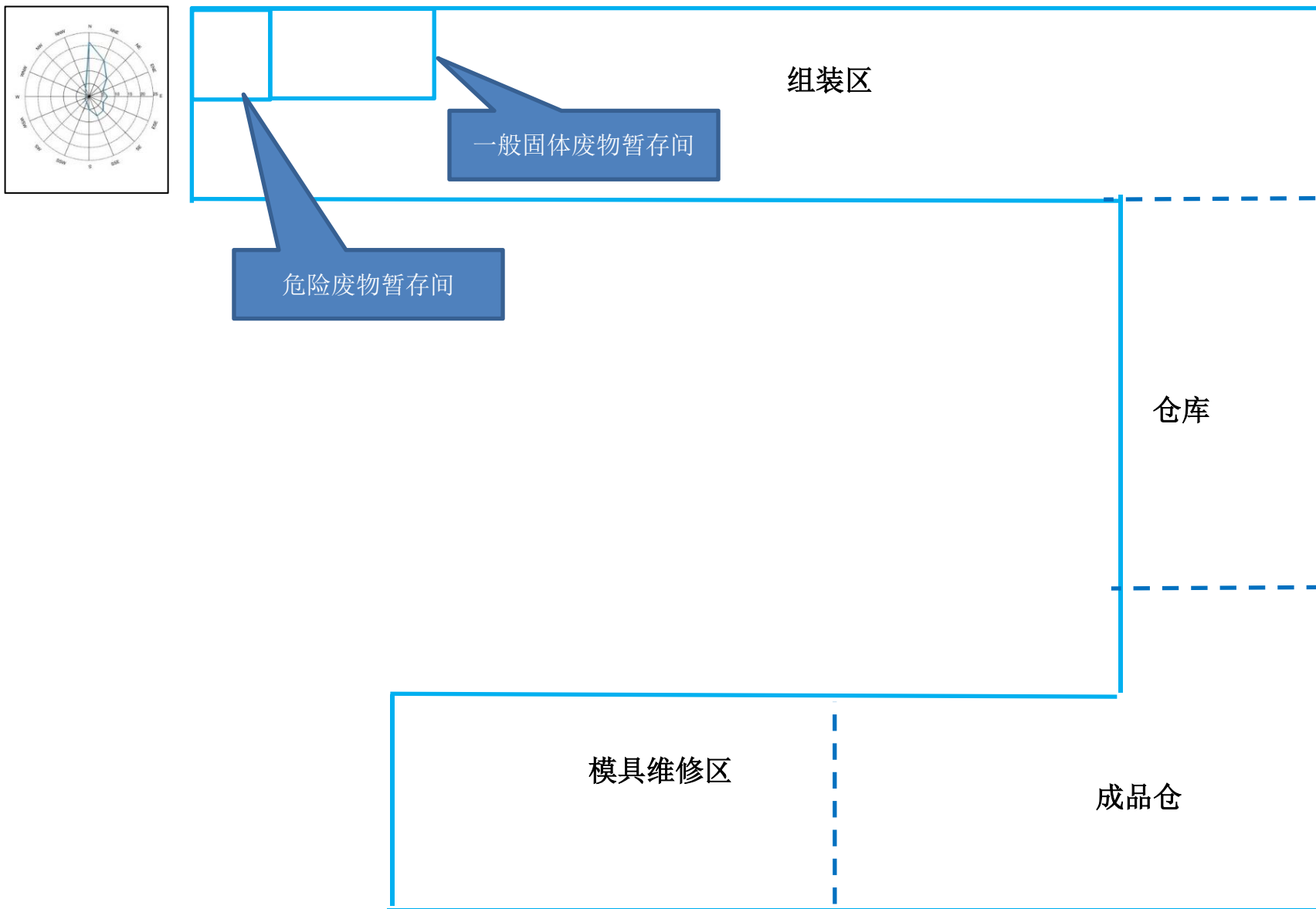
附图 5-3 项目生产车间 2 (1F) 平面图 (1:200)
