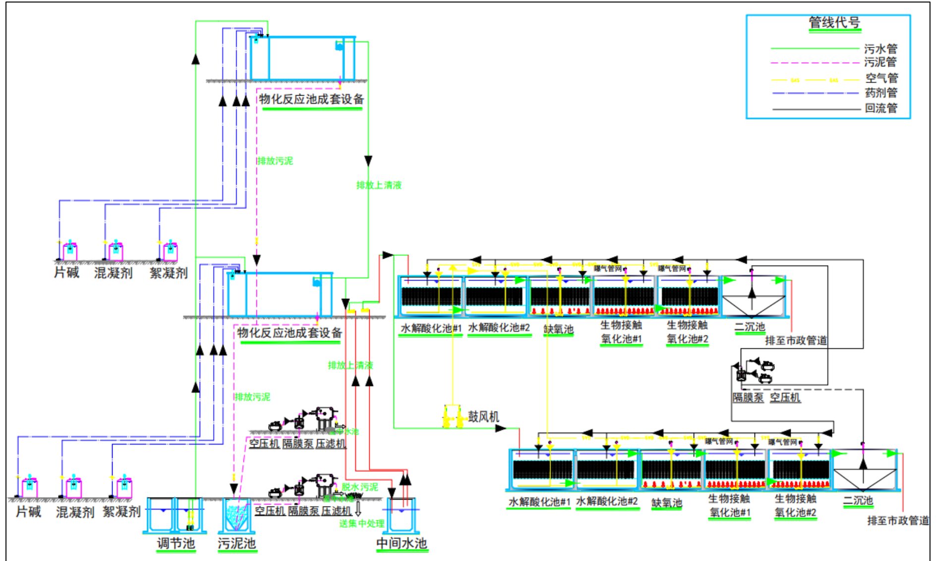
图 3.2-4 污水处理工艺流程及设备连接示意图
