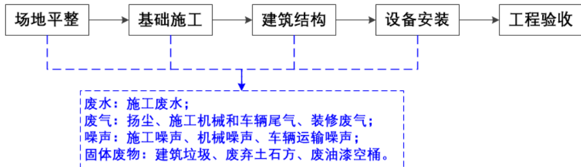
图 3.3-1 施工期工艺流程及产污环节图
