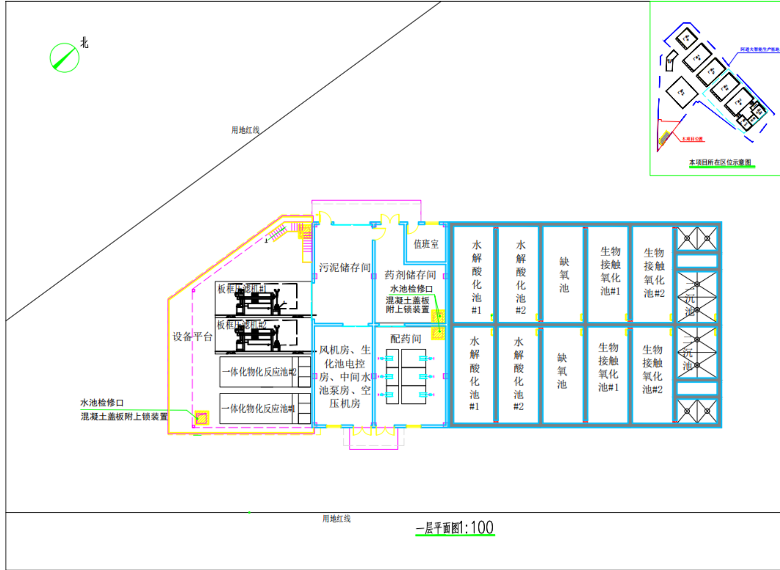
图 3.1-7 污水处理站一层平面图
