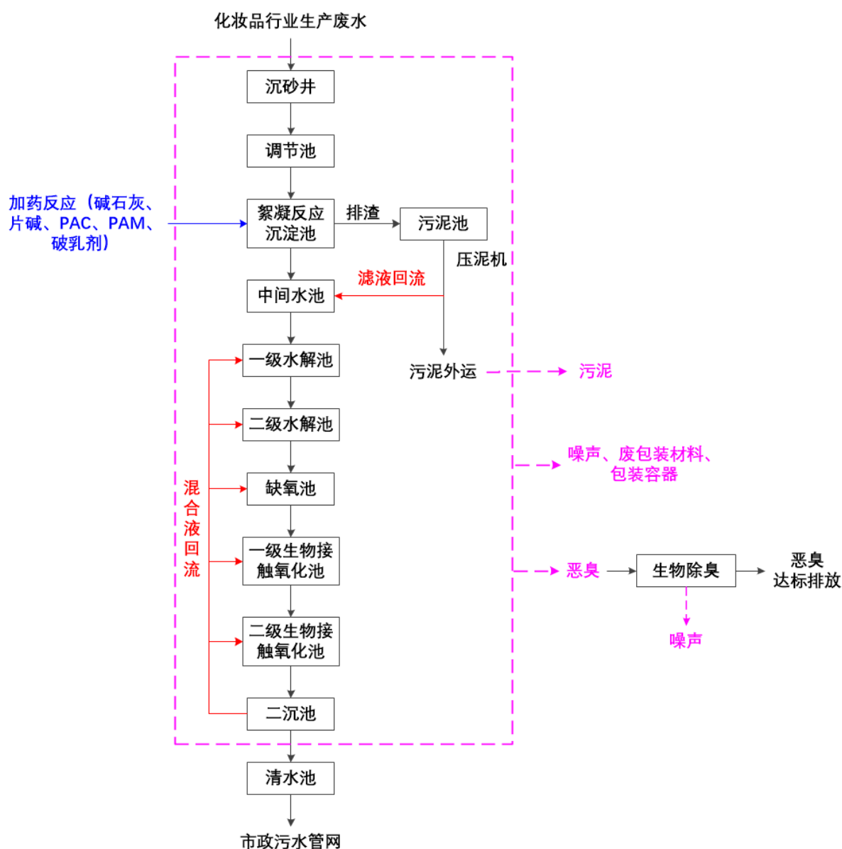
图 3.4-1 本项目污水处理工艺流程及产污环节图
