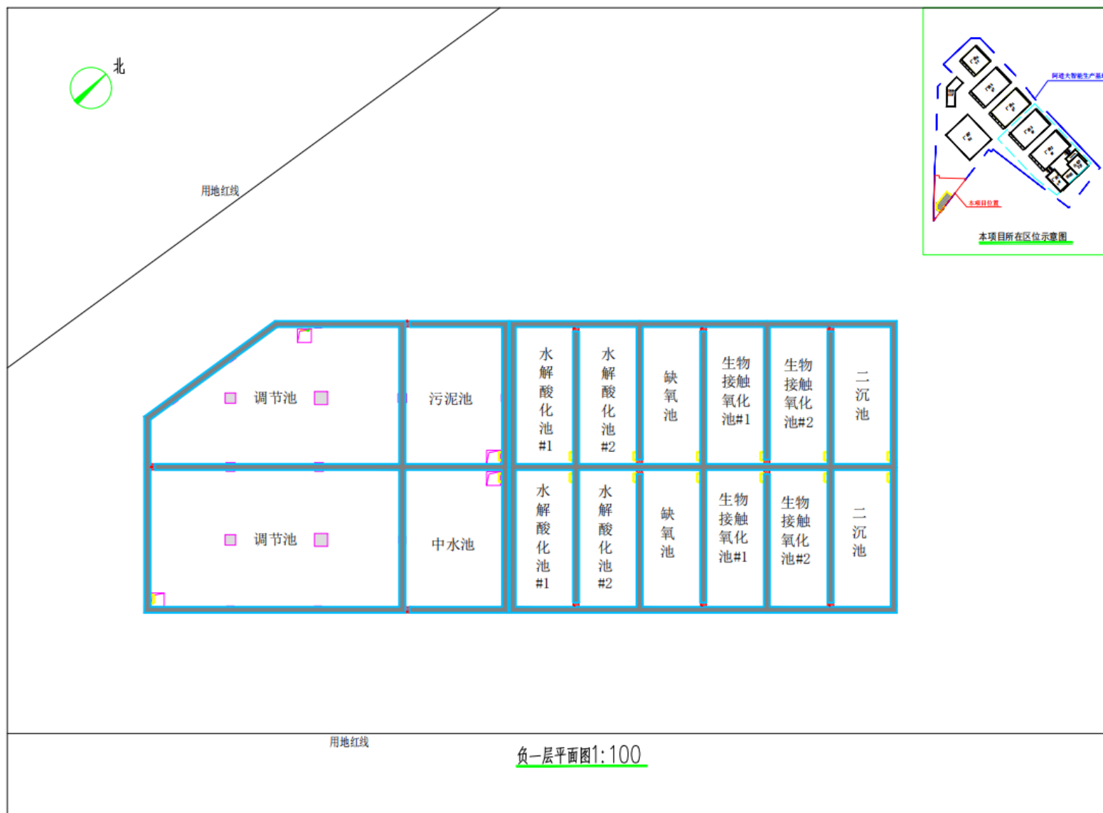
图 3.1-6 污水处理站负一层平面图
