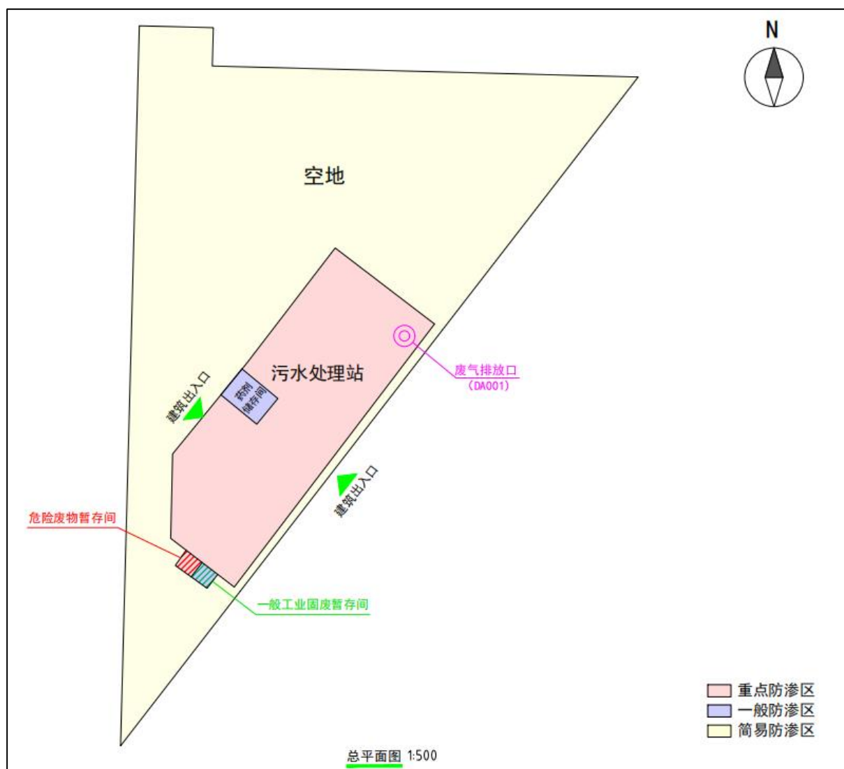
图 6.5-3 项目分区防渗示意图
