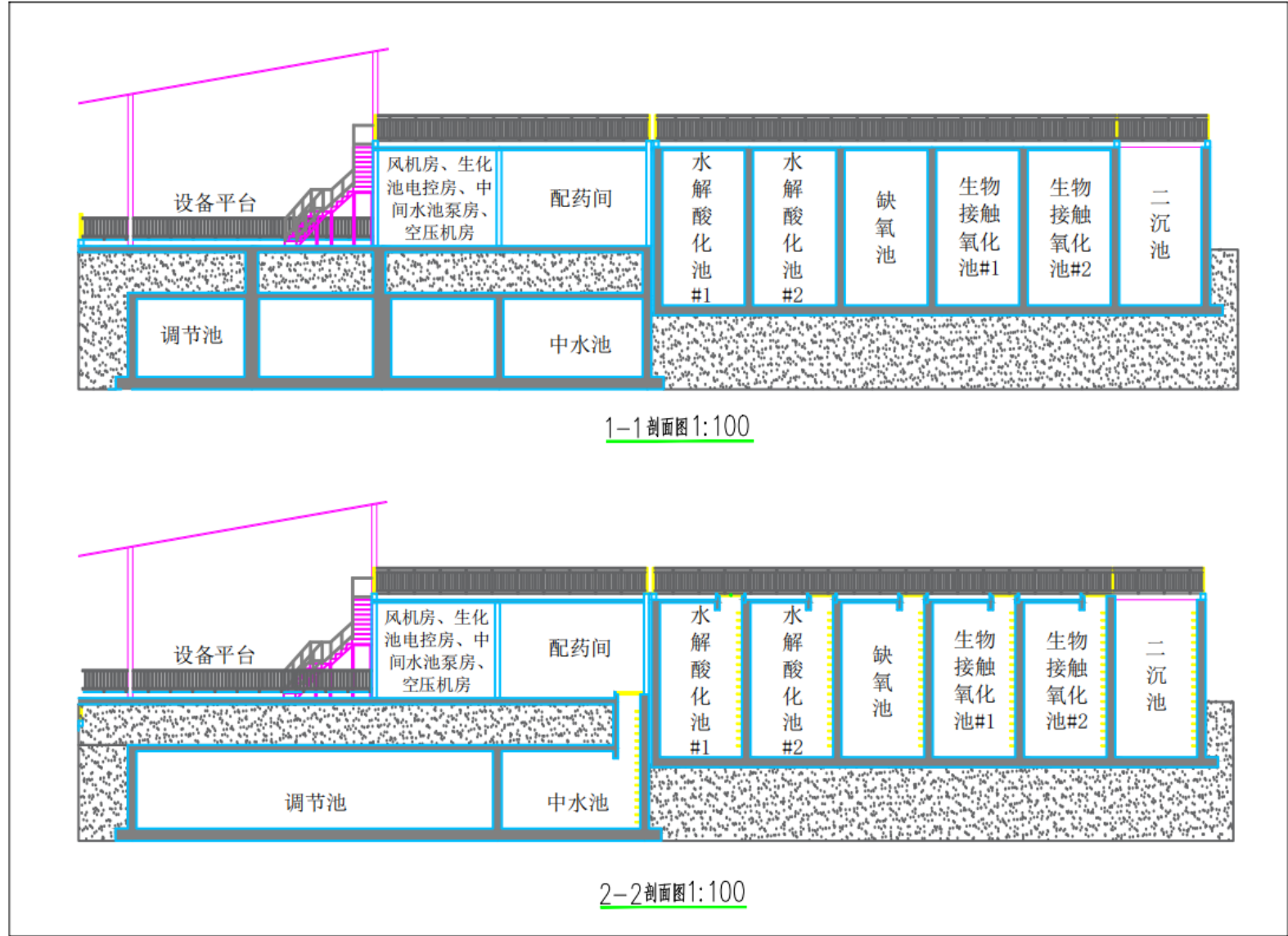
图 3.1-10 污水处理站剖面图（一）
