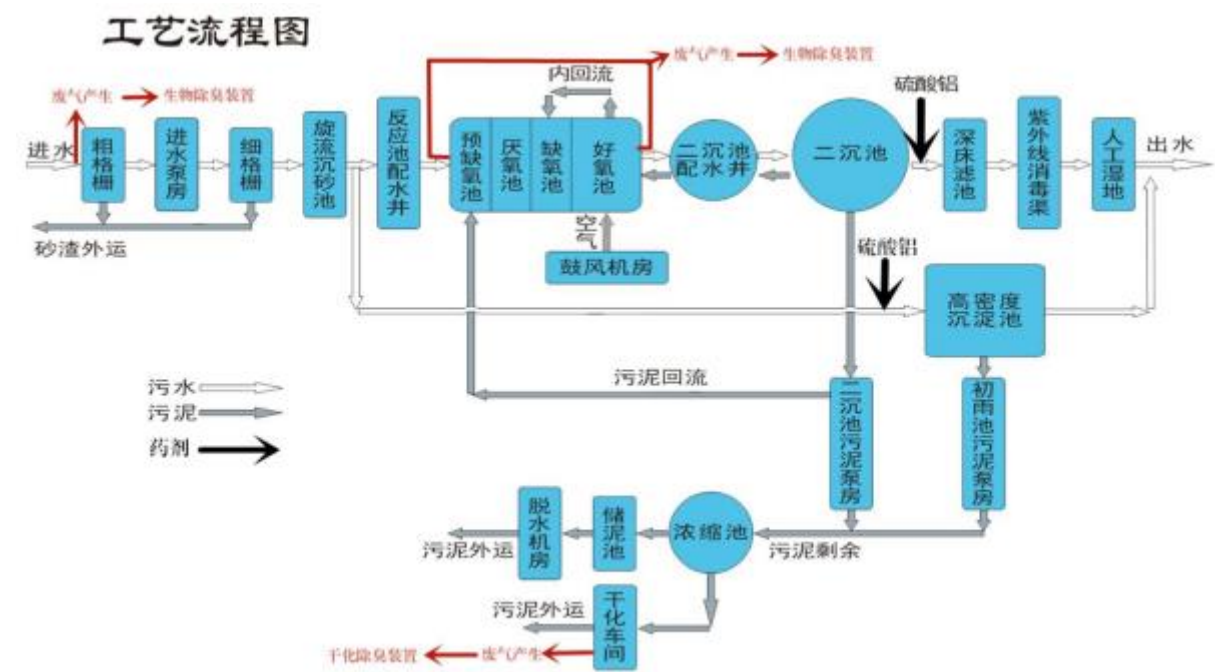
图 6.1-1 竹料污水处理厂污水处理工艺流程图
