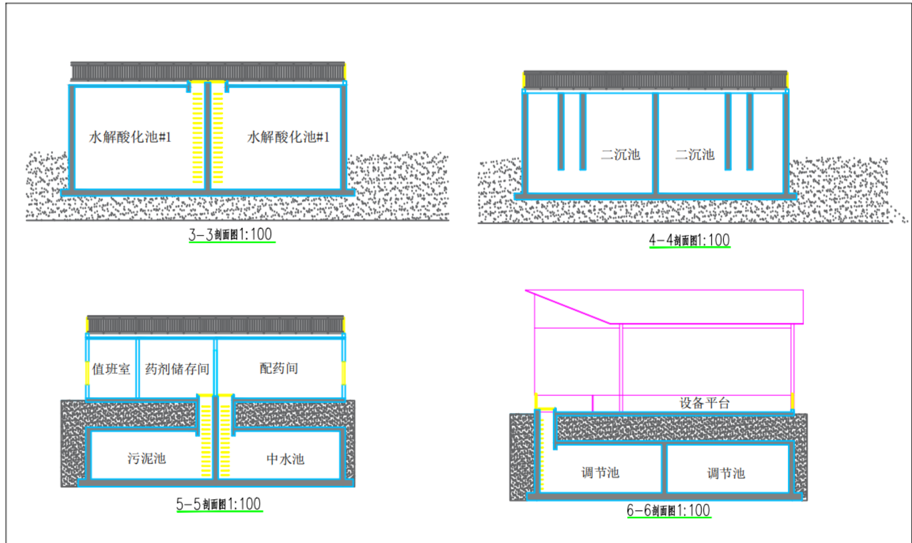
图 3.1-11 污水处理站剖面图（二）
