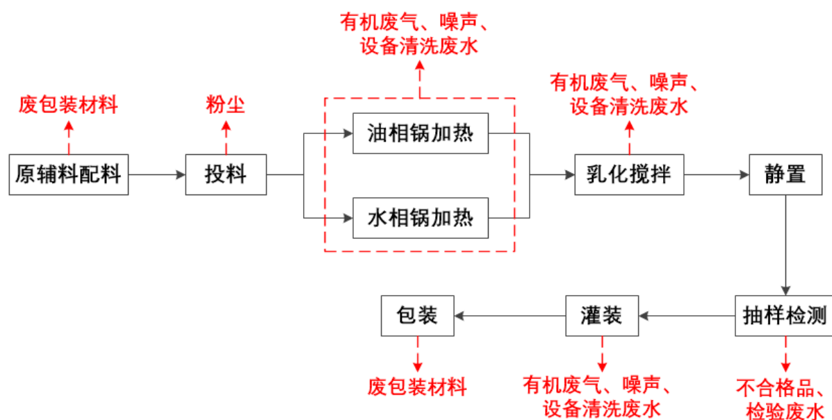
图 3.2-1 乳液、面膜、面霜主要生产工艺流程及产污环节图
