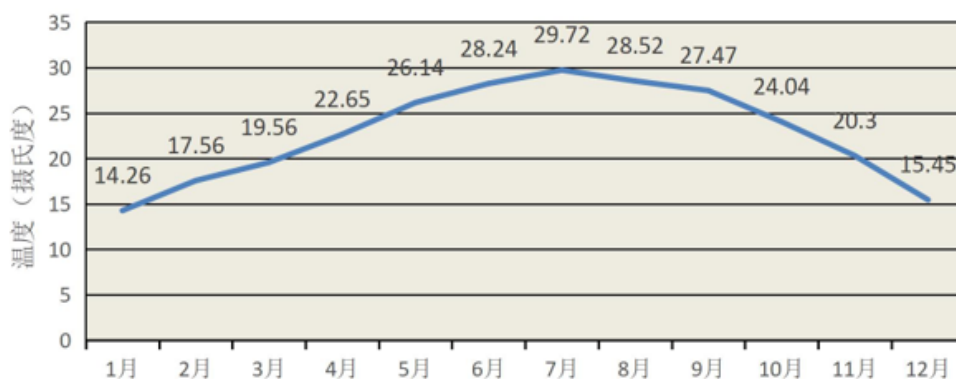
图 6.2-2 本地区 2023 年平均气温月变化图
