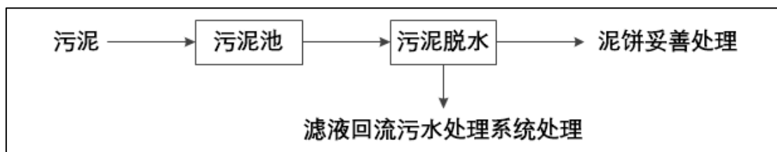
图 3.2-5 污泥处理流程图
