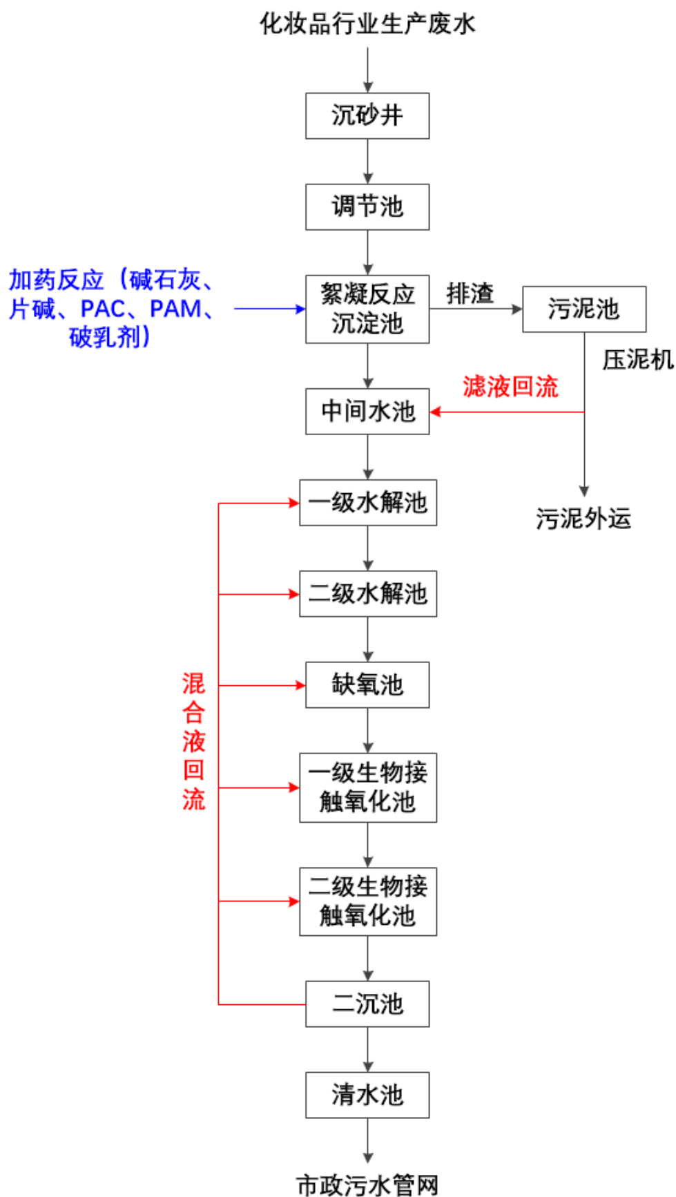
图 3.2-3 本项目污水处理工艺流程图
