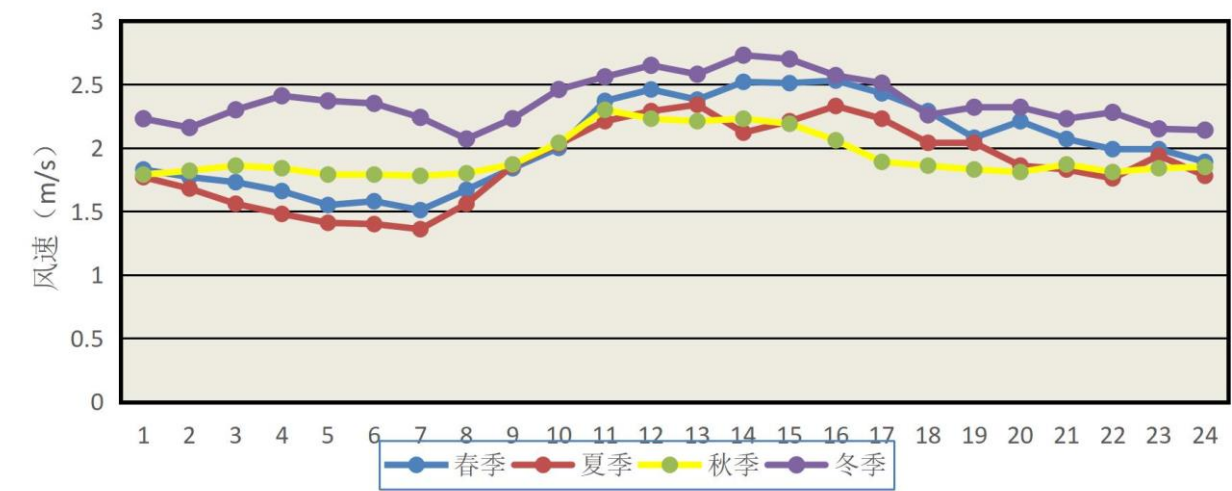
图 6.2-4 本地区 2023 年季小时平均风速的日变化图
