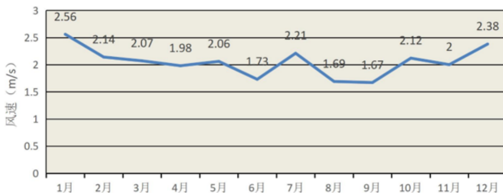
图 6.2-3 本地区 2023 年平均风速月变化图
