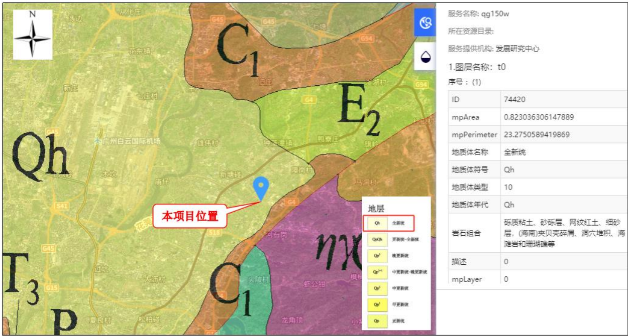
图 6.5-1 区域地质图
