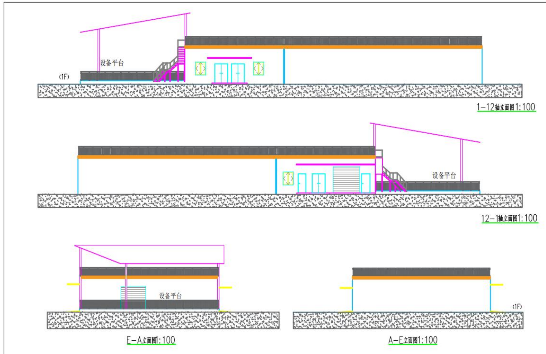
图 3.1-9 污水处理站立面图
