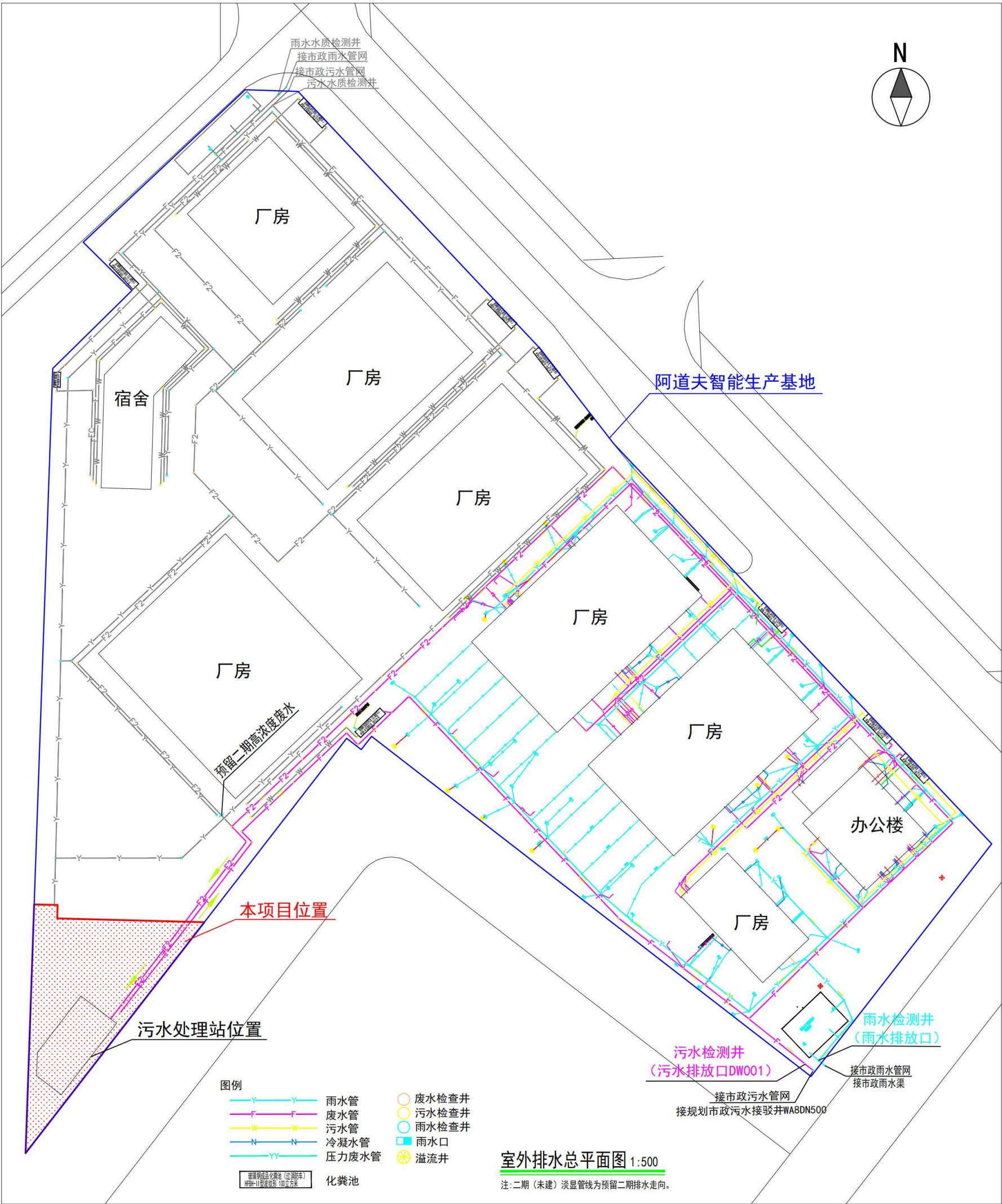
图 3.1-1 项目雨污排水走向图
