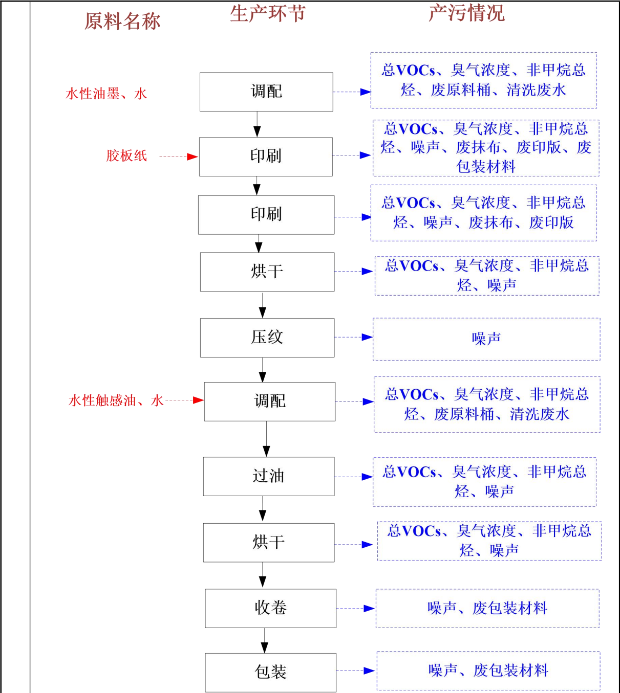
图 2-4 项目触感纸工艺流程图
