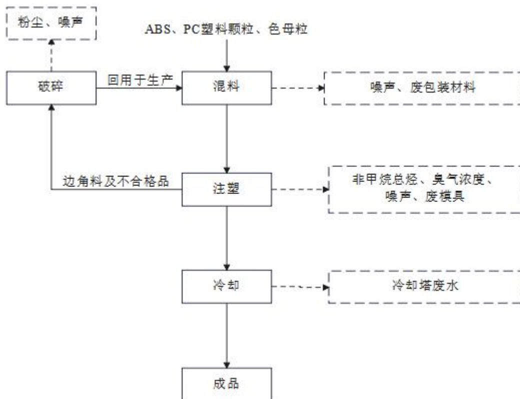
图 2-3 行李箱箱壳生产工艺流程及产污图
