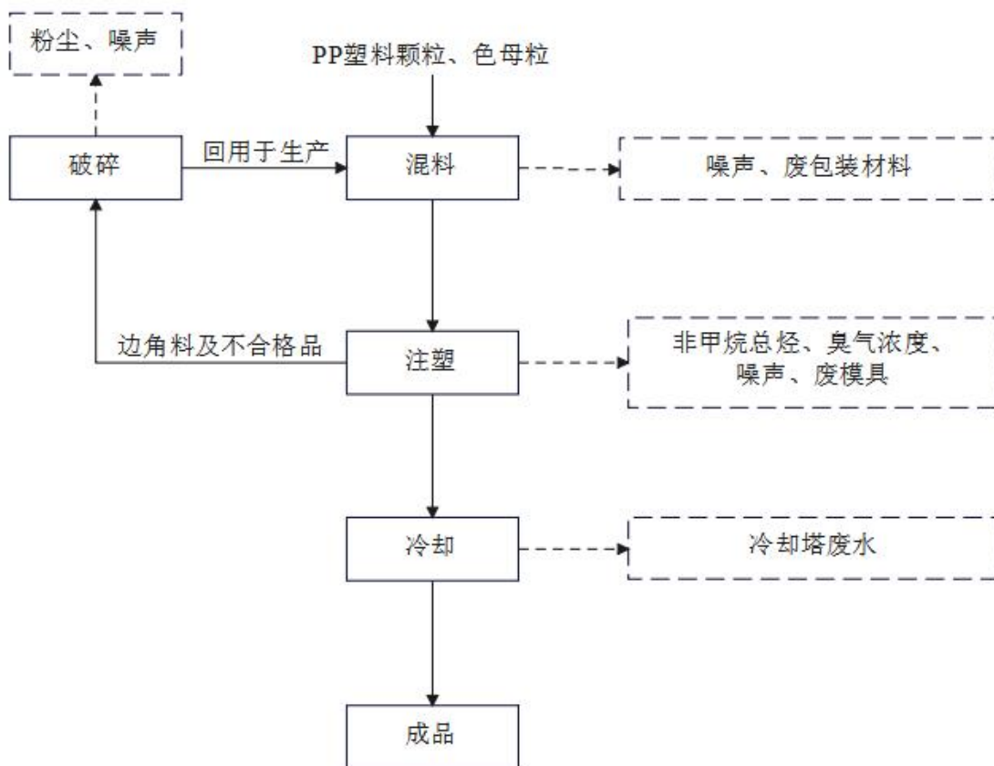
图 2-2 汽车零部件生产工艺流程及产污图
