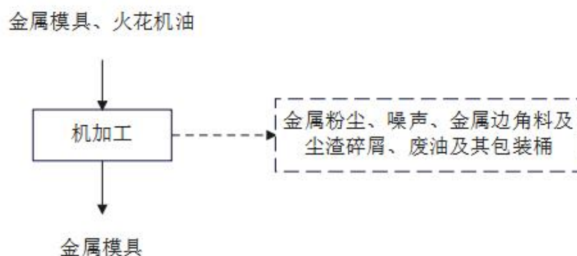
图 2-4 模具加工工艺流程及产污图
