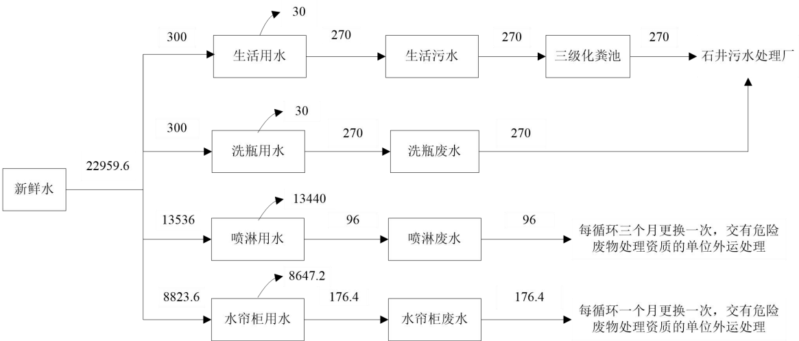
图1 本项目水平衡图 (t/a)
