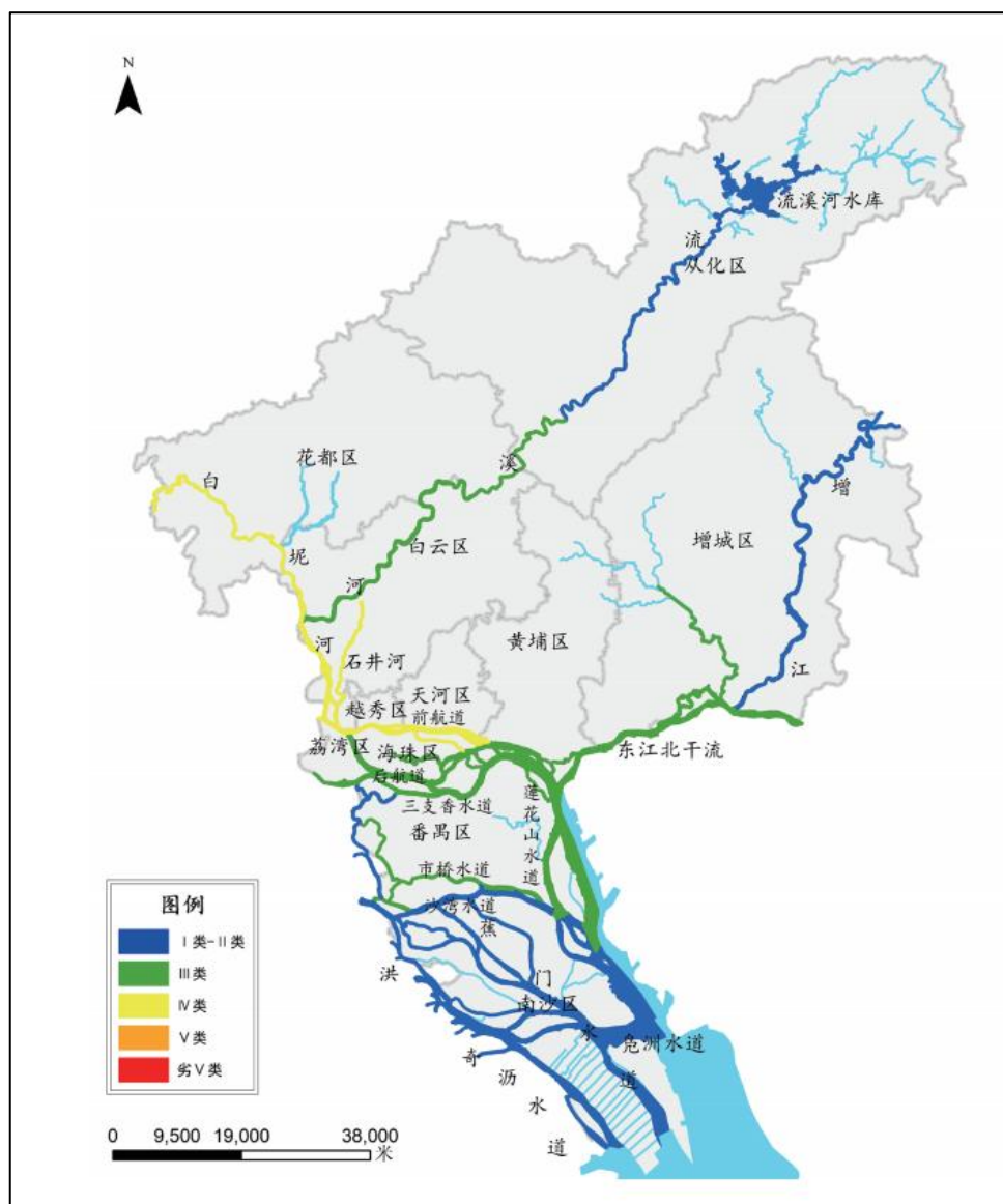
图5 2023年广州市水环境质量状况
