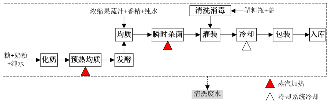
图 2-5 现有项目营养快线及乳饮料的生产工艺流程及产污环节图
