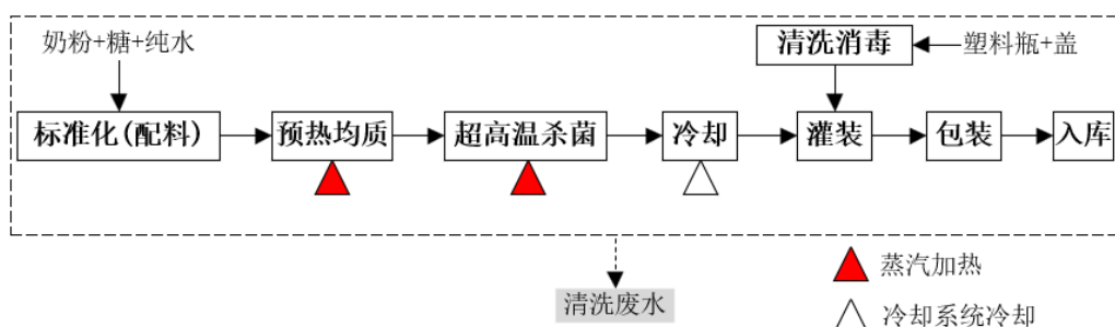
图 2-11 蛋白饮料的生产工艺流程及产污环节图（已停产）
