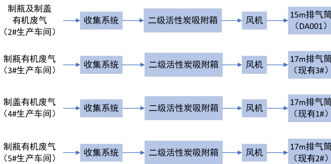
图 4-2 改扩建后的废气处理工艺流程图
