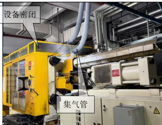
制坯机废气收集示意图
