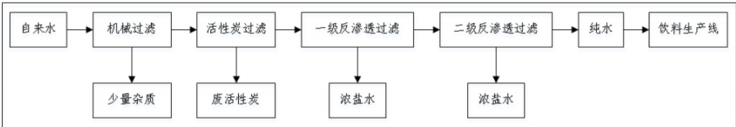
图 2-7 现有项目纯水制备工艺流程及产污环节图
