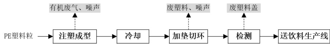
图 2-8 现有项目制盖工艺流程及产污环节图
