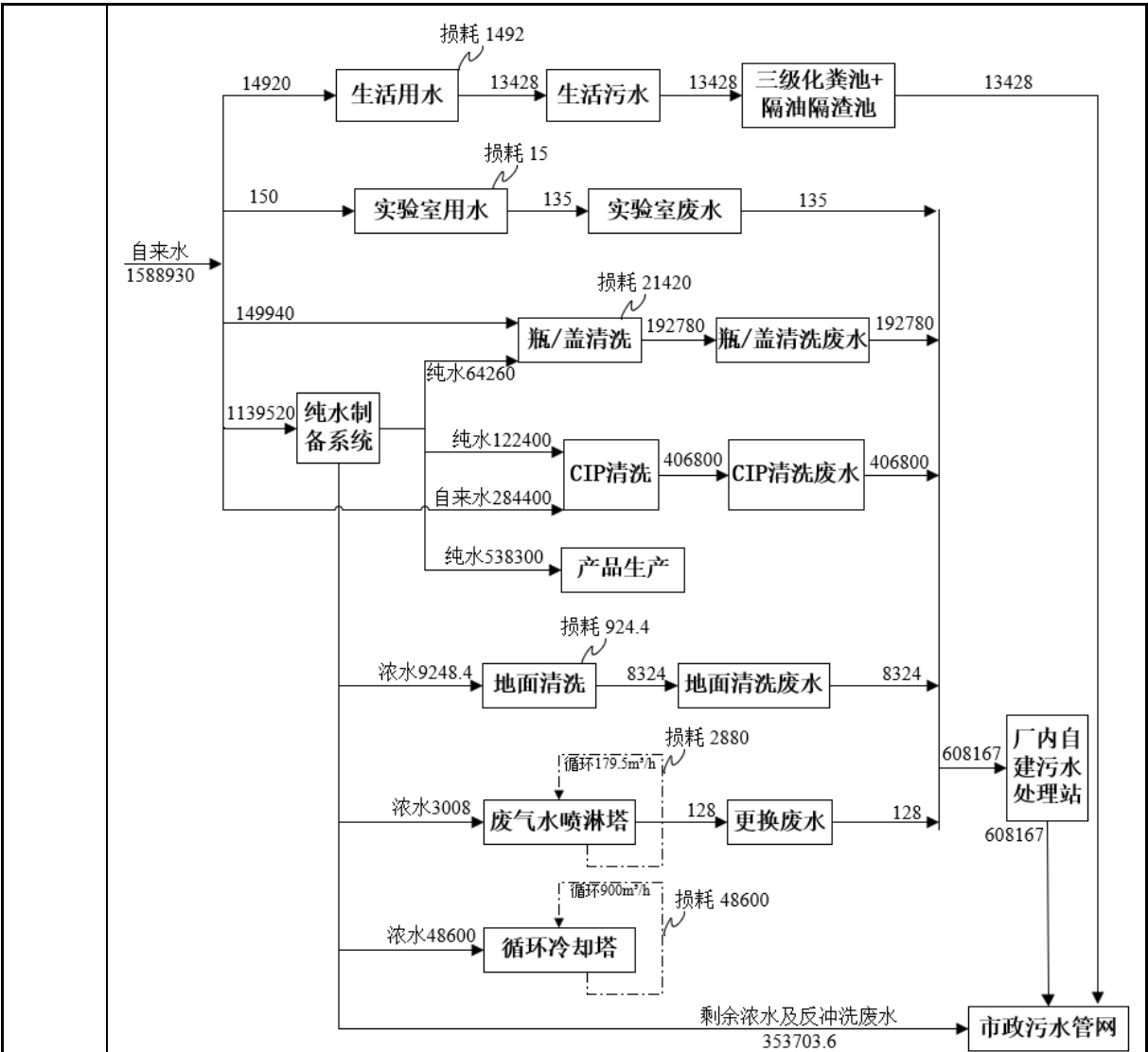
图 2-2 改扩建后全厂的水平衡图（单位： \text{m}^3/\text{a} ）
