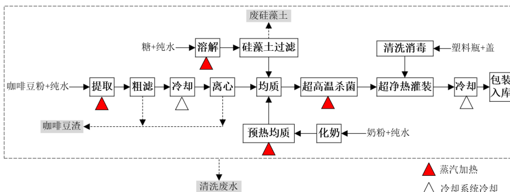
图 2-12 咖啡饮料的生产工艺流程及产污环节图（已停产）
