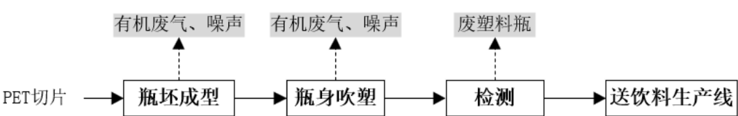
图 2-9 现有项目制瓶工艺流程及产污环节图
