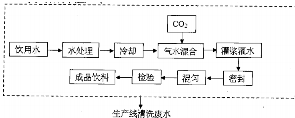
图 2-6 现有项目纯净水/苏打水的生产工艺流程及产污环节图
