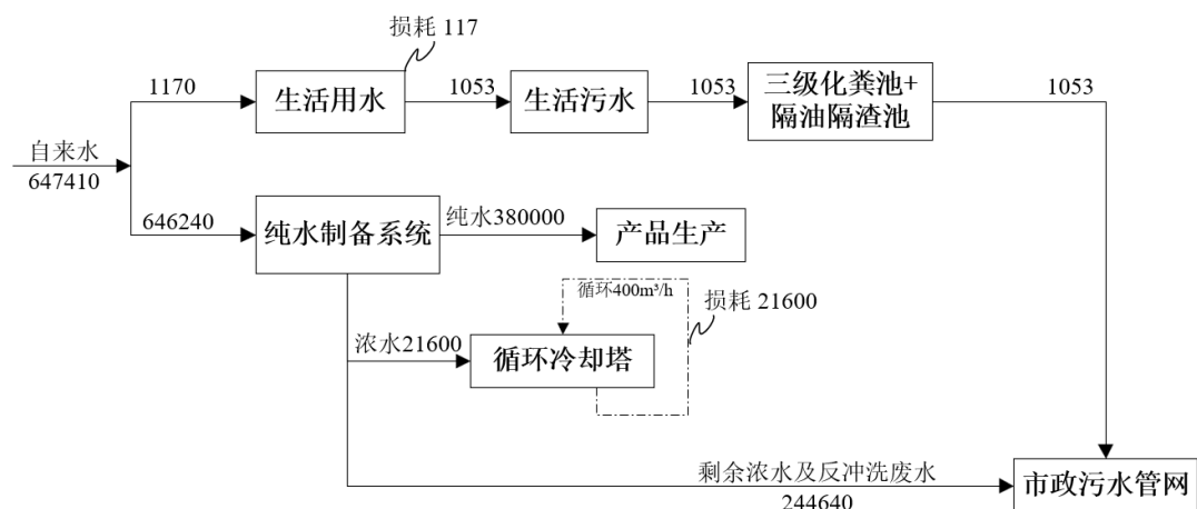
图 2-1 改扩建项目水平衡图（单位： \text{m}^3/\text{a} ）
