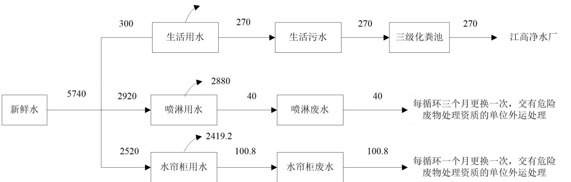
图1 本项目水平衡图 (t/a)
