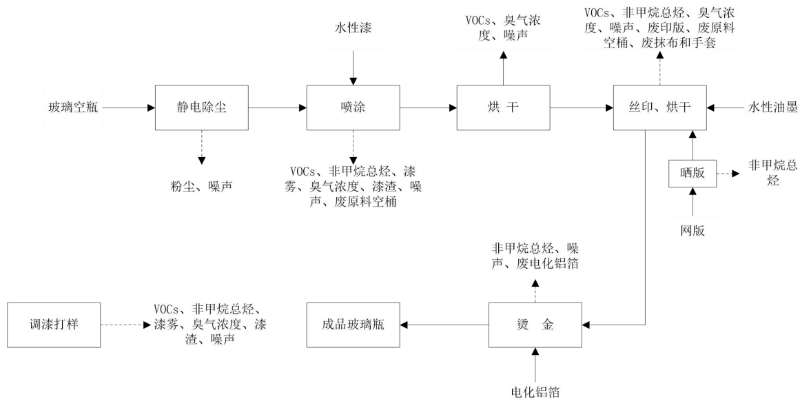
图2 本项目成品玻璃瓶加工生产工艺流程及产污环节图
