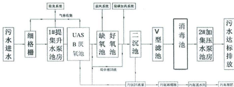
图 4-3 一、二期污水处理工艺流程图
