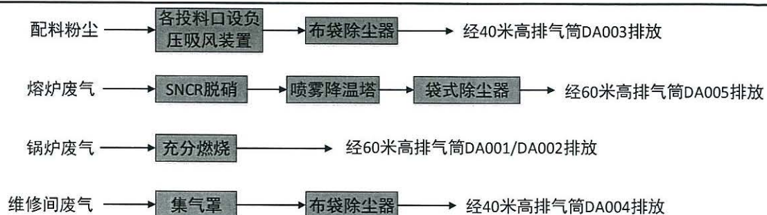
图2-5 现有项目废气处理工艺流程图
