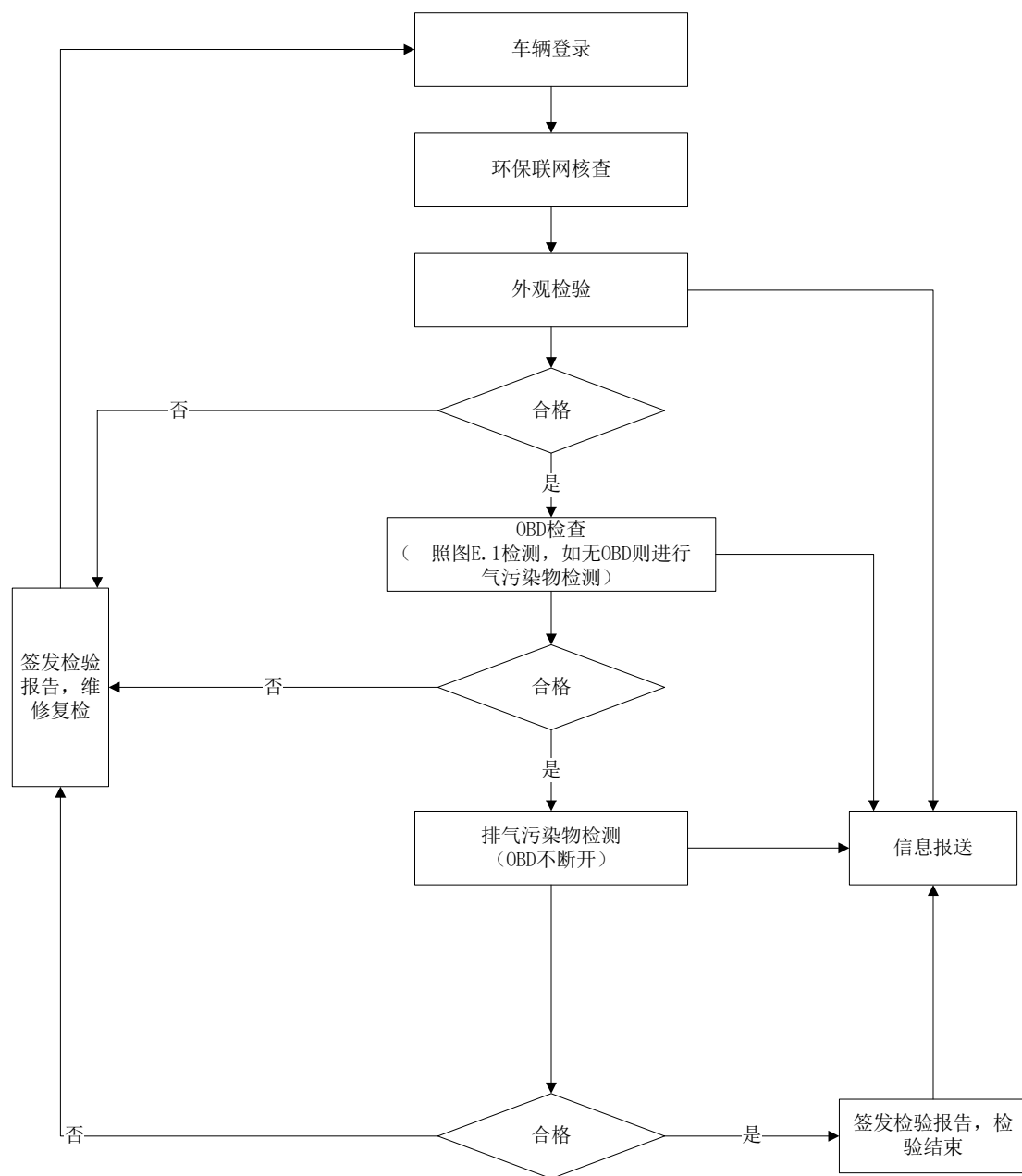
图 3 在用汽车环保检验流程图
