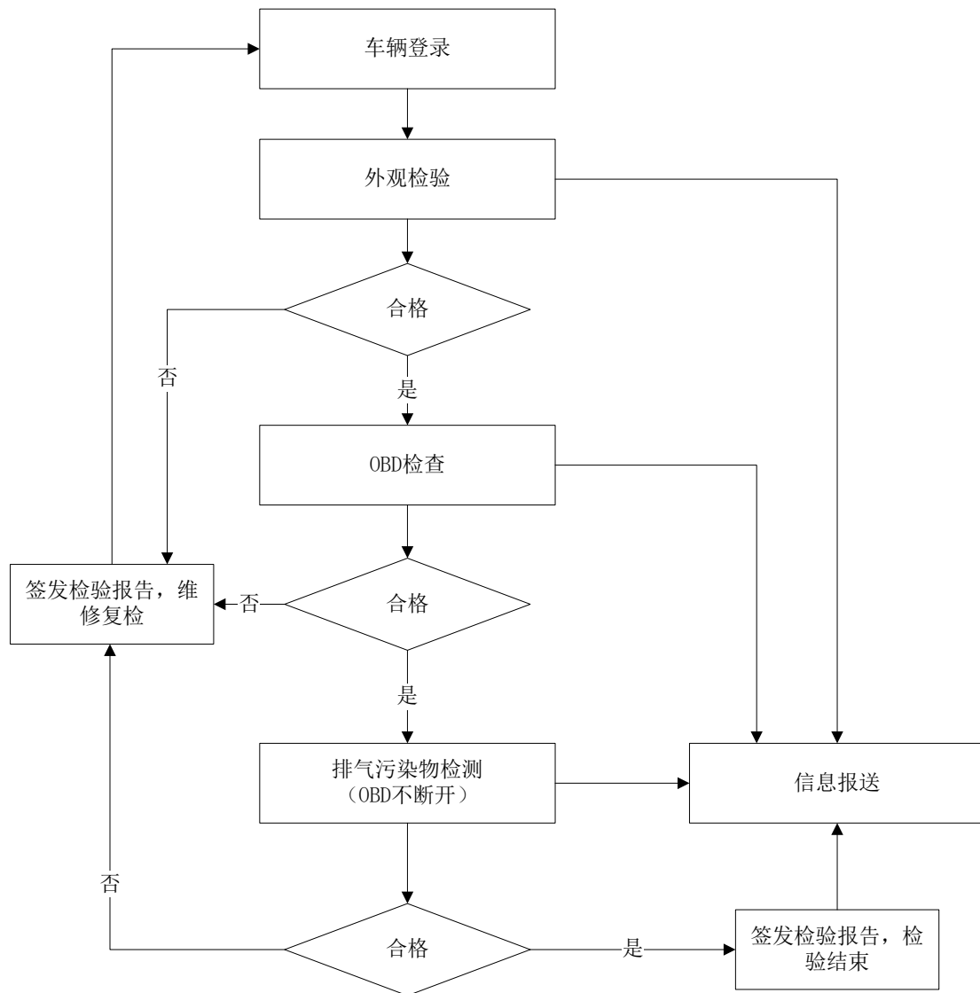
图 2 注册登记检验流程图
