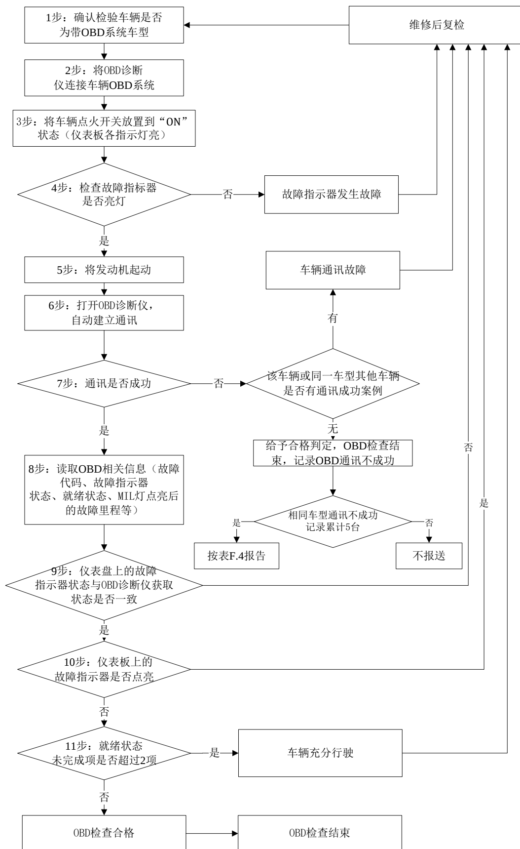
图 E.1 OBD 系统检查流程示意图
