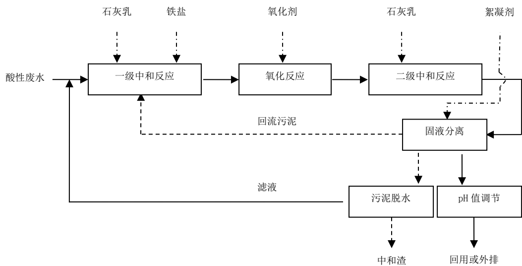
图 3 中和法处理酸性废水工艺流程图
