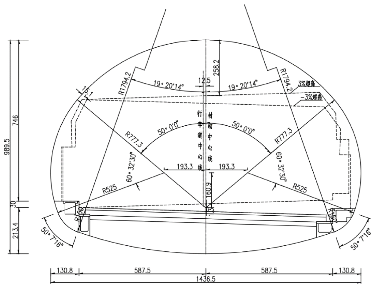
图 3.1-7 分离式隧道建筑限界及内轮廓图
