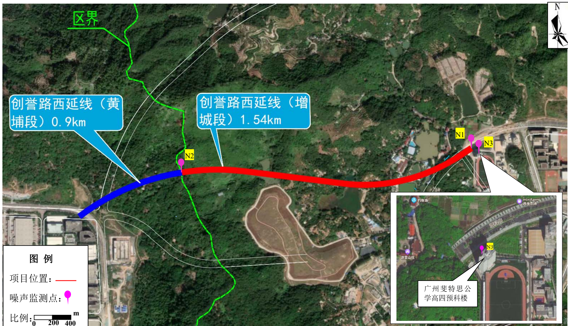
图 4.2-2 本项目噪声监测点位图
