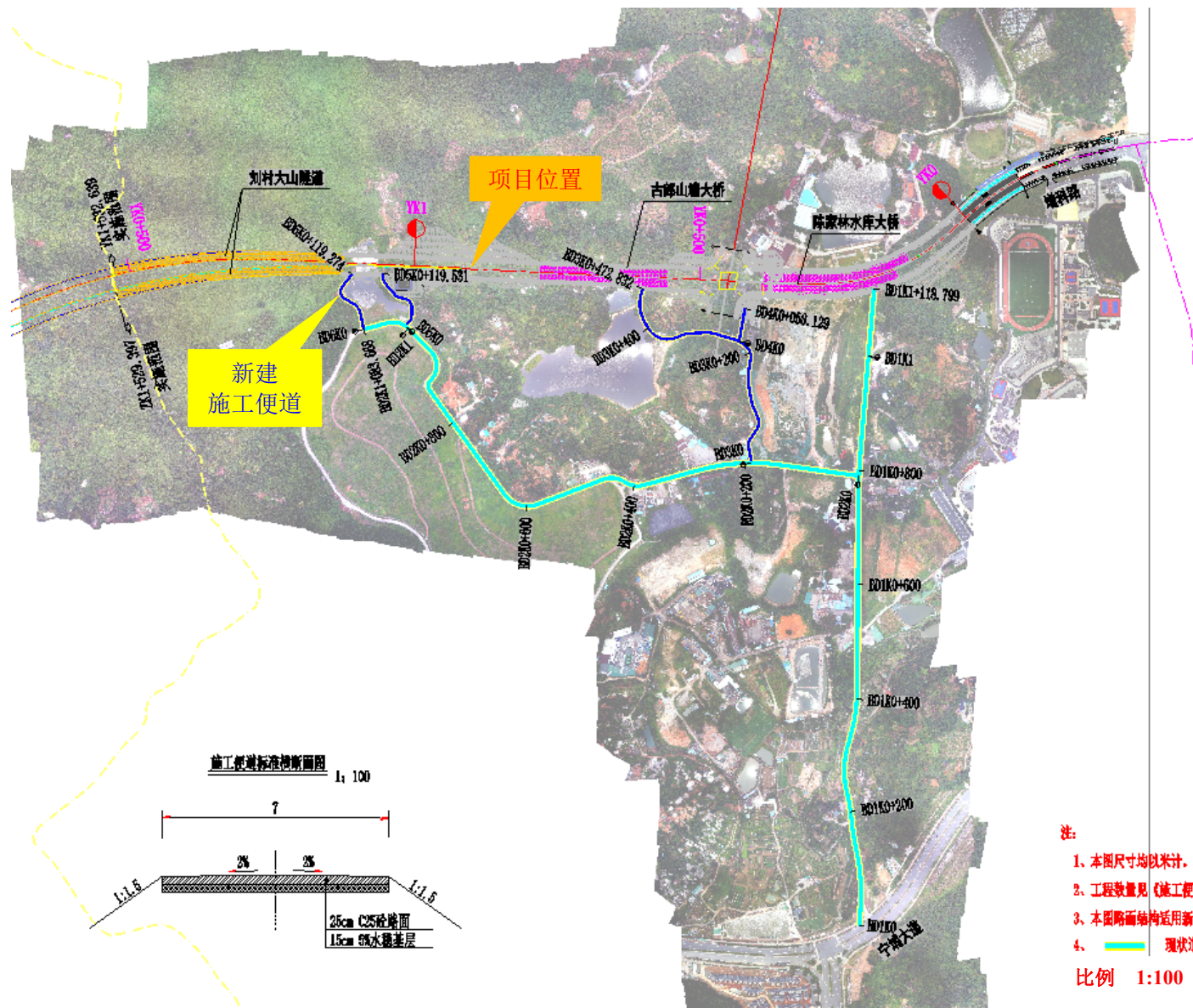
图 3.2-3 项目施工便道平面设计图
