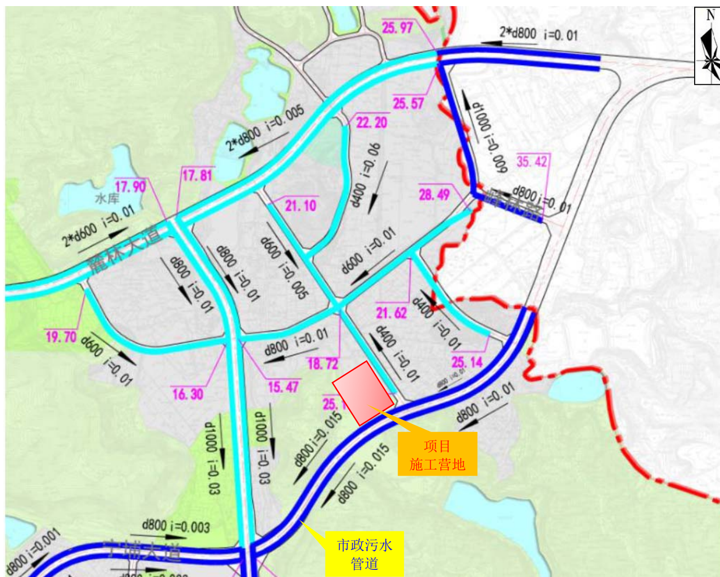
图 3.2-6 项目周边污水管网图
