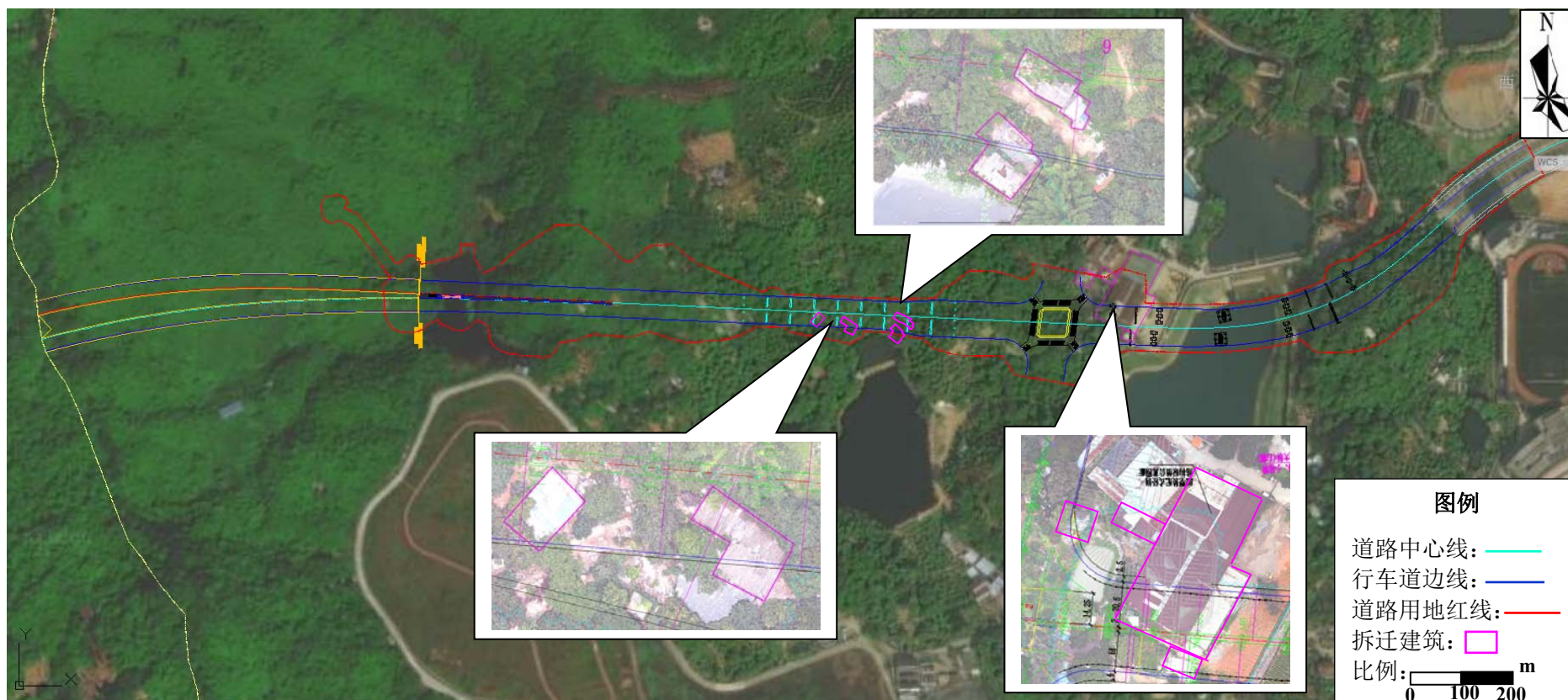
图 3.1-9 项目沿线建筑物拆迁范围图
