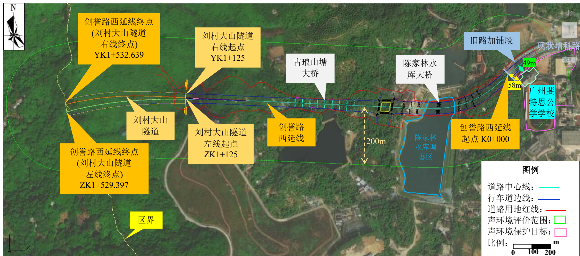
图 2.3-1 项目声环境评价范围及声环境保护目标分布图
