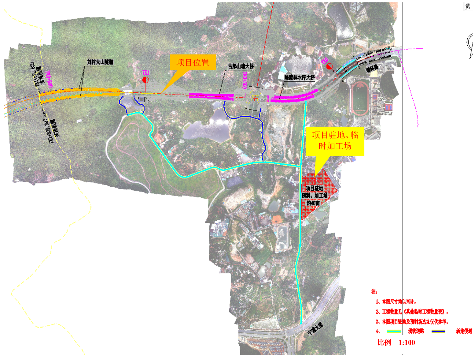
图 3.2-4 项目驻地（施工营地）、临时加工场（临时工程）布置图
