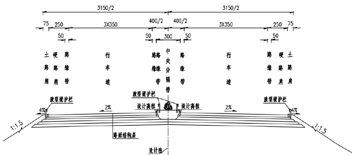
图 3.1-3 YK0+449.798~YK0+920 段整体式路基横断面图
