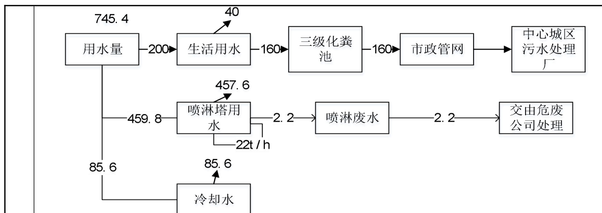
图 2-1 水平衡图 (单位: \text{m}^3/\text{a} )
