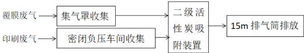
图 4-2 废气处理工艺图
