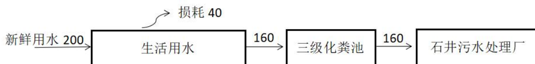
图 2-1 本项目水平衡图 (t/a)
