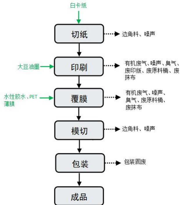
图 2-2 彩盒生产工艺流程及产污环节图
