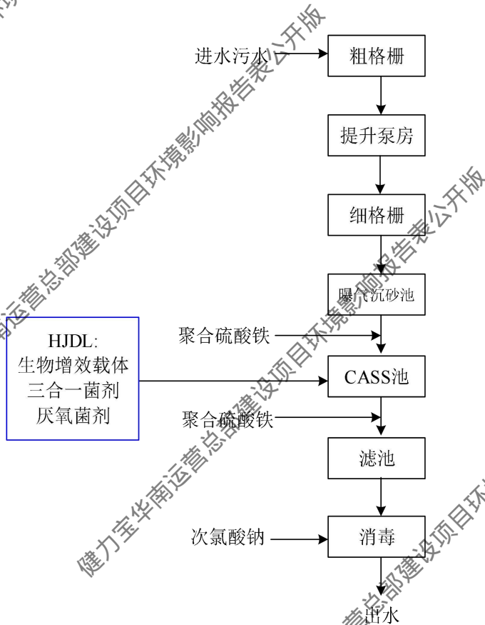
图 4.2-2 中部净水厂（一期）工艺流程图
