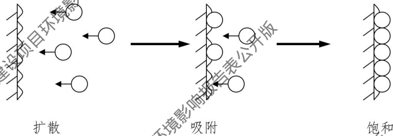
图 4.1-1 活性炭吸附过程示意图
