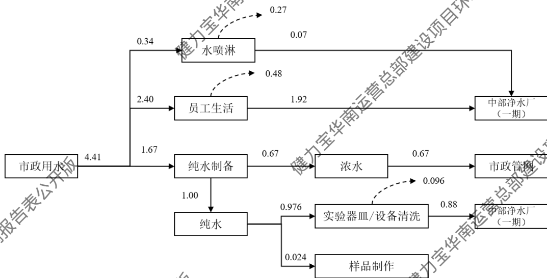
图 2.3-1 项目水平衡图 (单位: \text{m}^3/\text{d} )
