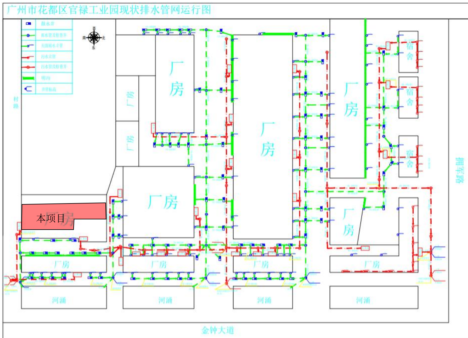
附图 20 雨污管网图
