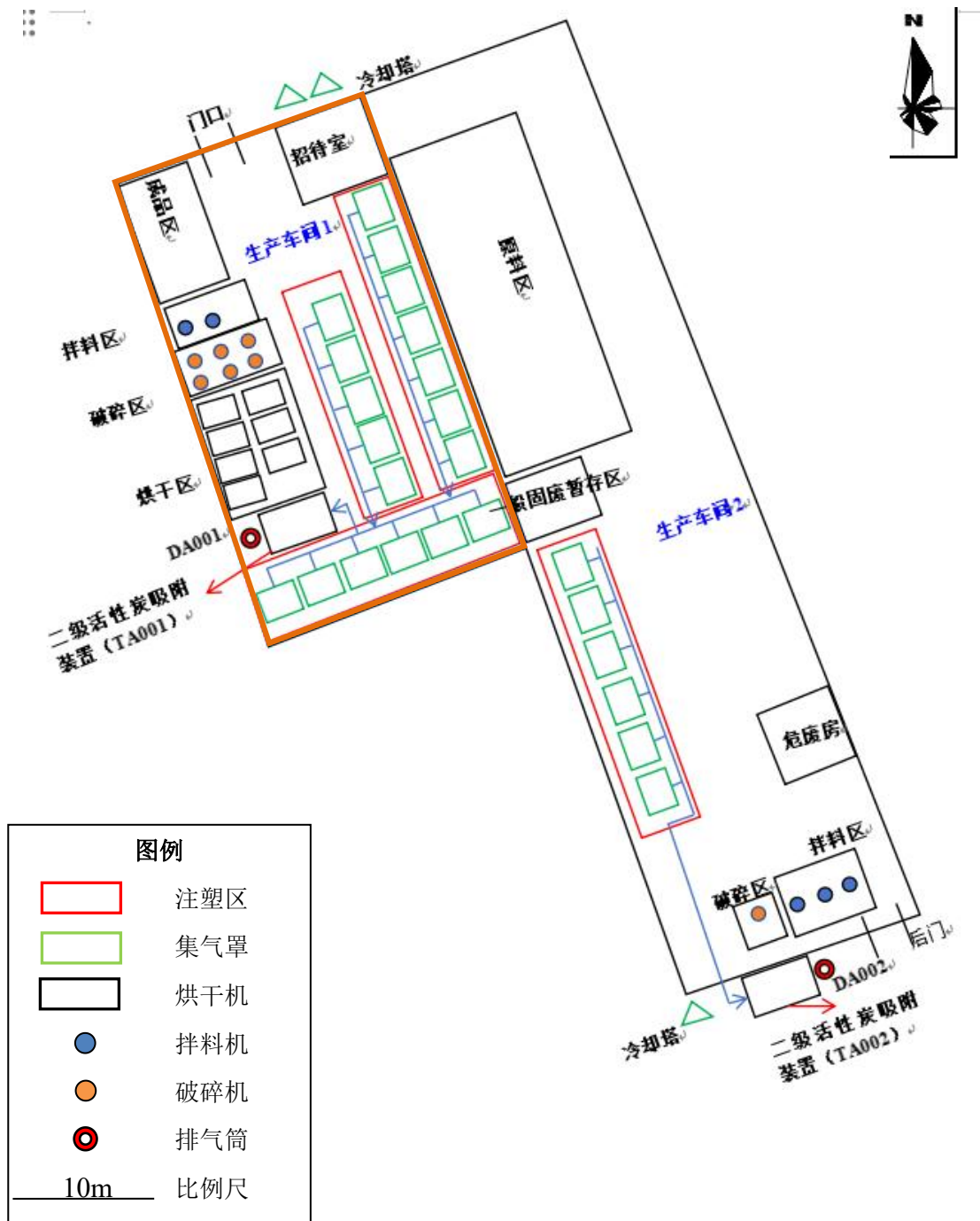
附图 4 项目总平面布置图
