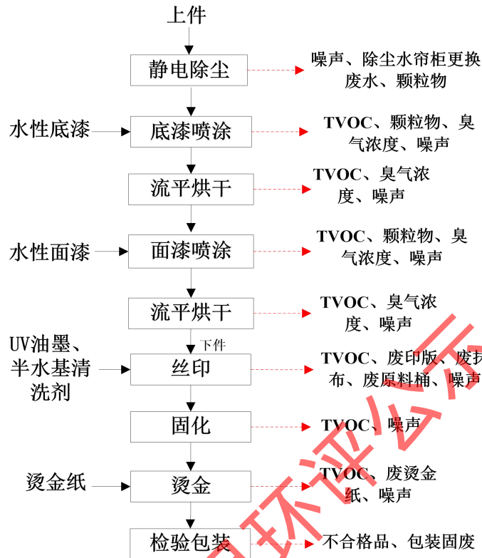
图 2-3 产品生产工艺流程及产污节点图
