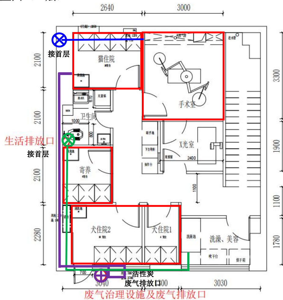
附图 3.2 项目平面布置图（二层）
