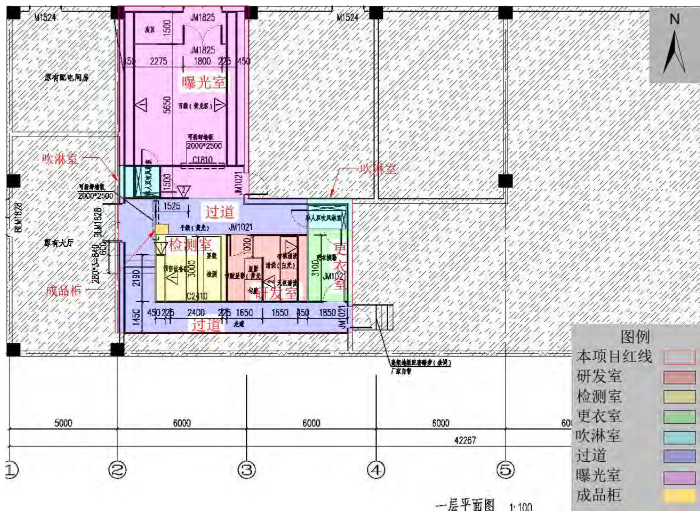
附图 5 本项目 16 栋一楼平面布置图
