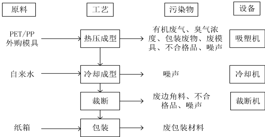
图 2-3 吸塑托盘工艺流程图
