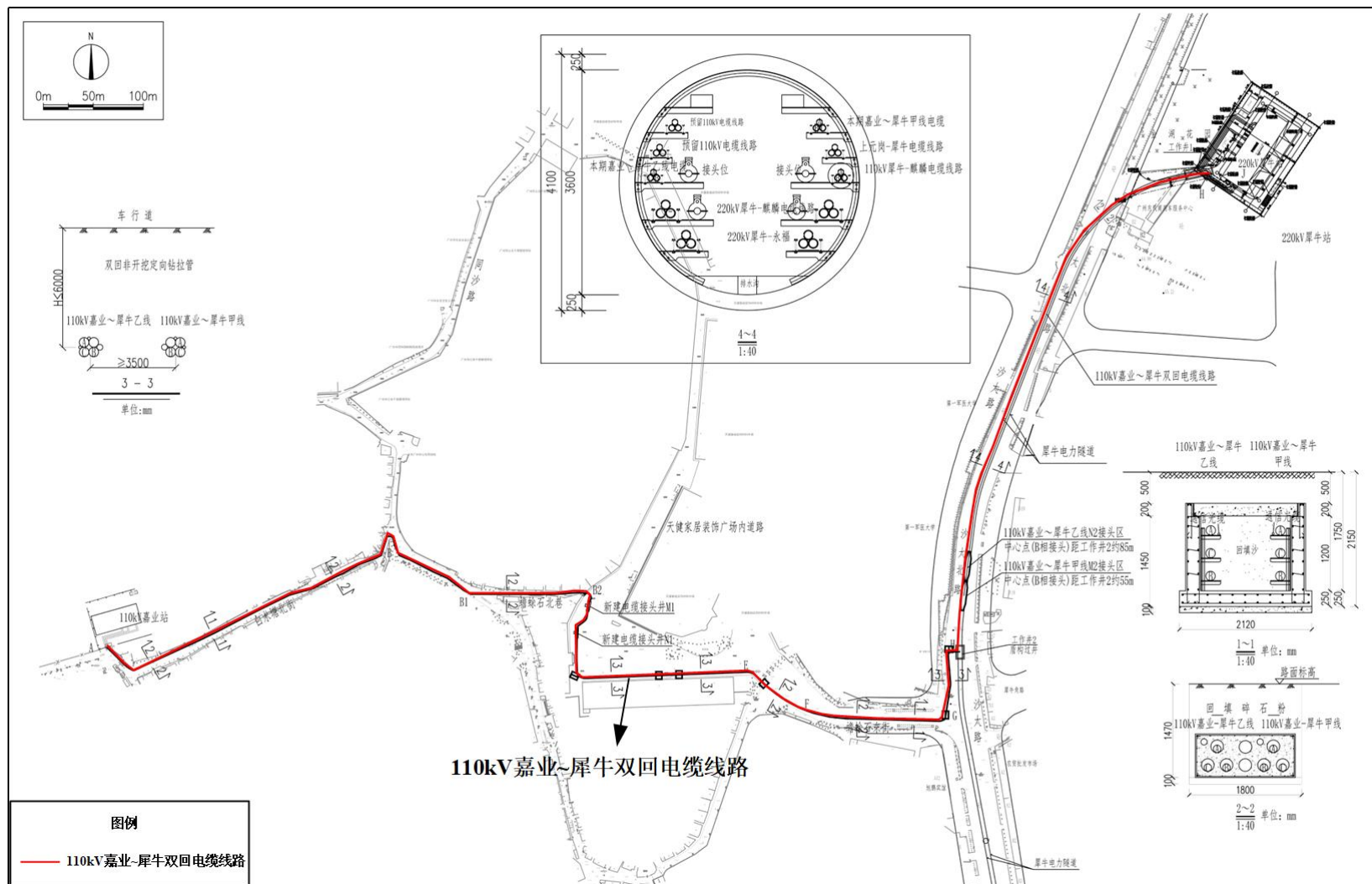
附图2 本项目线路路径图
