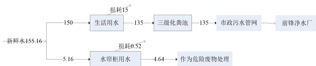
图2-1 项目水平衡图（单位：m³/a）
