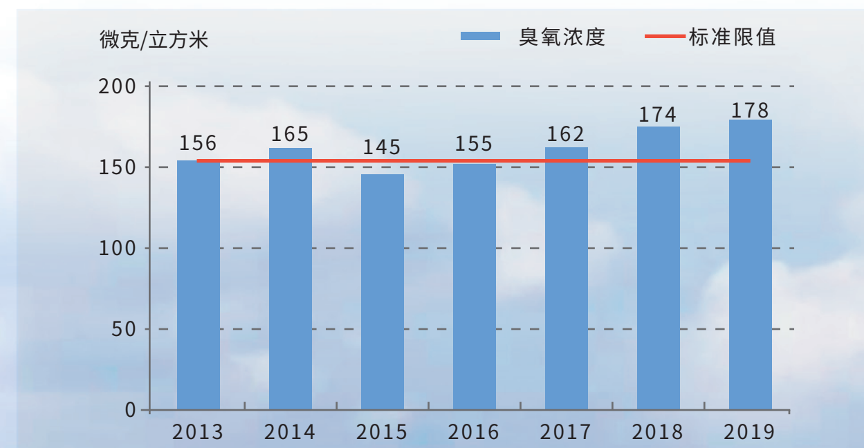
图6 2013-2019年臭氧浓度
