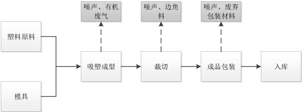
图 2-5 项目吸塑生产工艺流程及产污环节
