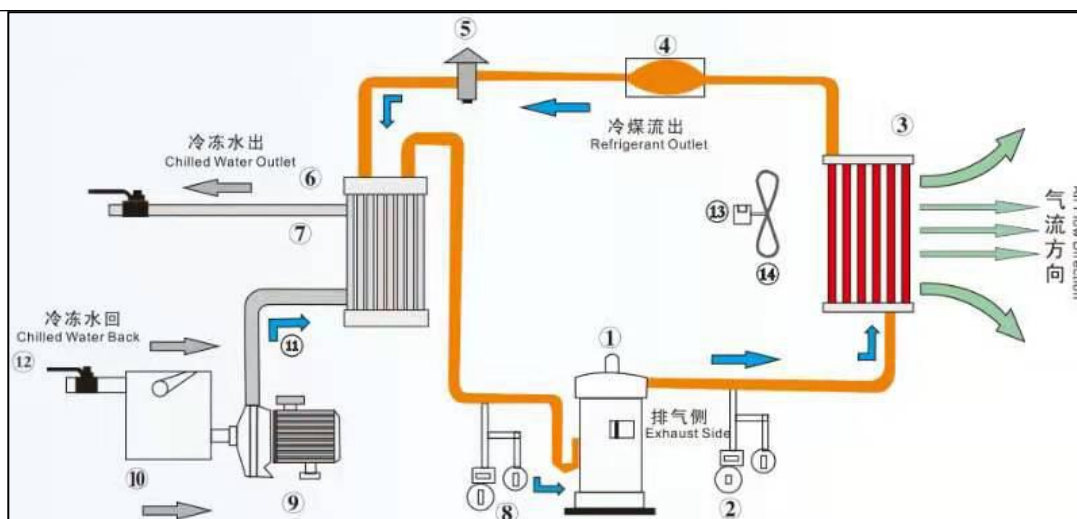
图 2-6 风冷式冷水机组工作原理图
