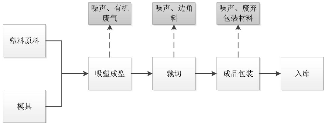
图 2-9 原项目吸塑生产工艺流程及产污环节
