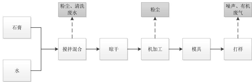
图 2-8 原项目石膏模具生产工艺流程及产污环节
