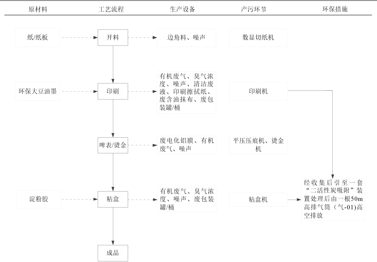
图2-3 迁扩建前项目商品零售包装盒生产工艺流程图
