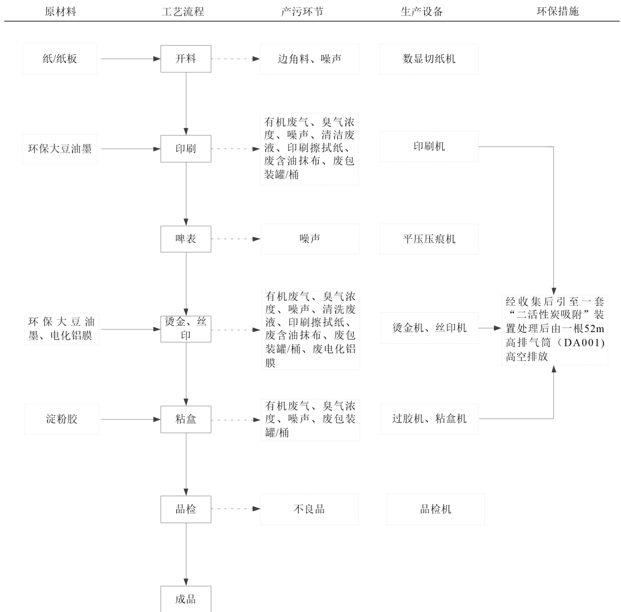
图 2-2 本迁扩建项目工艺流程图
