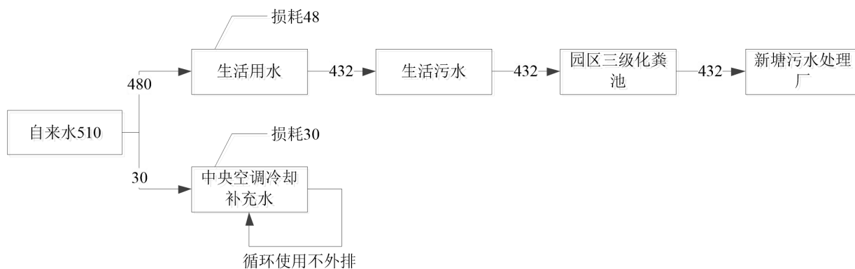
图 2-2 迁扩建前项目水平衡图 (单位 m³/a)
