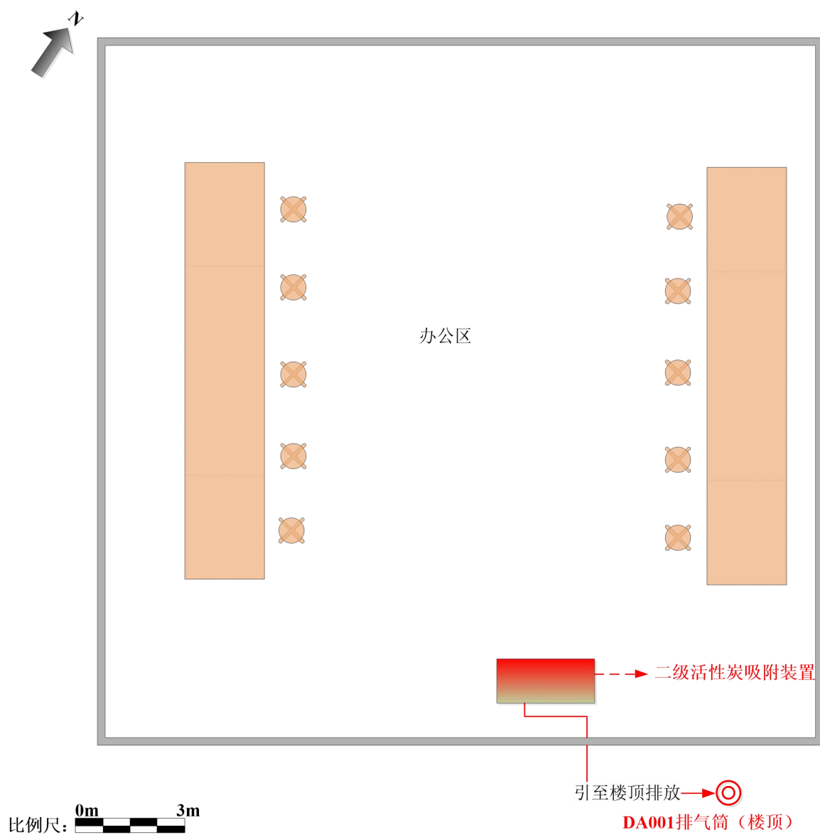
附图 4-2 项目平面布置图 (本迁扩建项目 1 楼夹层)
