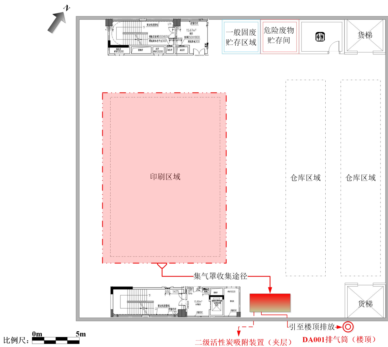
附图 4-1 项目平面布置图 (本迁扩建项目 1 楼)
