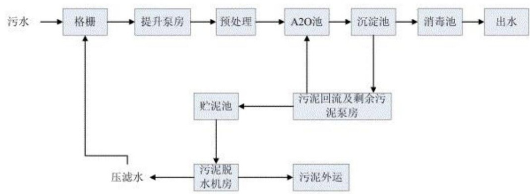
图 4-1 大岗南部污水处理厂处理工艺流程图
