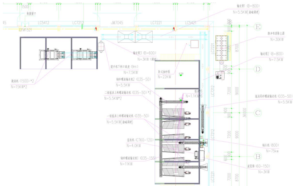
图 2-2 设备连接示意图
