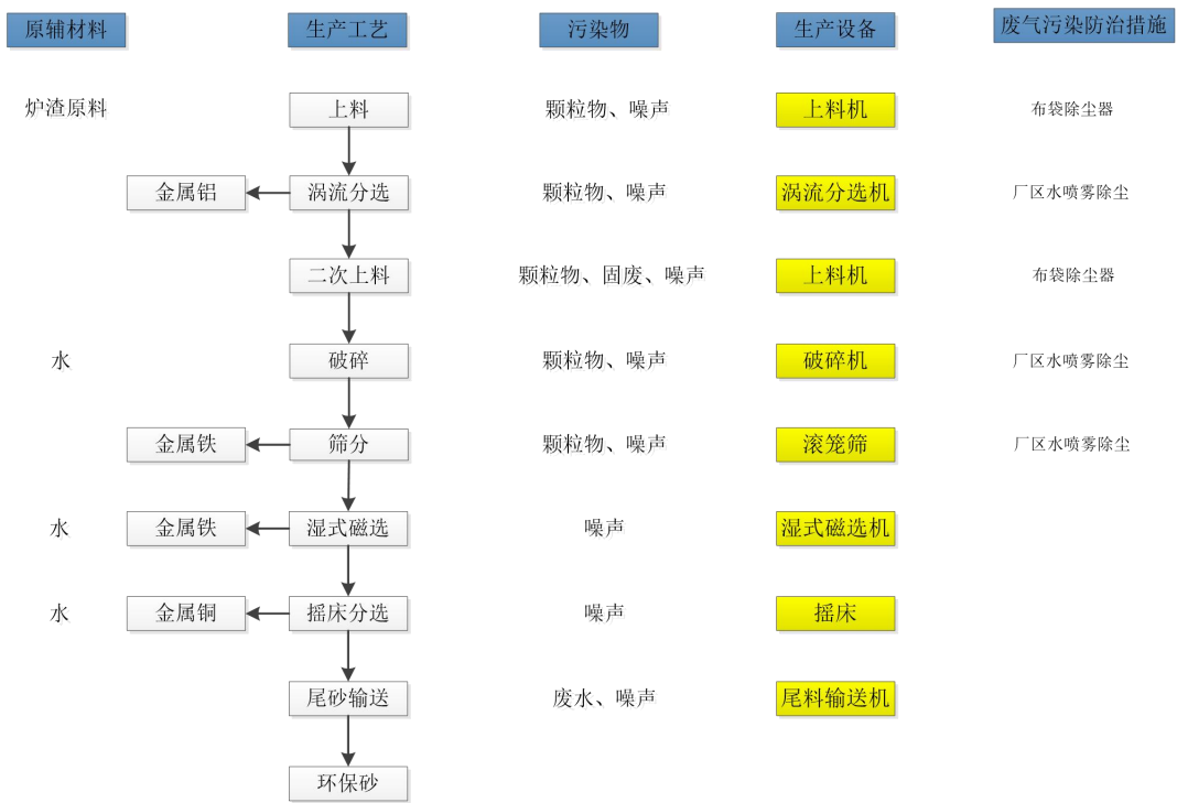
图 2-1 本项目炉渣处理工艺流程及产污环节示意图
