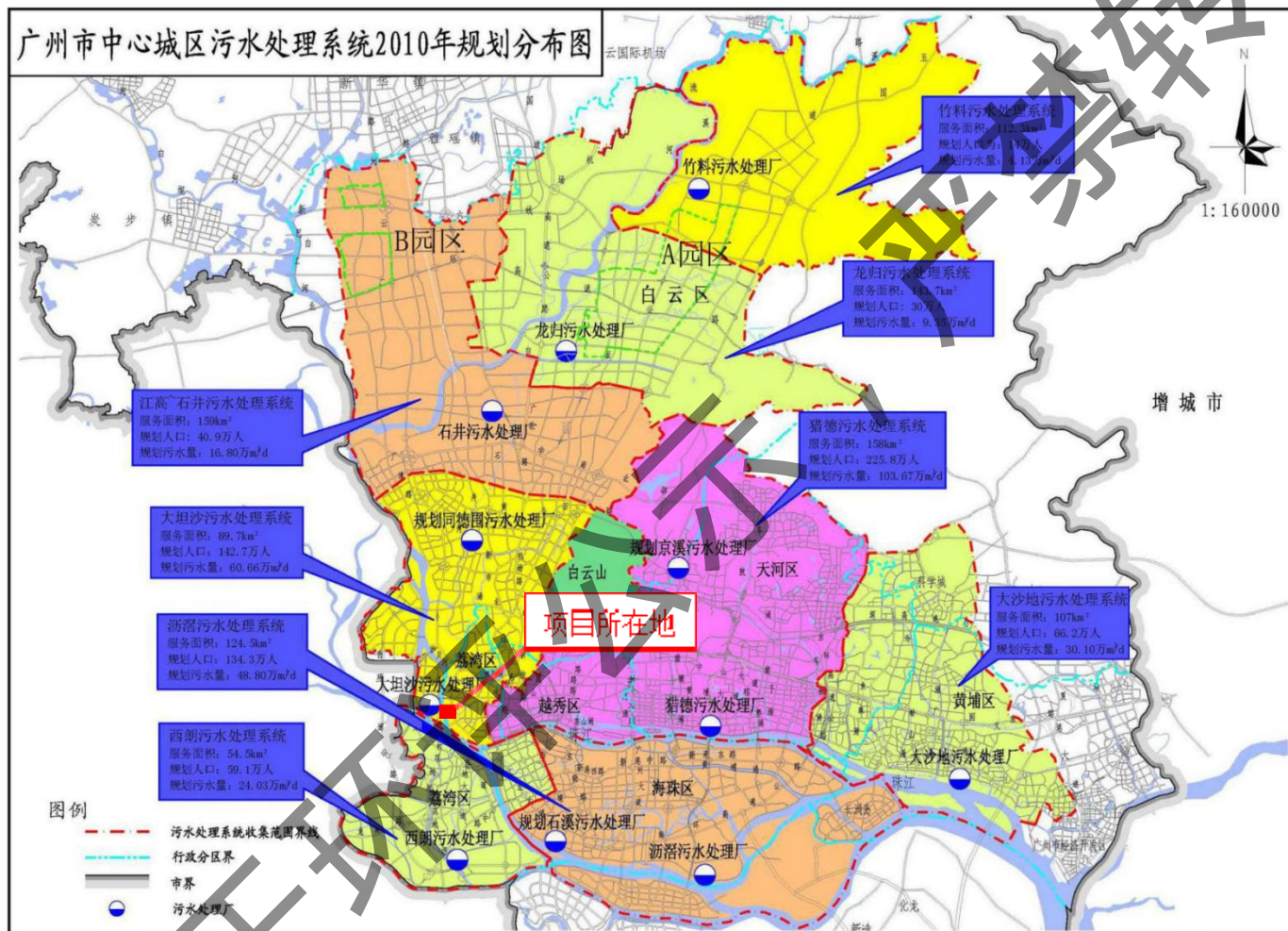
附图 14 广州市中心城区污水处理系统分布图
