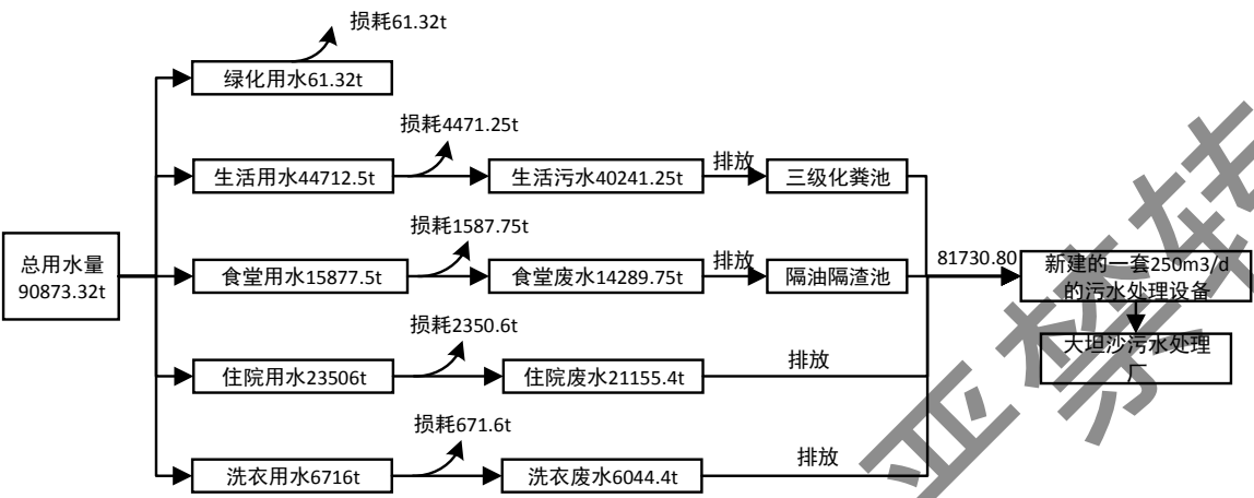
图 4-1 本扩建项目水平衡图
