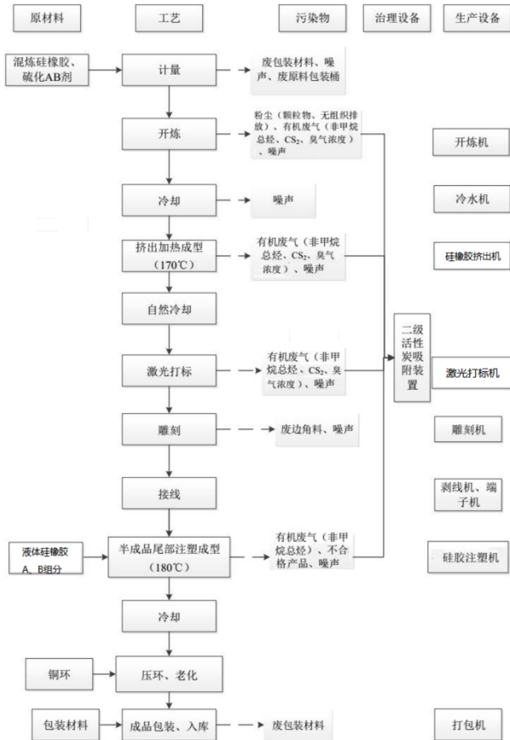
(3) 硅橡胶霓虹灯带生产工艺及产污环节流程见下图:
