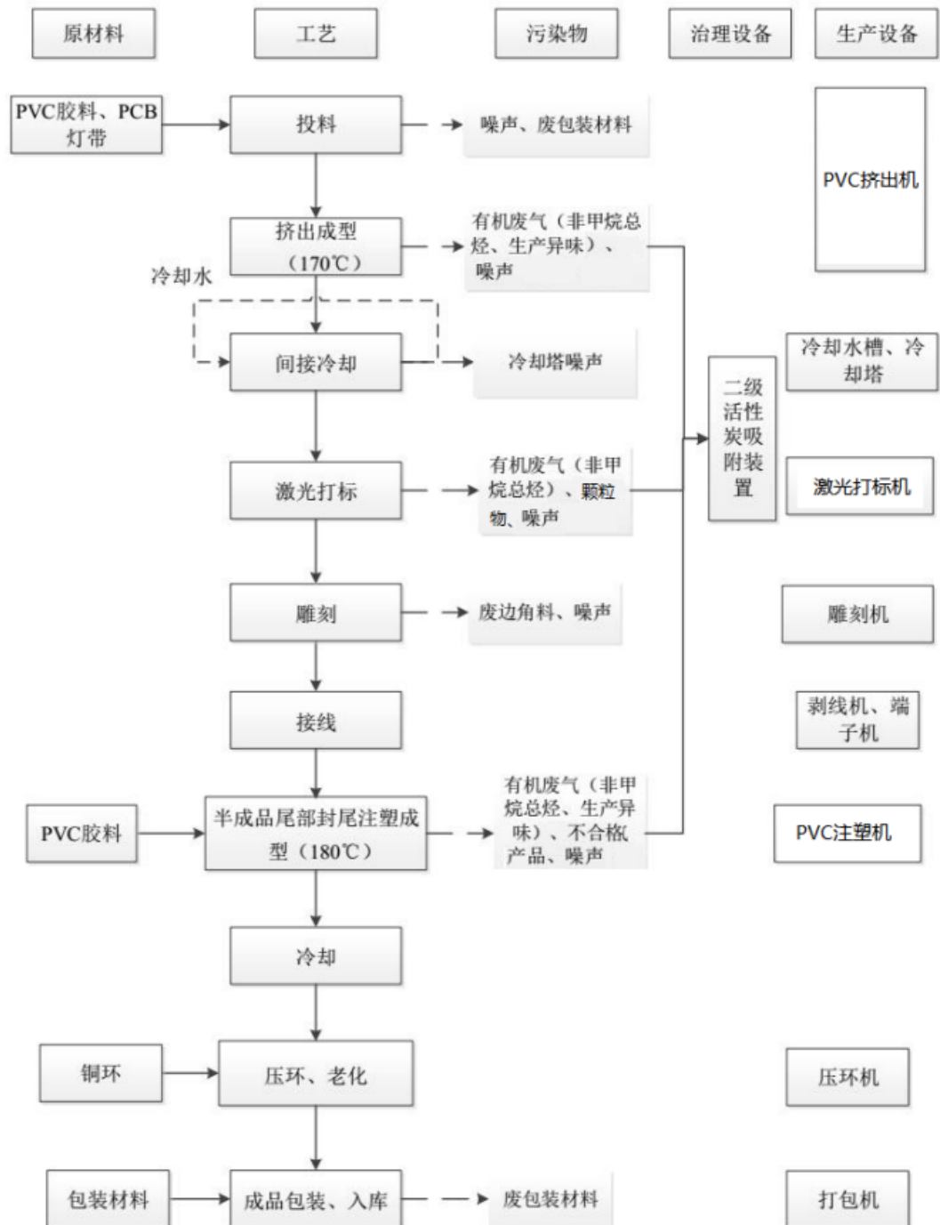
图 2-6 PVC 霓虹灯带生产工艺流程及产污环节图
