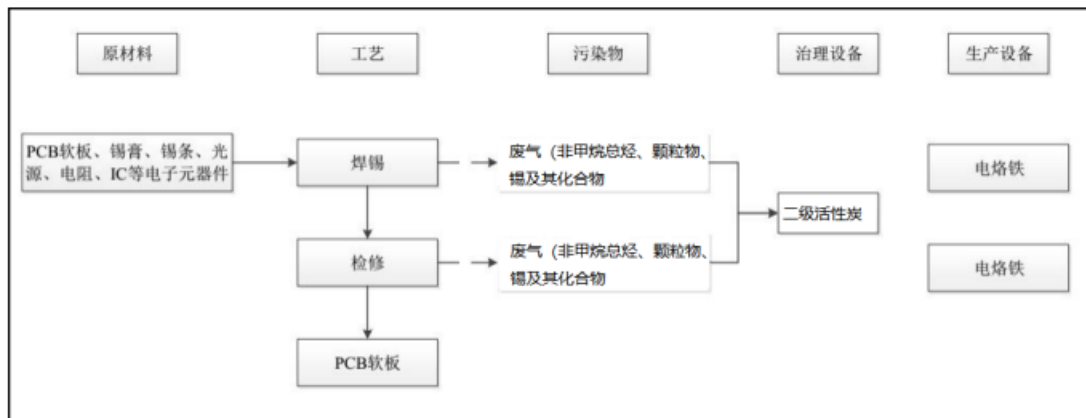
图 2-5 PCB 软板生产工艺流程及产污环节图
