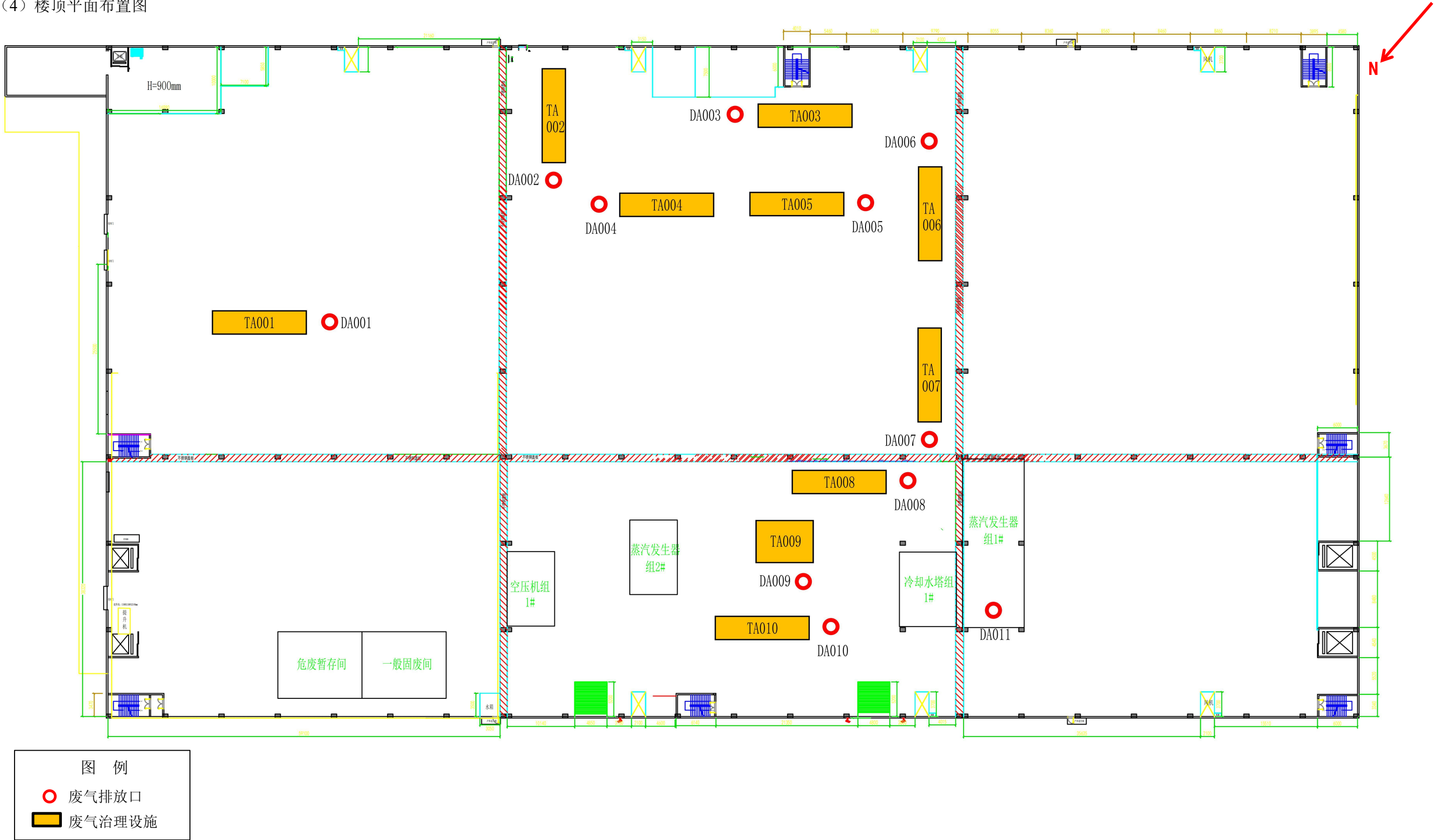
(4) 楼顶平面布置图
