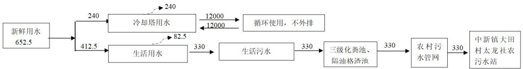
图2-3 改扩建后项目用水平衡示意图 (单位: m³/a)
