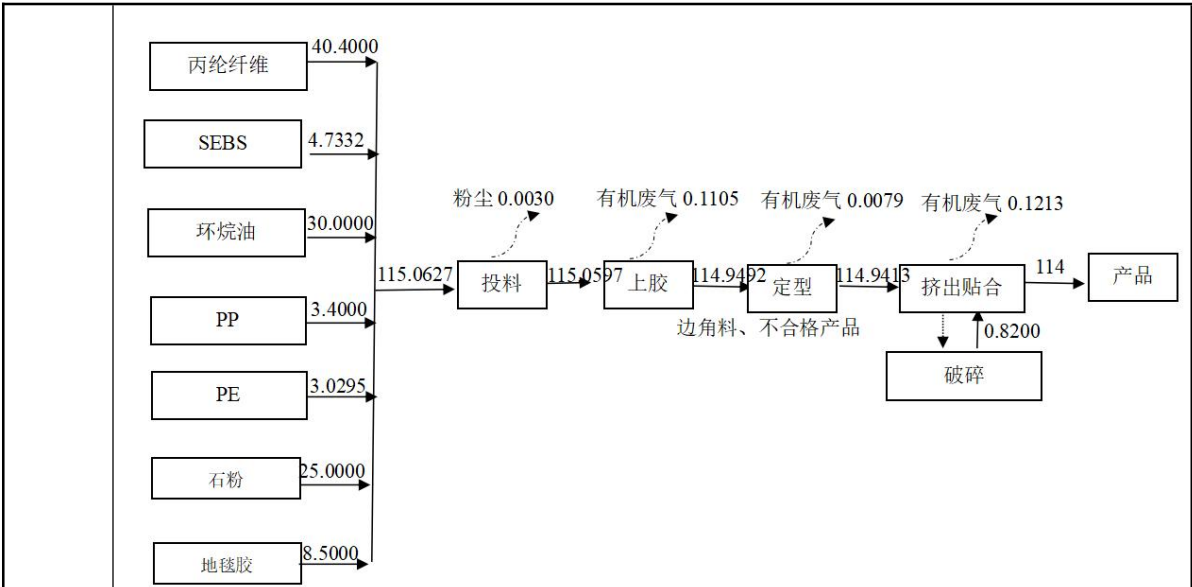
图2-1b 改扩建项目TPR地毯物料平衡示意图 (单位: t/a)
