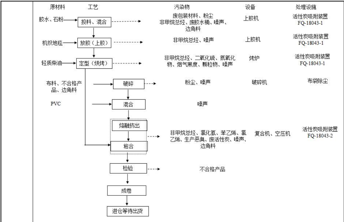
图2-6 改扩建项目PVC地毯工艺流程图
