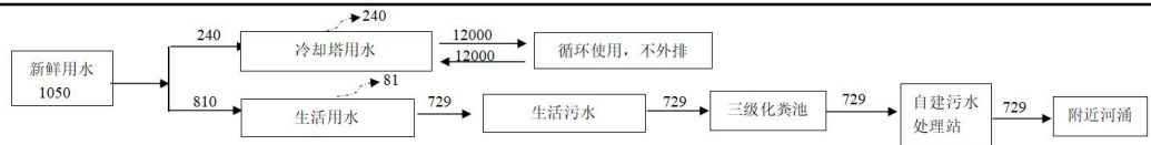
图2-2 原项目用水平衡示意图 (单位: m³/a)
