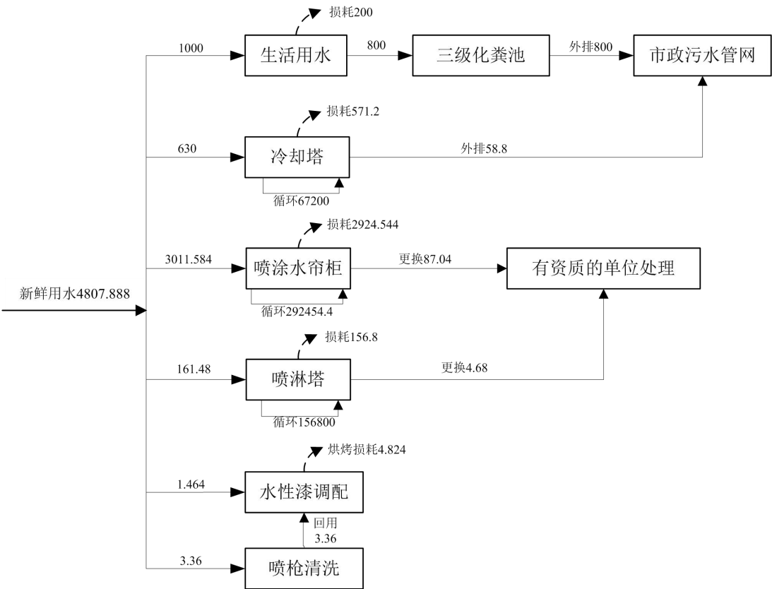
图 4-2 项目年水平衡图 单位 m 3 /a
