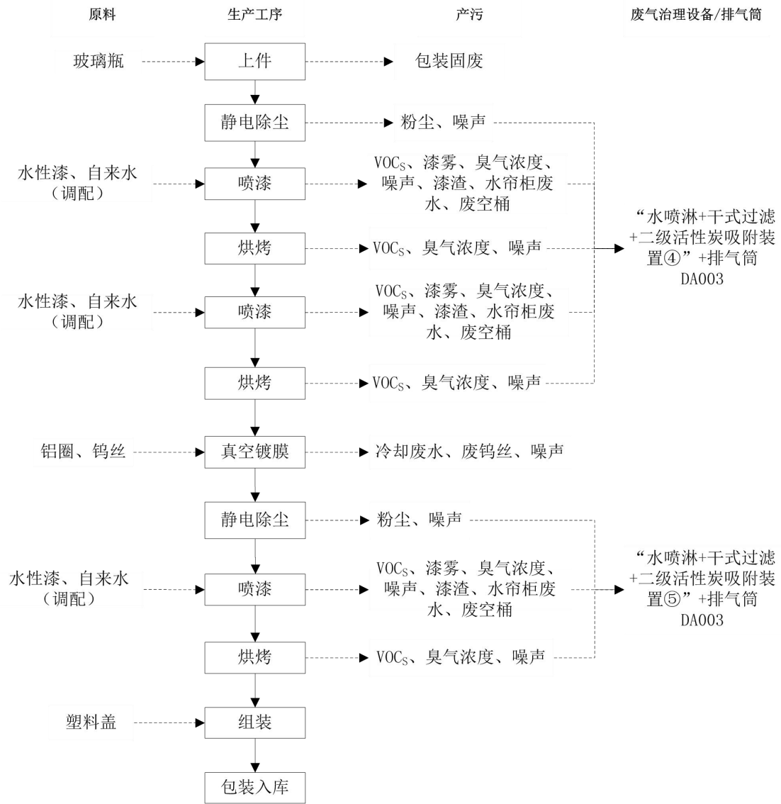
图2-3 玻璃瓶（含电镀工艺）生产工艺流程图
