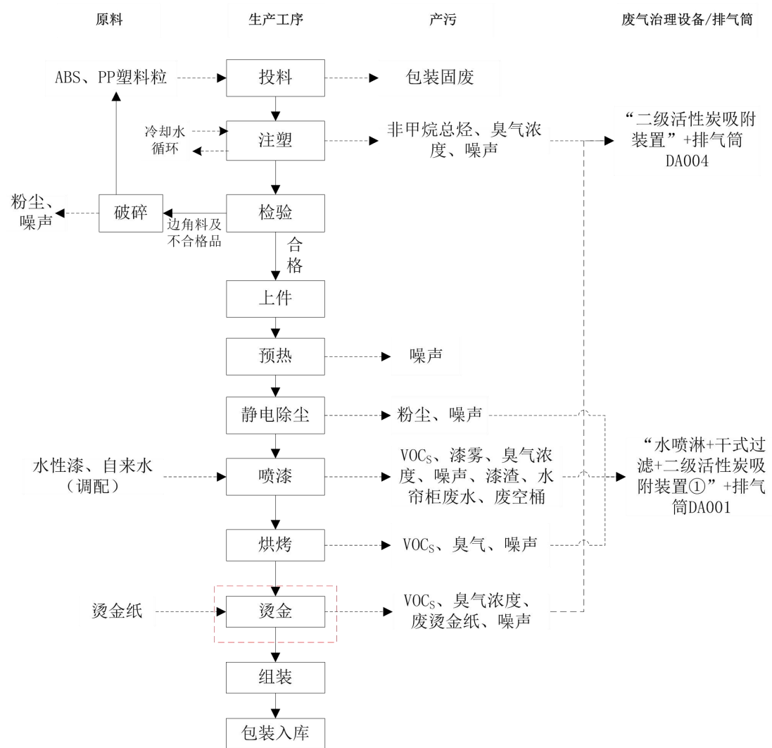
图2-1 塑料瓶、盖生产工艺流程图
